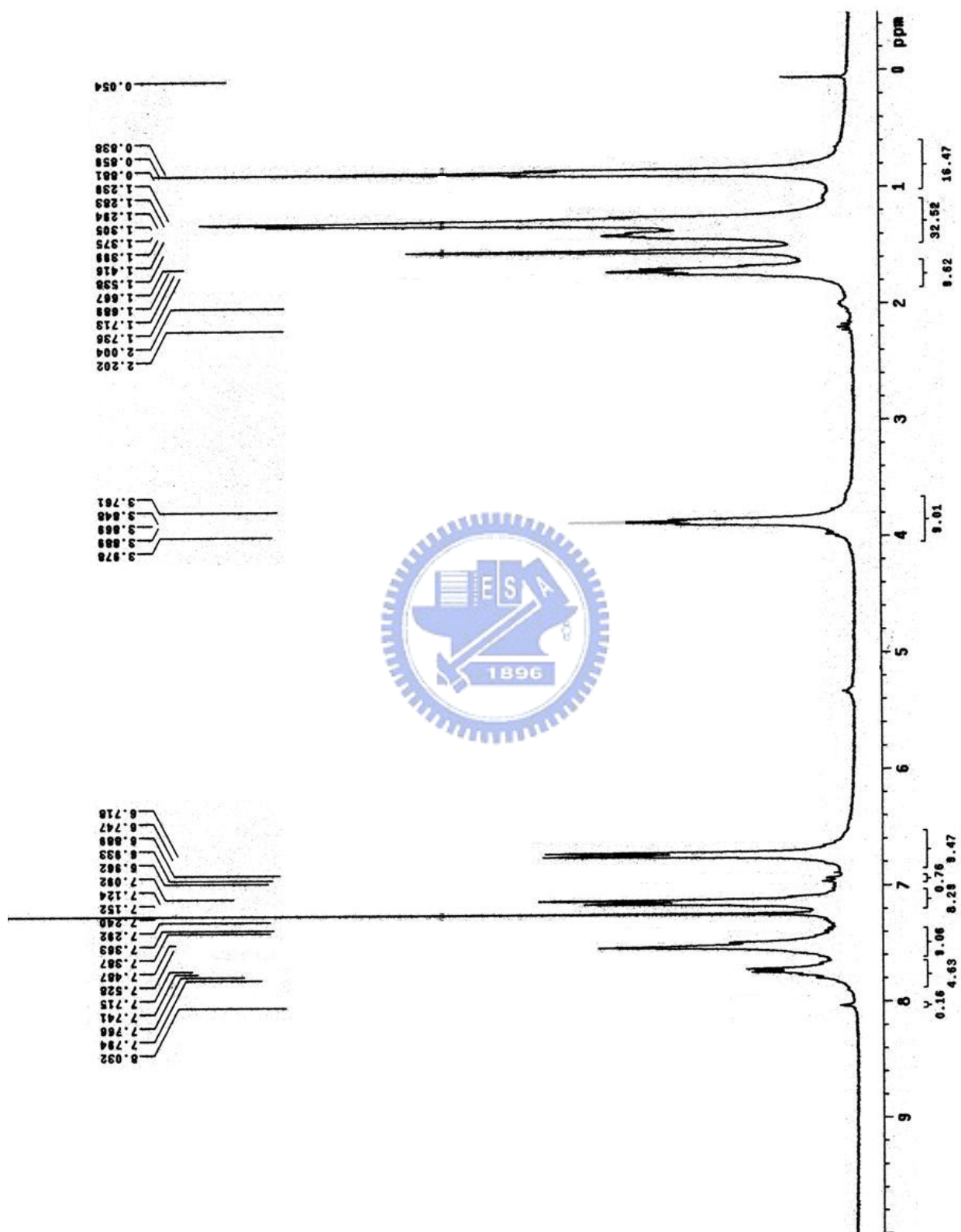
附圖 33. ^1\text{H} -NMR spectrum of P4-TAZ3-TPA0
