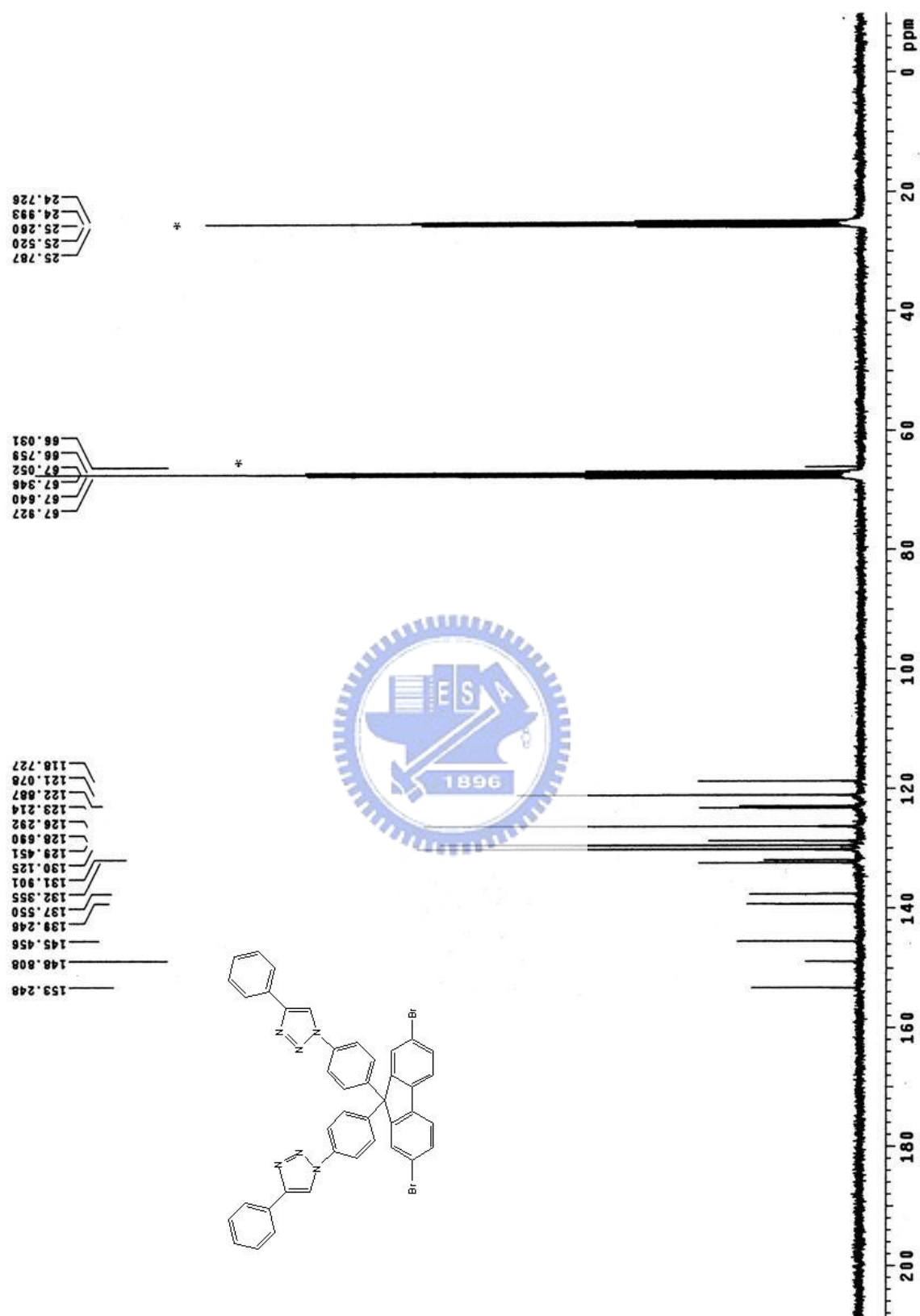
附圖 8. 13 C-NMR spectrum of M1
