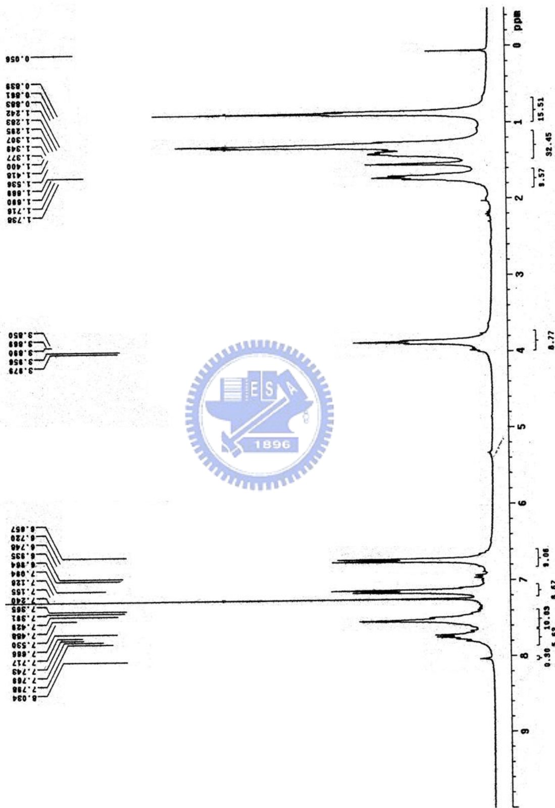
附圖 24. ^1\text{H} -NMR spectrum of P1-TAZ5
