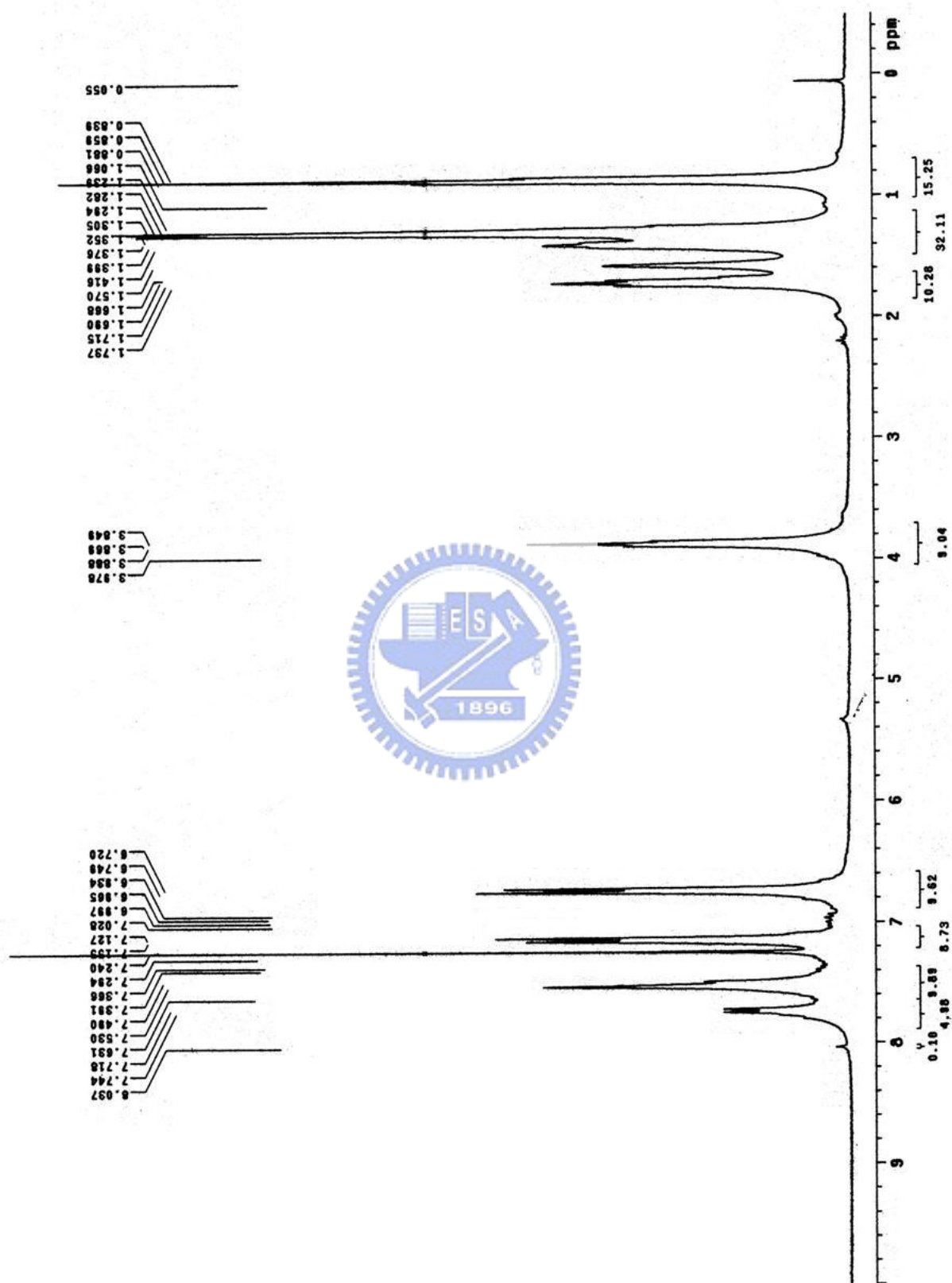
附圖 25. ^1\text{H} -NMR spectrum of P1-TAZ2
