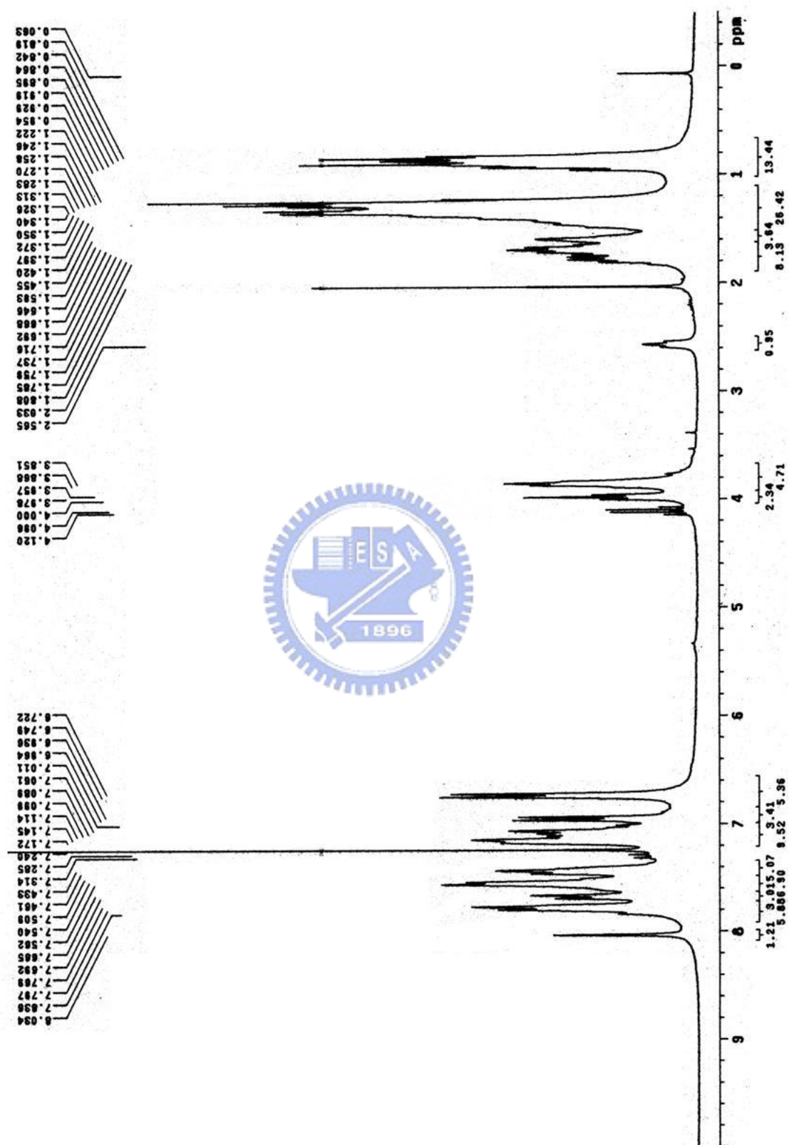
附圖 26. ^1\text{H} -NMR spectrum of P2-TAZ25
