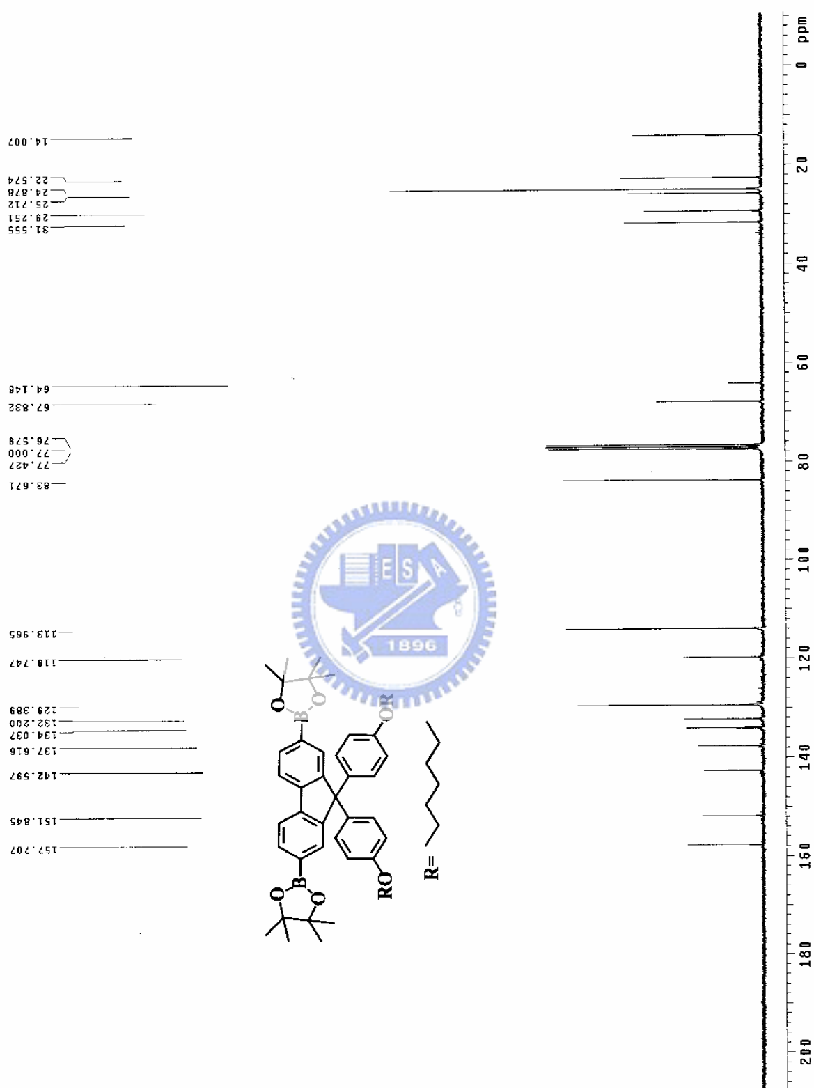
附圖 11. ^{13}\text{C} -NMR spectrum of M4
