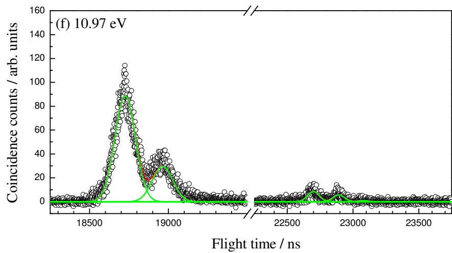
圖 3-5-2 激發光能量(d) 10.92 (e) 10.94 (f) 10.97 eV 之 1,3 二氯丙烷同現質譜。
