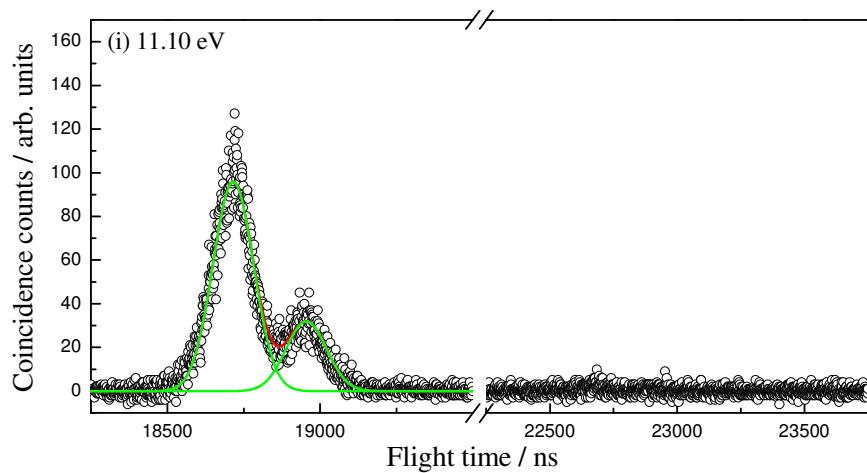
圖 3-5-3 激發光能量(g) 11.00 (h) 11.05 (i) 11.10 eV 之 1,3 二氯丙烷同現質譜。
