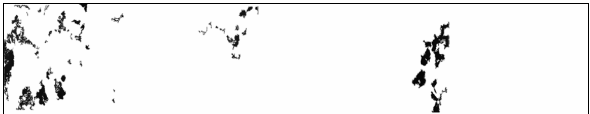
(d) 28 天齡期孔隙分佈圖(孔隙率=10.60%)
