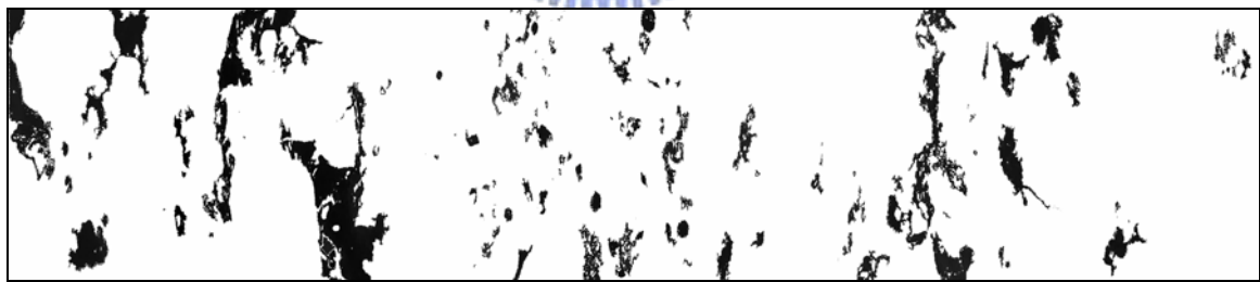
(d) 28 天齡期孔隙分佈圖(孔隙率=9.93%)
