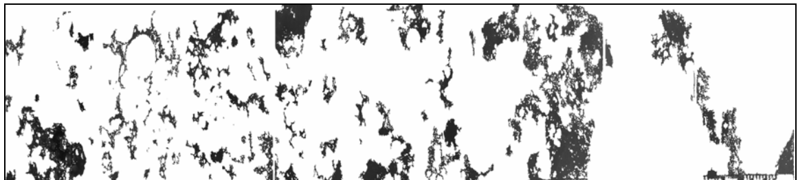
(c) 14 天齡期孔隙分佈圖(孔隙率=15.13%)
