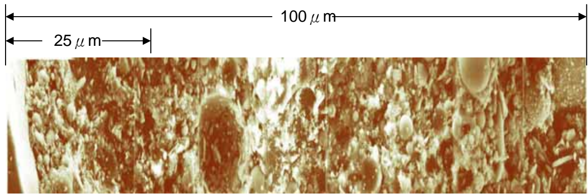
(a) 1 天齡期過渡區之微觀晶相圖 (W/B=0.35)
