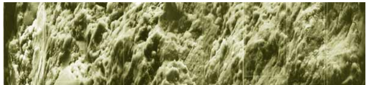
(e) 56 天齡期過渡區之微觀晶相圖 (W/B=0.54)
