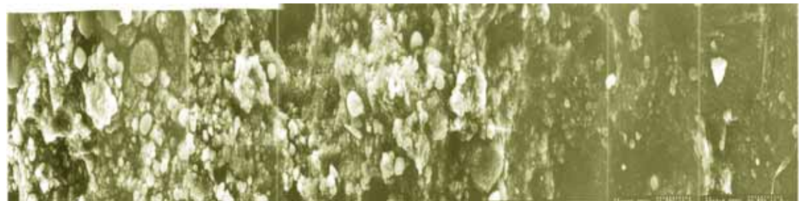
(c) 14 天齡期過渡區之微觀晶相圖 (W/B=0.54)
