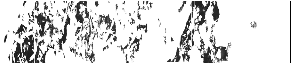
(b) 7 天齡期孔隙分佈圖(孔隙率=19.01%)
