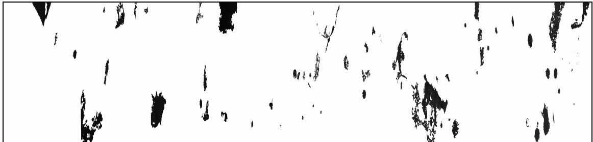
(e) 56 天齡期孔隙分佈圖 (孔隙率 5.11%)
