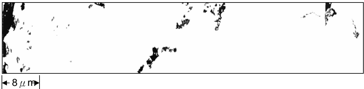
(e) 56 天齡期孔隙分佈圖(孔隙率=3.51%)
