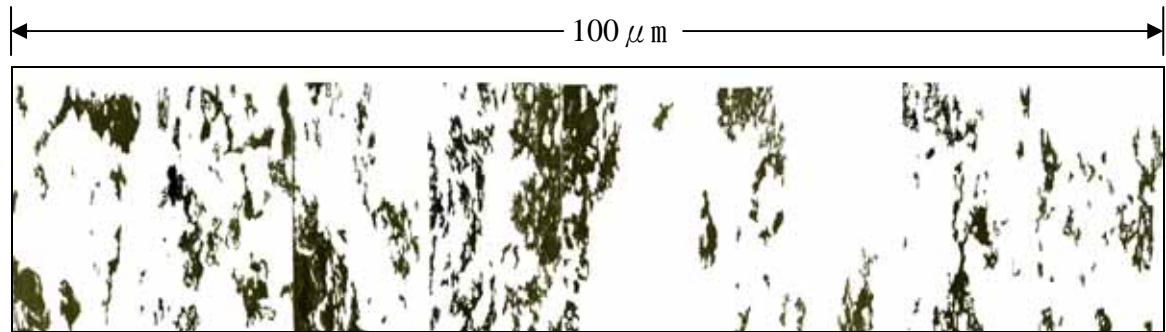
(a) 1 天齡期孔隙分佈圖 (孔隙率 18.41%)
