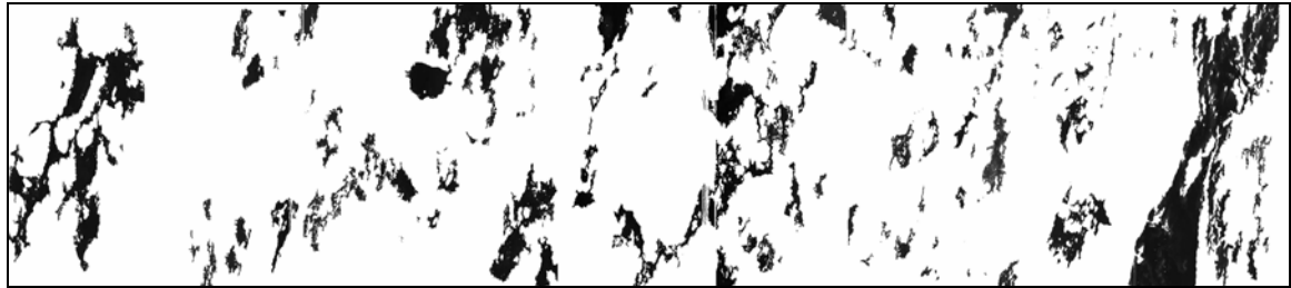
(b) 7 天齡期孔隙分佈圖(孔隙率=16.55%)
