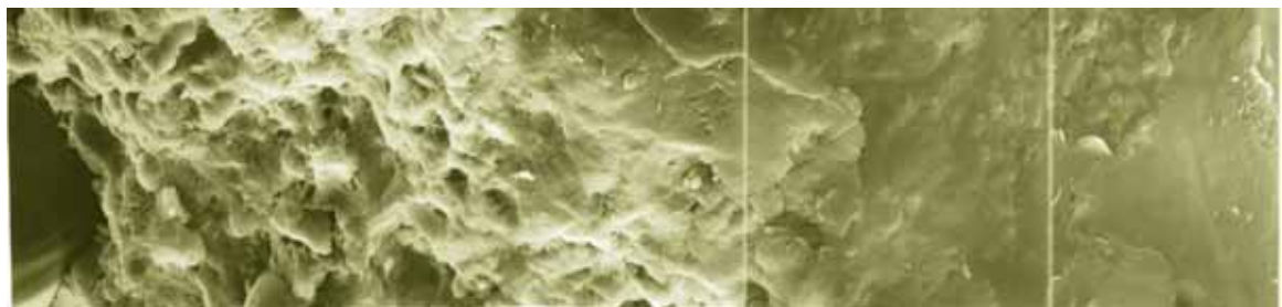
(d) 0.65 水膠比 28 天齡期微觀晶相圖
