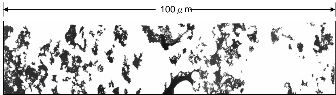
(a) 1 天齡期孔隙分佈圖(孔隙率=20.14%)
