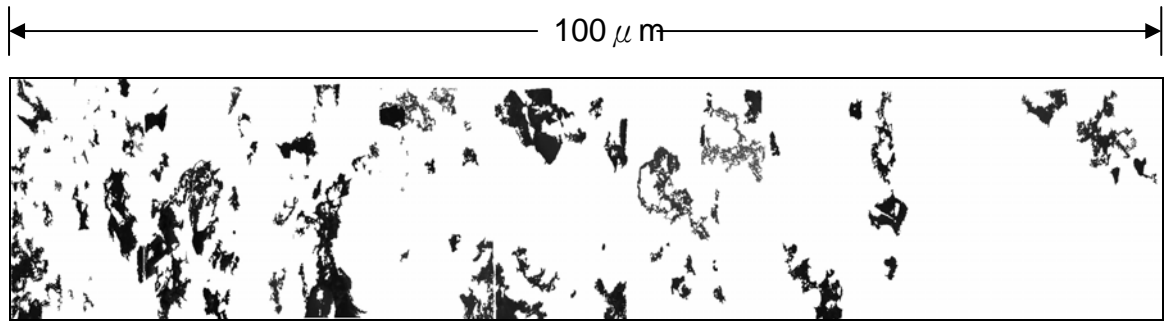
(a) 1 天齡期孔隙分佈圖(孔隙率=20.44%)
