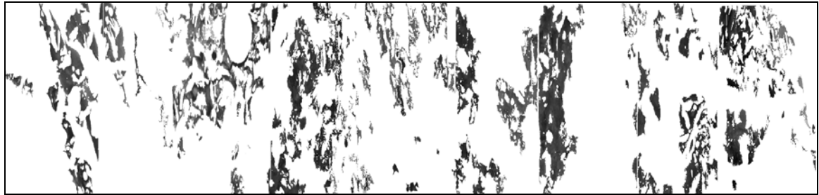
(b) 7 天齡期孔隙分佈圖 (孔隙率 21.30%)
