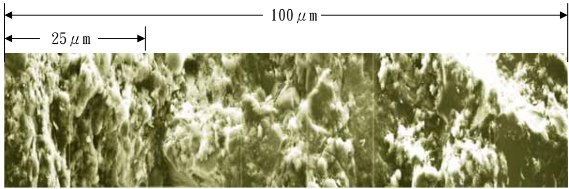
(a) 0.65 水膠比 1 天齡期微觀晶相圖
