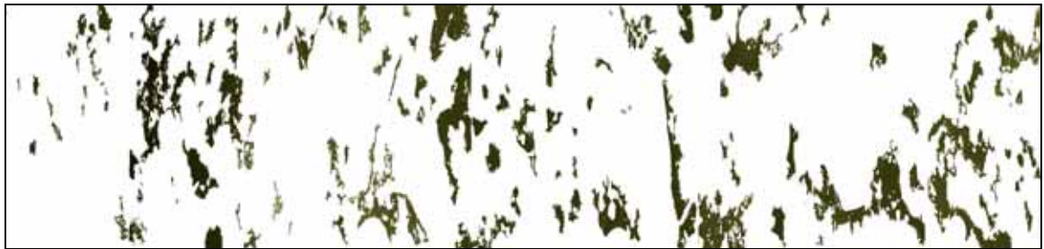
(c) 14 天齡期孔隙分佈圖 (孔隙率 11.53%)
