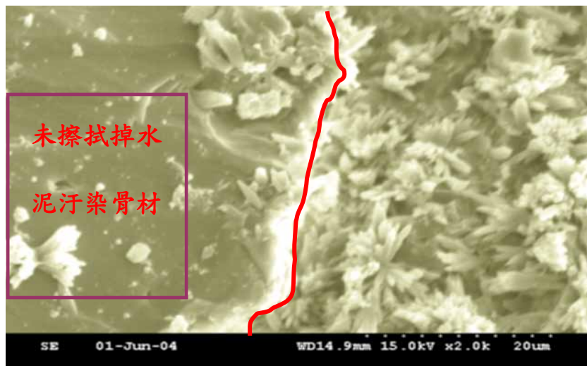
(b) 擦拭後
