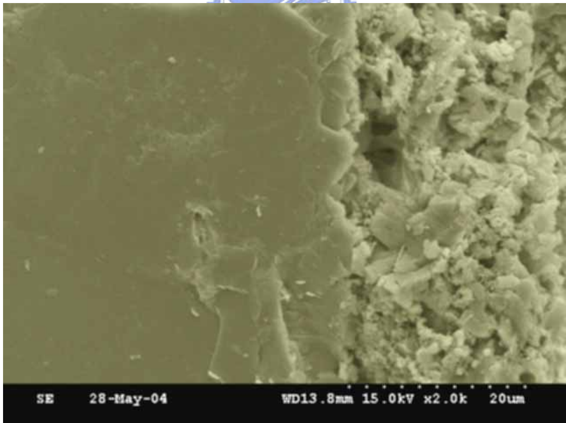
圖 7-2 片狀石頭之 2000 倍全視圖
