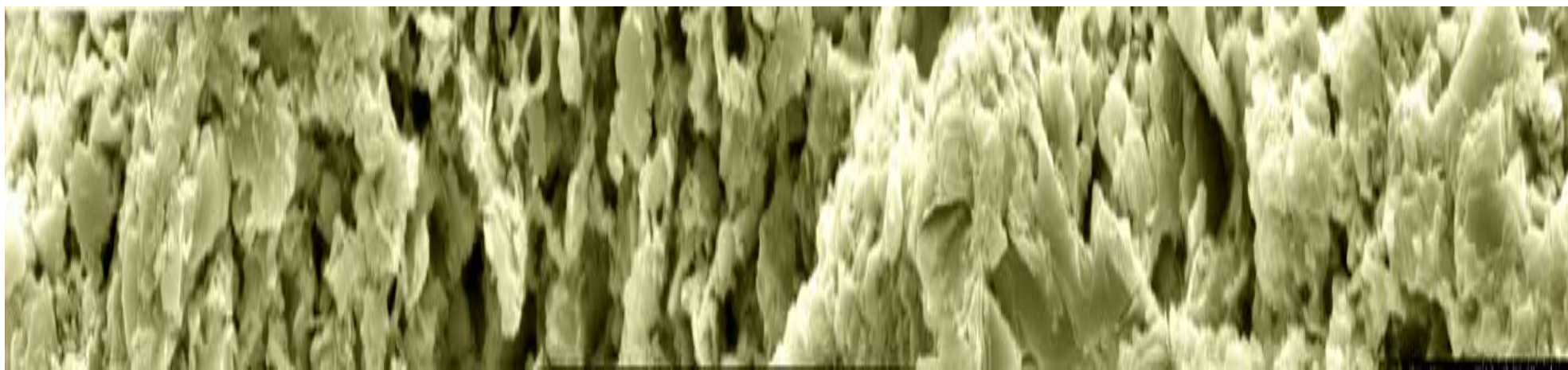
圖 7-3 蜂巢狀石頭 10000 倍之微觀晶相圖
