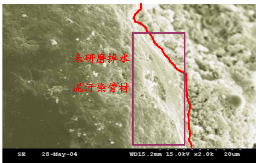
(c) 研磨後
