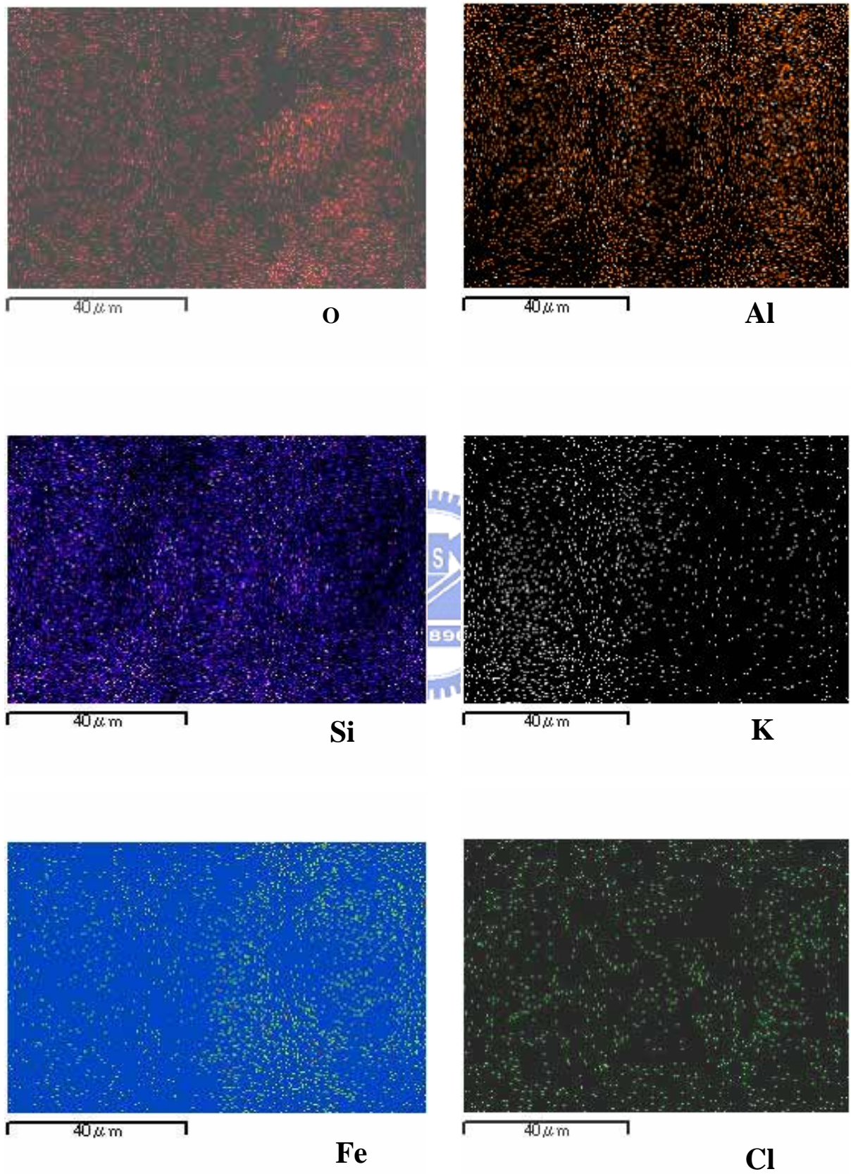
圖 7-28 片狀石頭之 2000 倍 mapping 圖
