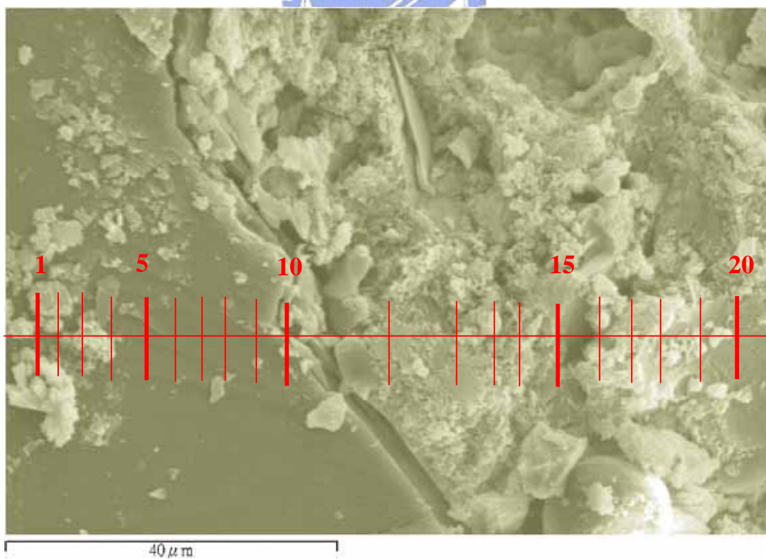
圖 7-24 W/B=0.54 飽和石灰水養護 7 天齡期擦拭後 mapping 用之 2000 倍 SEM 圖及 EDS 位置
