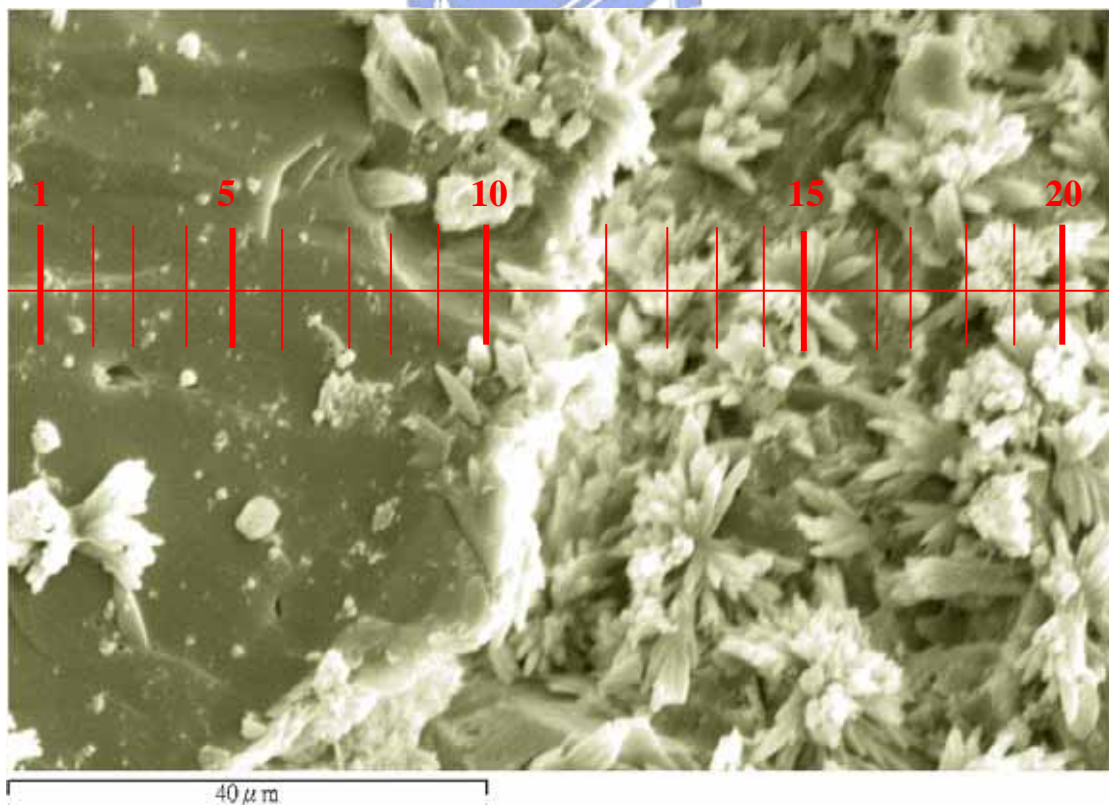
圖 7-26 W/B=0.54 飽和石灰水養護 28 天齡期擦拭後 mapping 用之 2000 倍 SEM 圖及 EDS 位置
