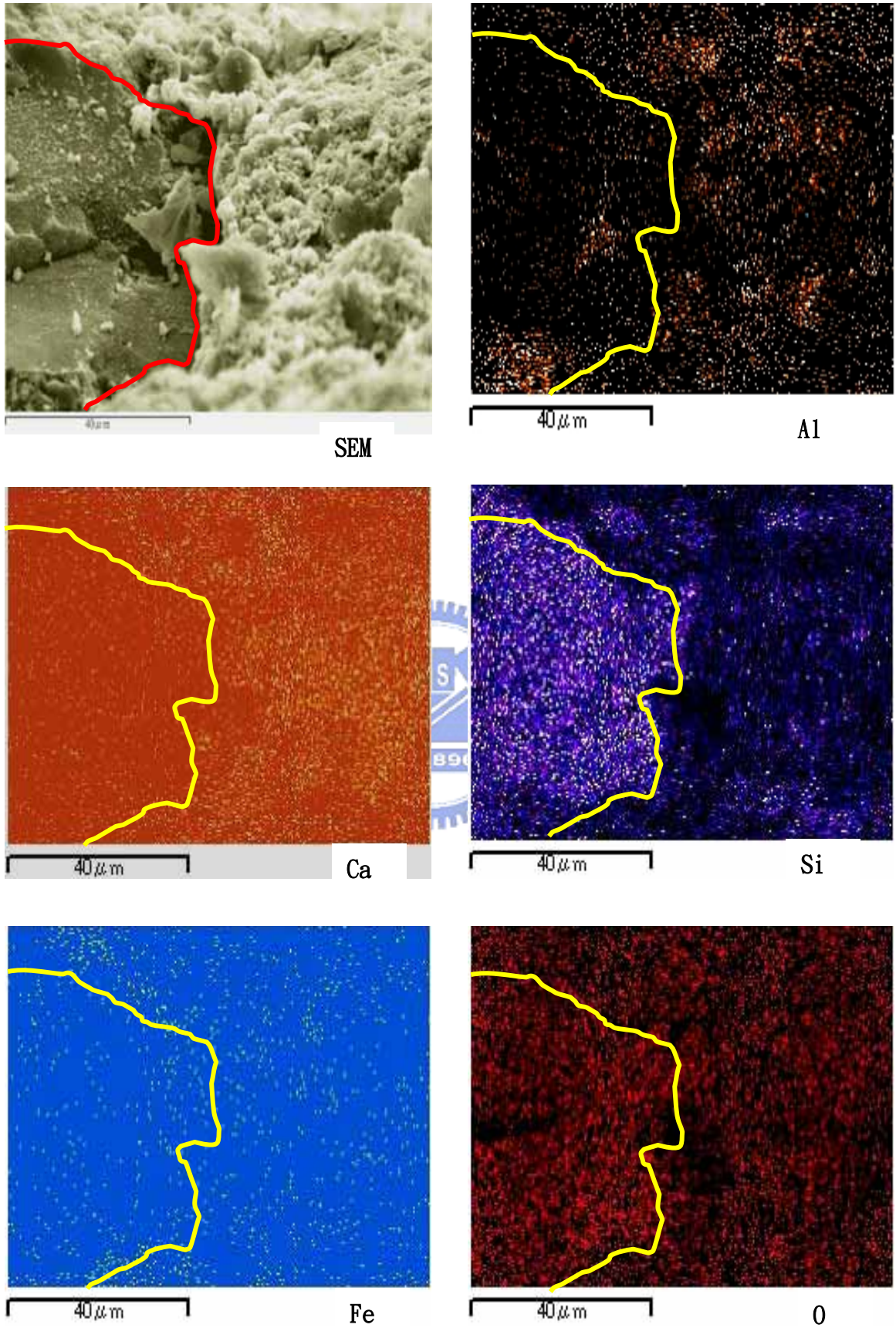
圖 7-29 W/B=0.54 飽和石灰水養護 1 天齡期擦拭後之 2000 倍 mapping 圖
