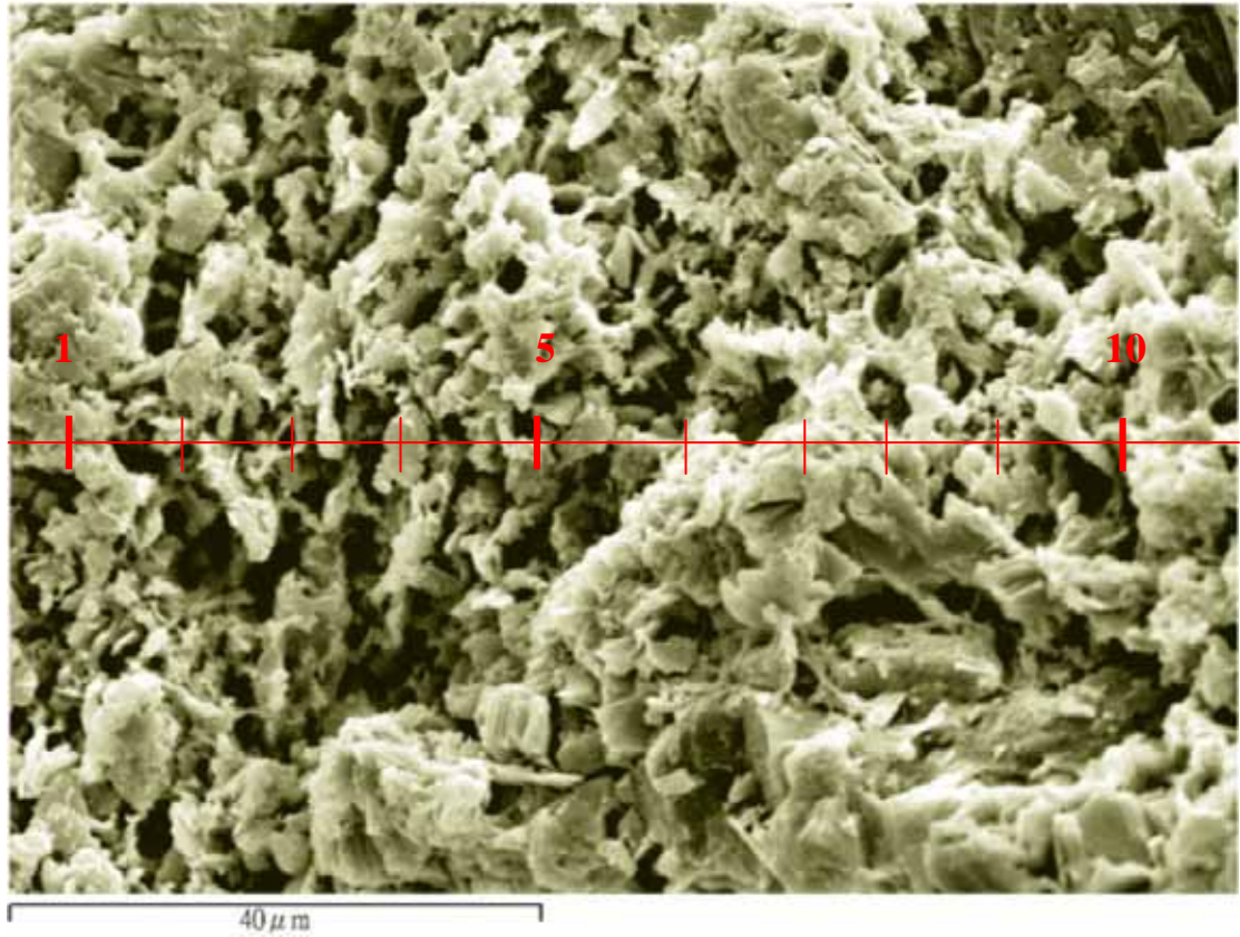
圖 7-21 蜂巢狀石頭 mapping 用之 2000 倍 SEM 圖及 EDS 位置
