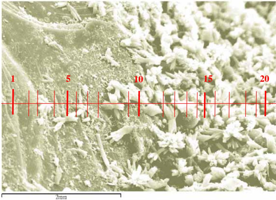
圖 7-25 W/B=0.54 飽和石灰水養護 14 天齡期擦拭後 mapping 用之 2000 倍 SEM 圖及 EDS 位置
