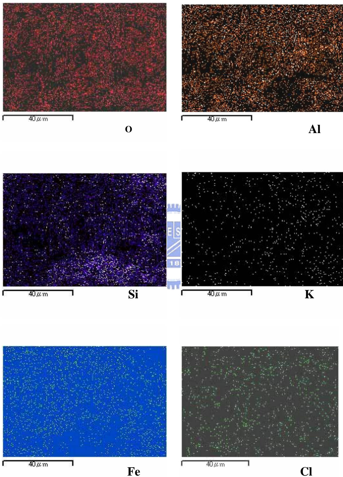
圖 7-27 蜂巢狀石頭之 2000 倍 mapping 圖
