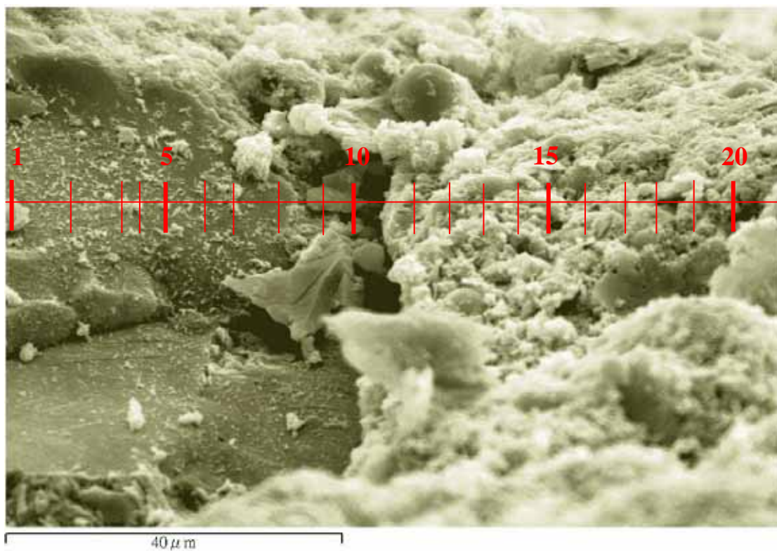
圖 7-23 W/B=0.54 飽和石灰水養護 1 天齡期擦拭後之 mapping 用之 2000 倍 SEM 圖及 EDS 位置
