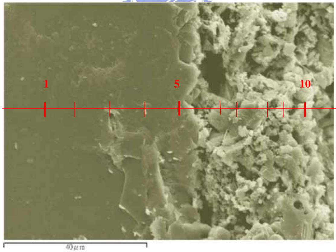
圖 7-22 片狀石頭 mapping 用之 2000 倍 SEM 圖及 EDS 位置
