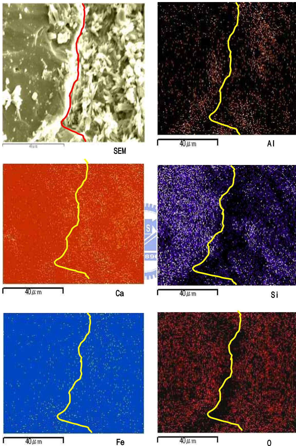
圖 7-32 W/B=0.54 飽和石灰水養護 28 天齡期擦拭後之 2000 倍 mapping 圖
