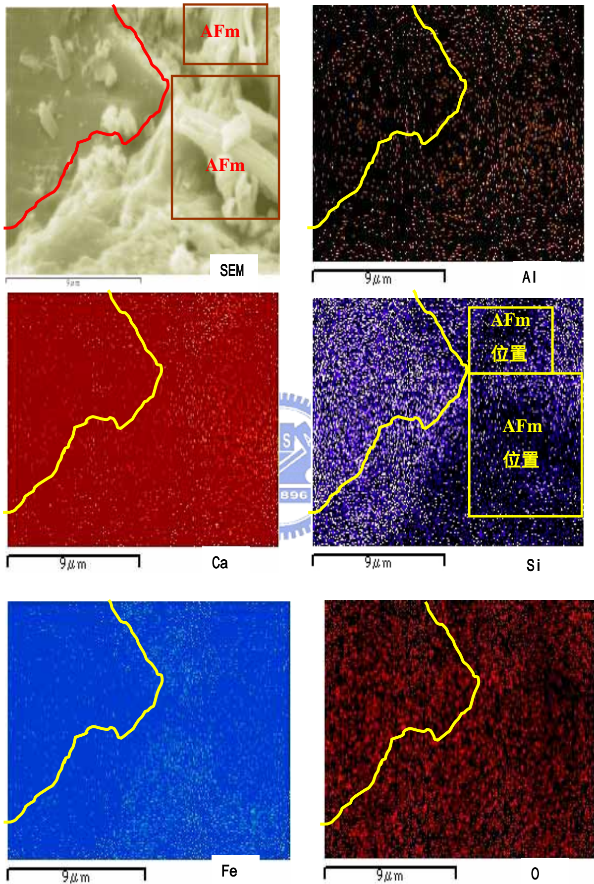
圖 7-34 W/B=0.54 飽和石灰水養護 1 天之 10000 倍 mapping 圖
