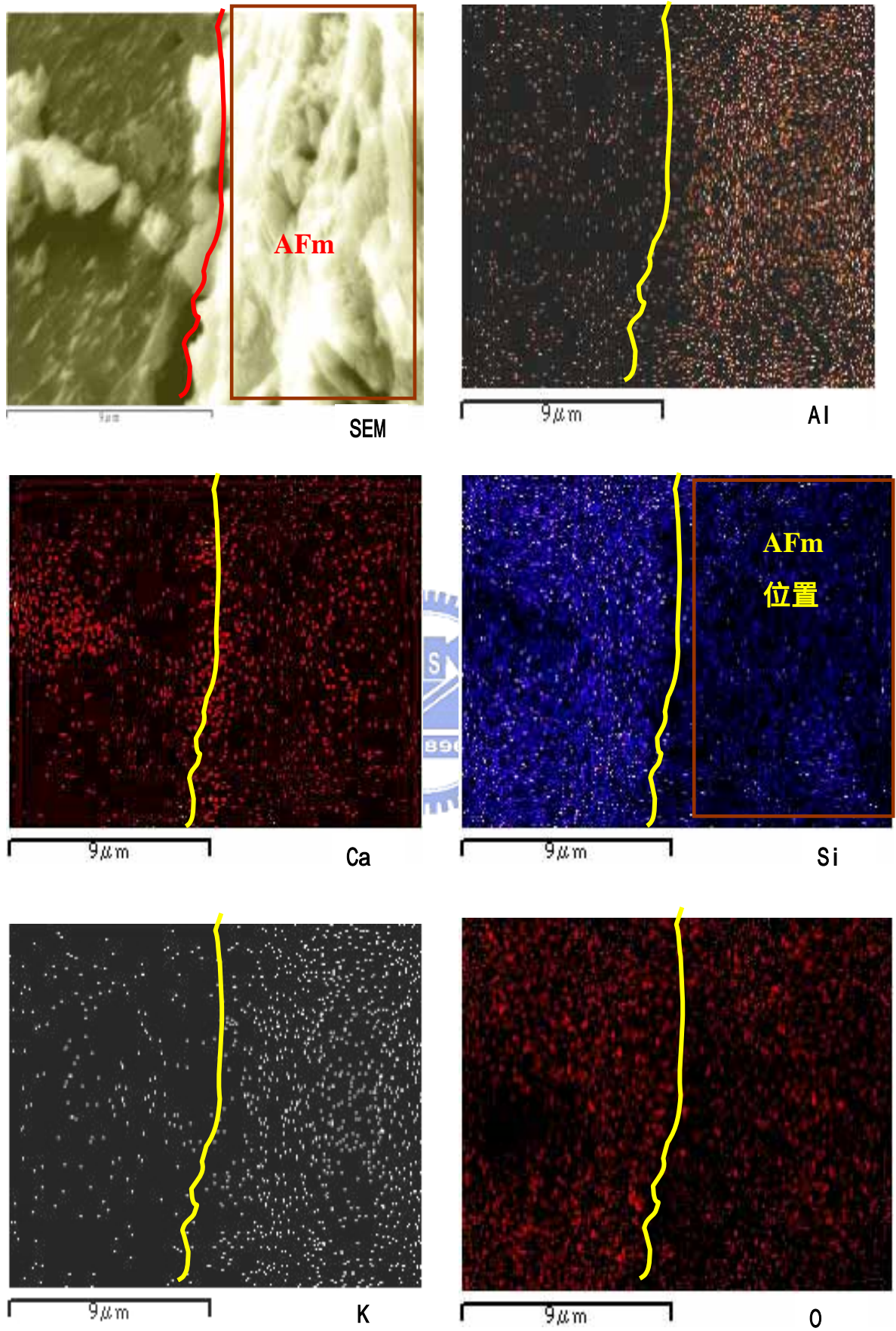
圖 7-35 W/B=0.54 飽和石灰水養護 7 天之 10000 倍 mapping 圖
