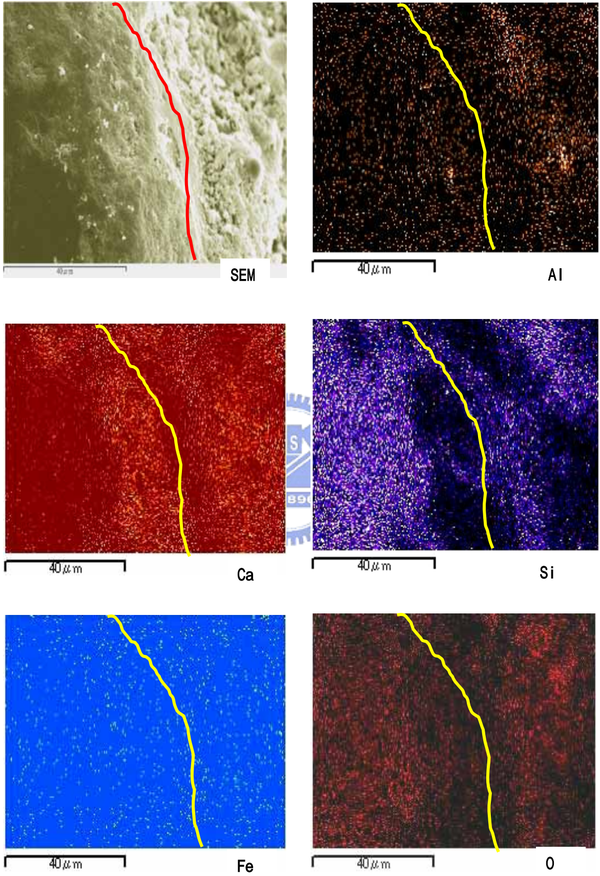
圖 7-30 W/B=0.54 飽和石灰水養護 7 天齡期擦拭後之 2000 倍 mapping 圖
