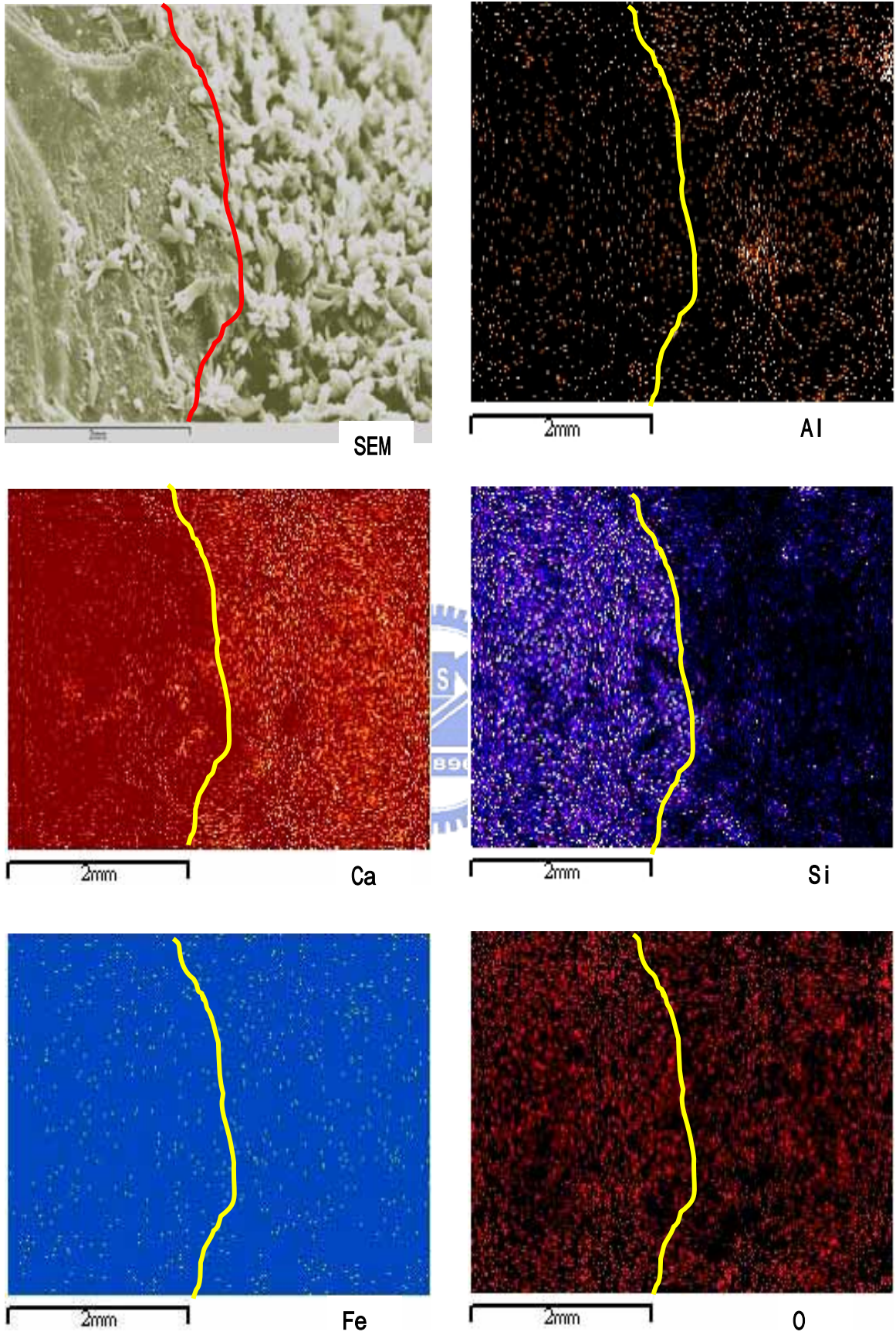
圖 7-31 W/B=0.54 飽和石灰水養護 14 天齡期擦拭後之 2000 倍 mapping 圖
