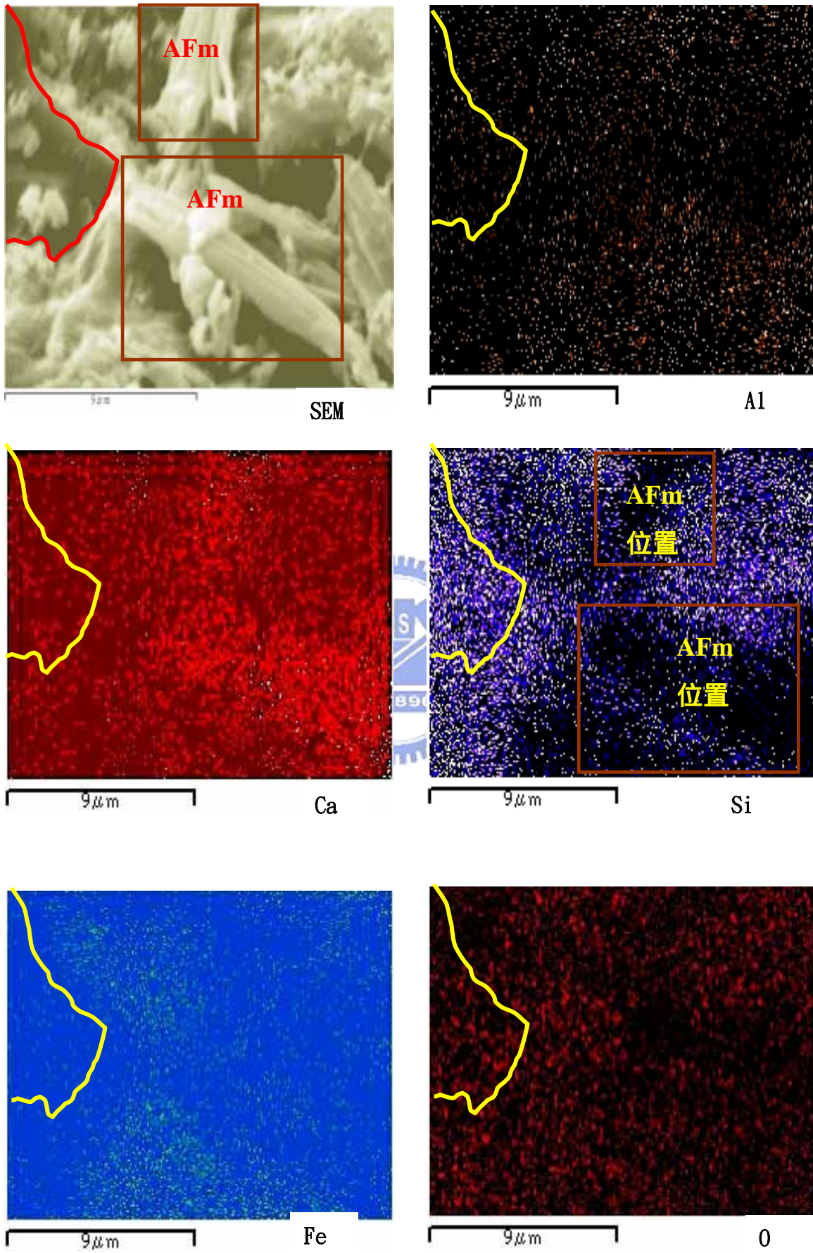
圖 7-38 W/B=0.54 飽和石灰水養護 1 天水泥漿之 10000 倍 mapping 圖
