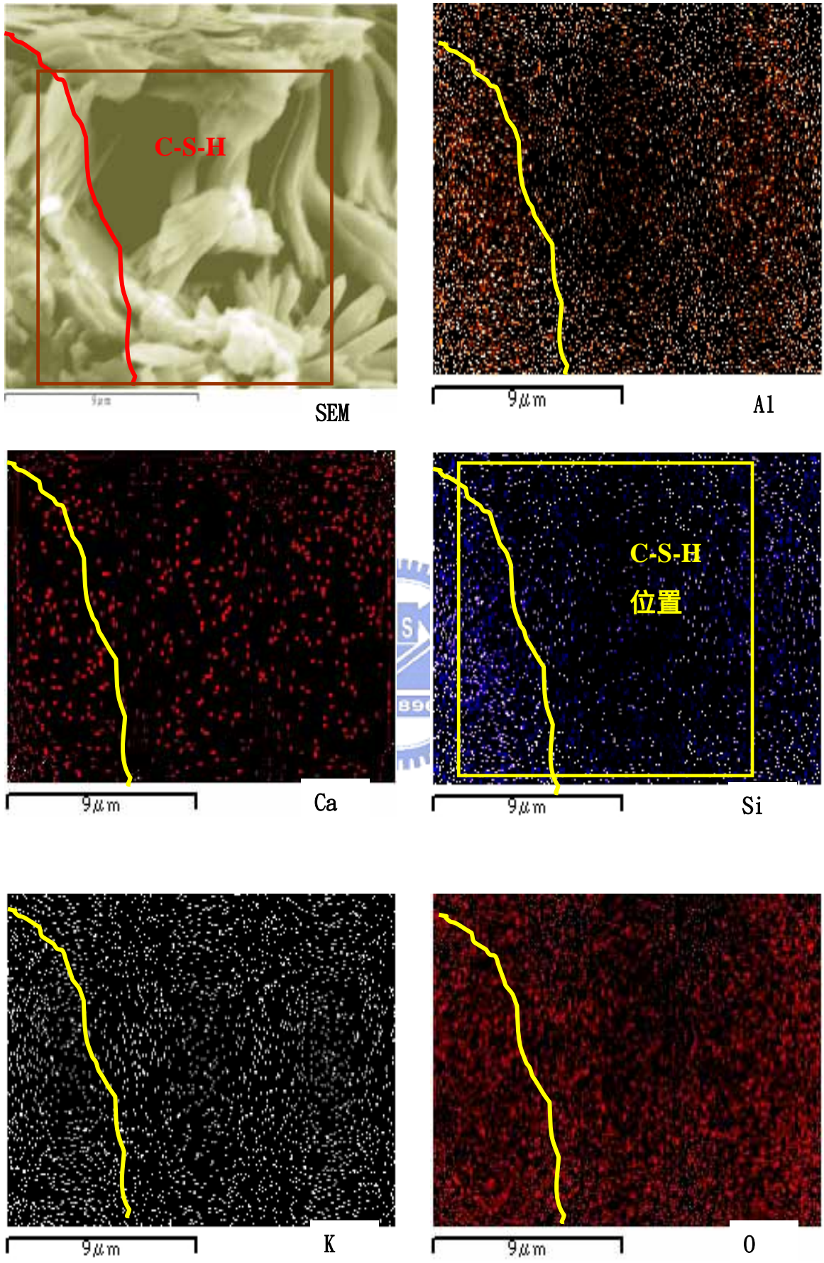
圖 7-41 W/B=0.54 飽和石灰水養護 28 天水泥漿之 10000 倍 mapping 圖
