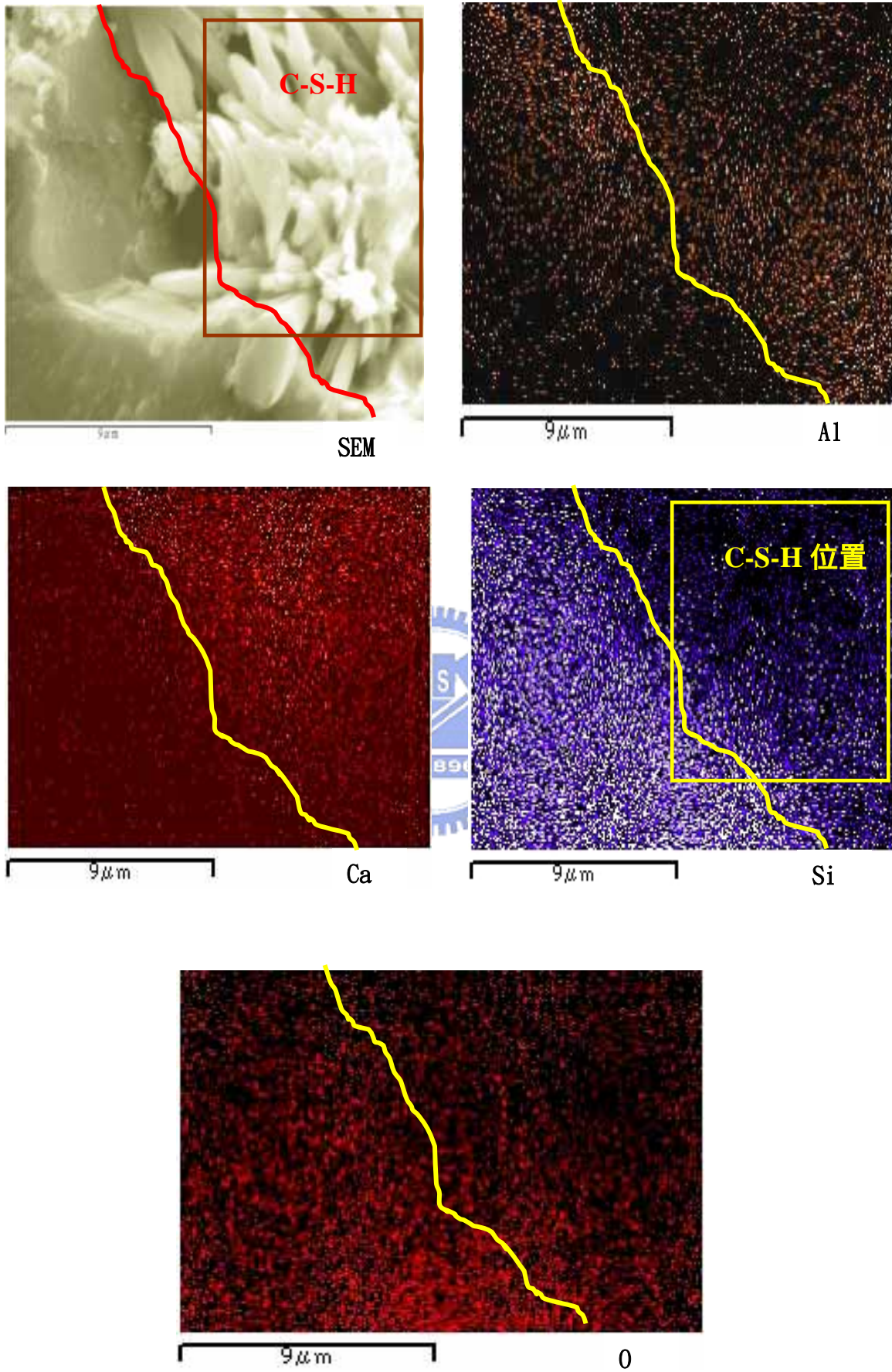
圖 7-37 W/B=0.54 飽和石灰水養護 28 天之 10000 倍 mapping 圖
