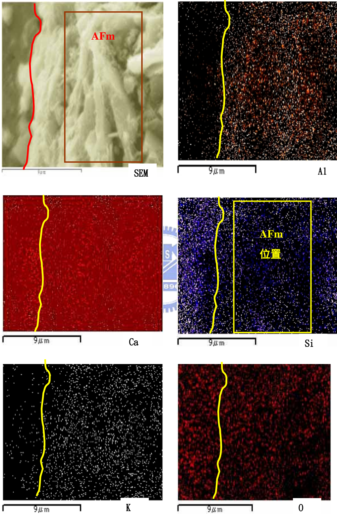
圖 7-39 W/B=0.54 飽和石灰水養護 7 天水泥漿之 10000 倍 mapping 圖
