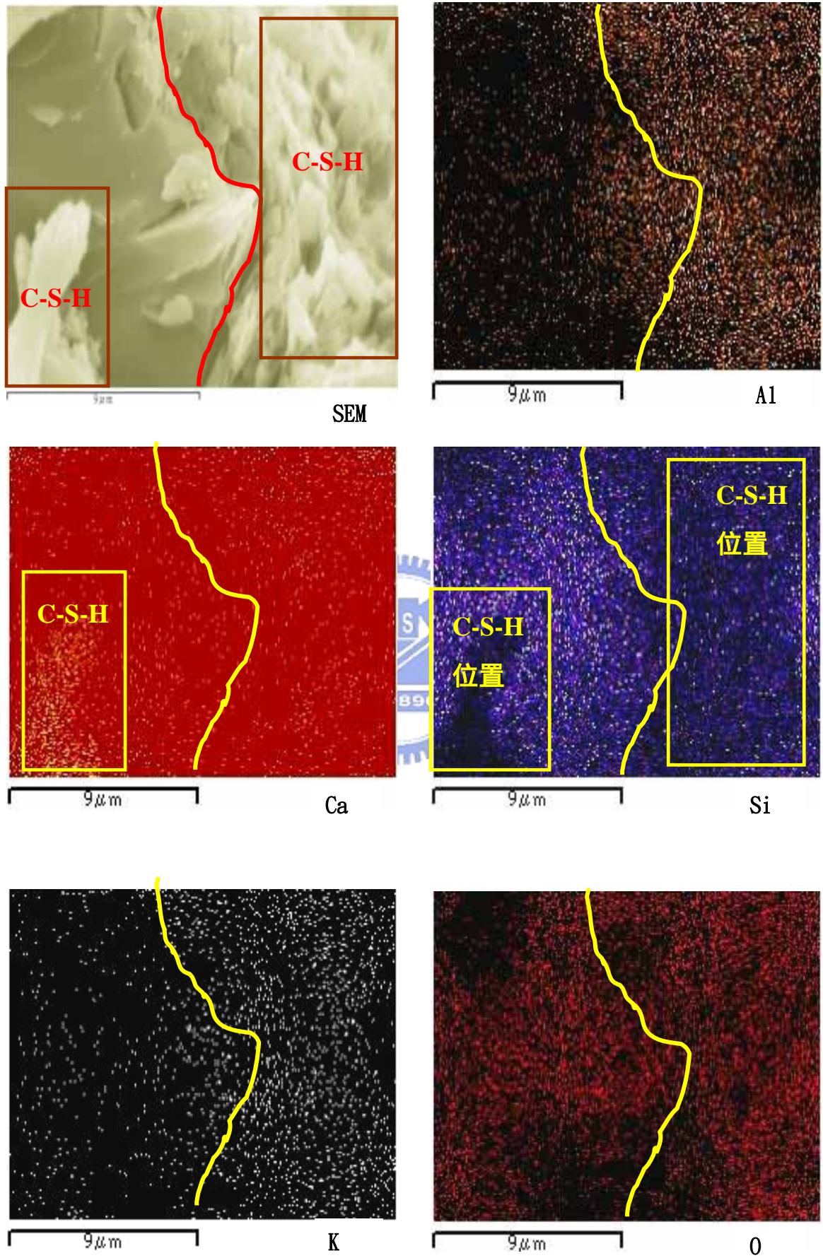
圖 7-36 W/B=0.54 飽和石灰水養護 14 天之 10000 倍 mapping 圖
