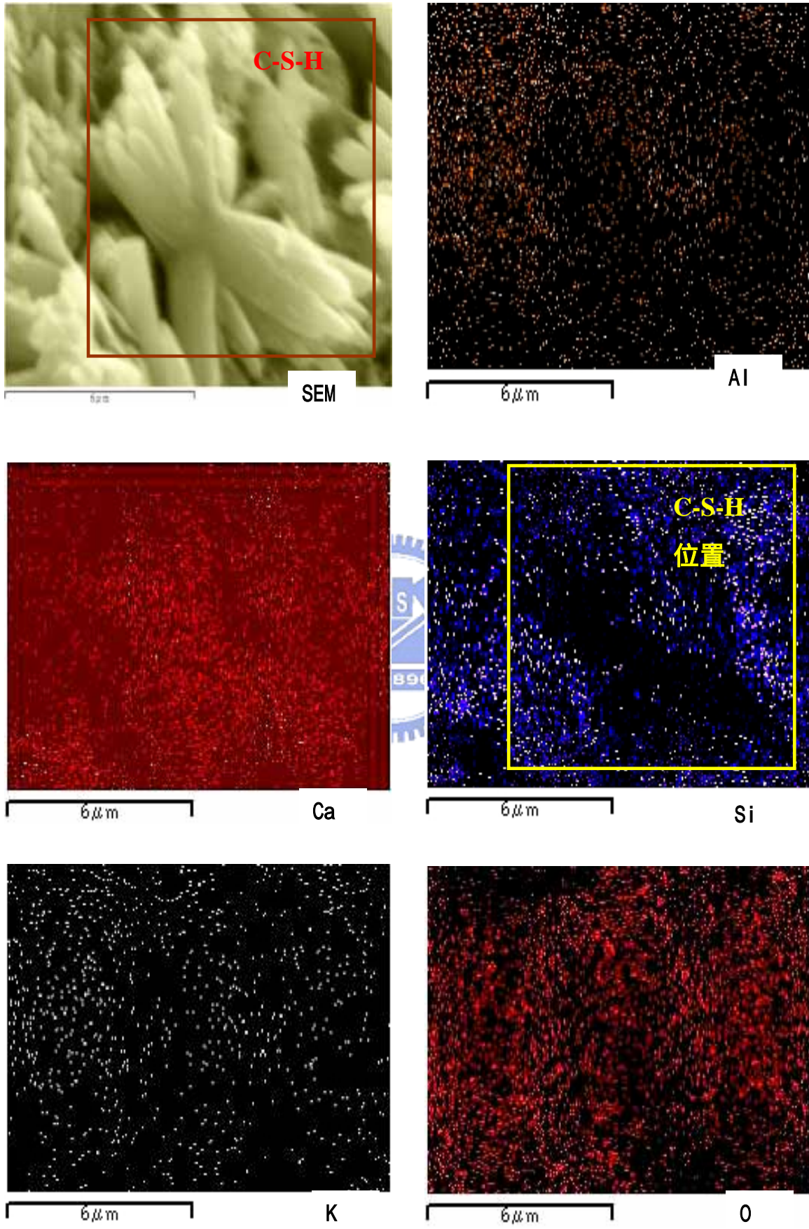
圖 7-44 W/B=0.54 飽和石灰水養護 14 天 C-S-H 整體之 15000 倍 mapping 圖
