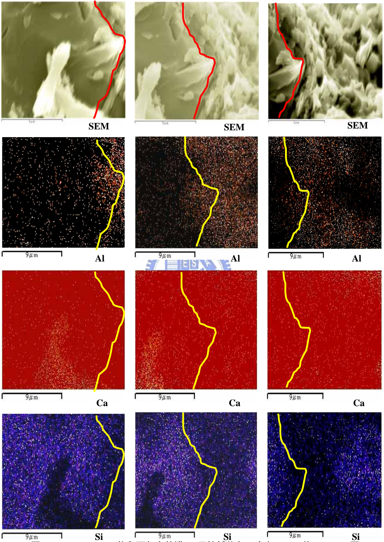
圖 7-48 W/B=0.54 飽和石灰水養護 14 天擦拭後各元素之 10000 倍 mapping 圖
