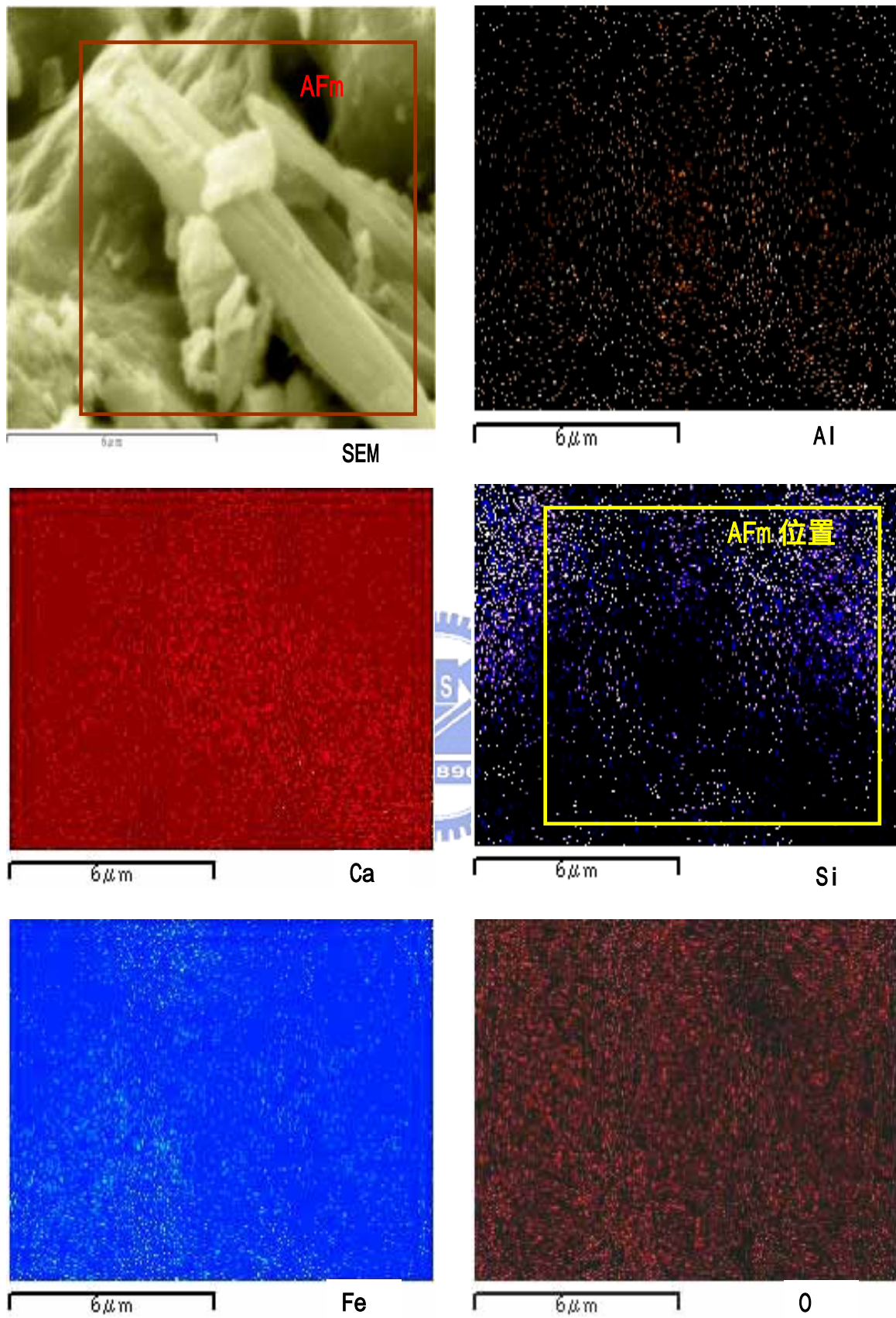
圖 7-47 W/B=0.54 飽和石灰水養護 1 天 AFm 整體之 15000 倍 mapping 圖
