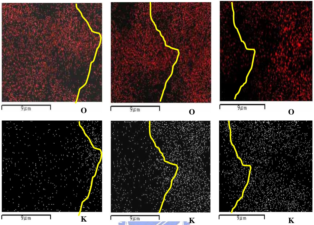
圖 7-49 W/B=0.54 飽和石灰水養護 14 天擦拭後各元素之 10000 倍 mapping 圖(續)
