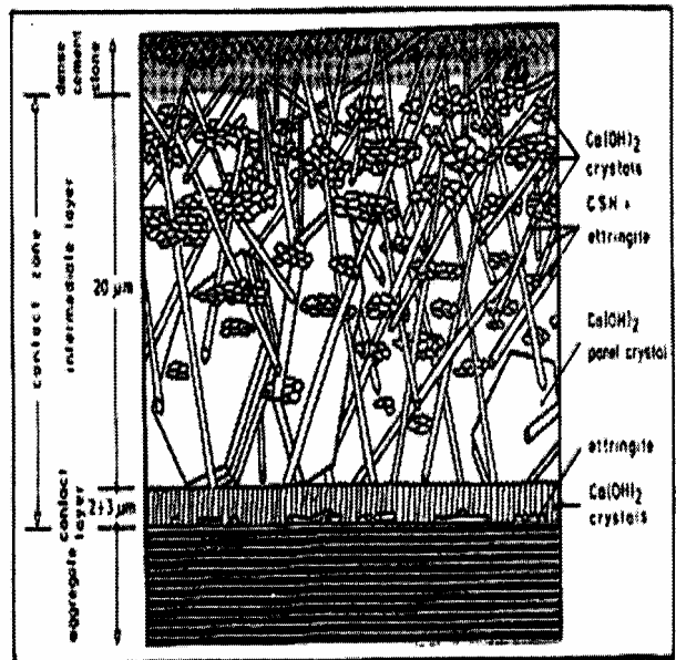
圖 2-3 Zimbelmann 模型 [14]
