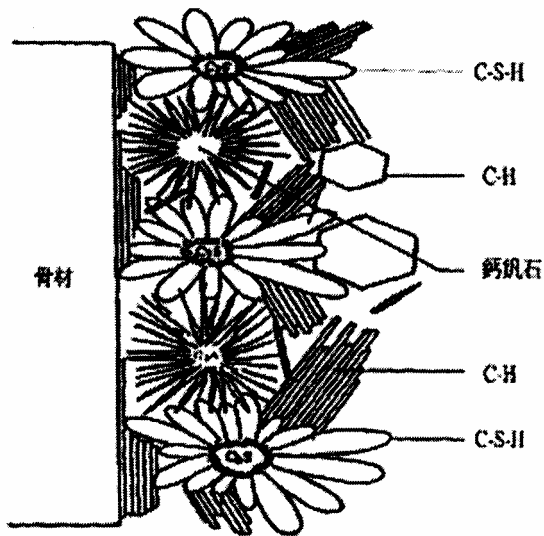
圖 2-2 Ollivier-Grandet 模型 [13]
