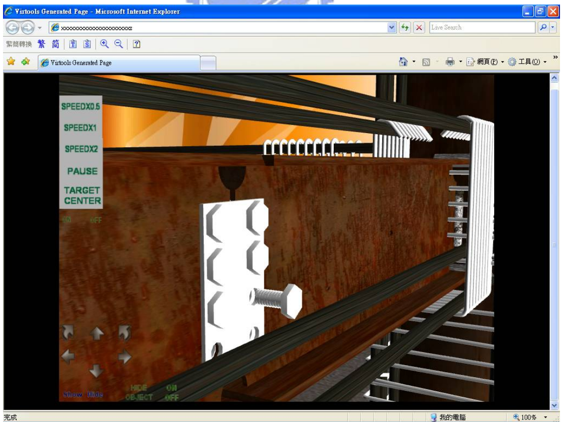
圖6-15 接合板正使用螺栓接合(正面)
