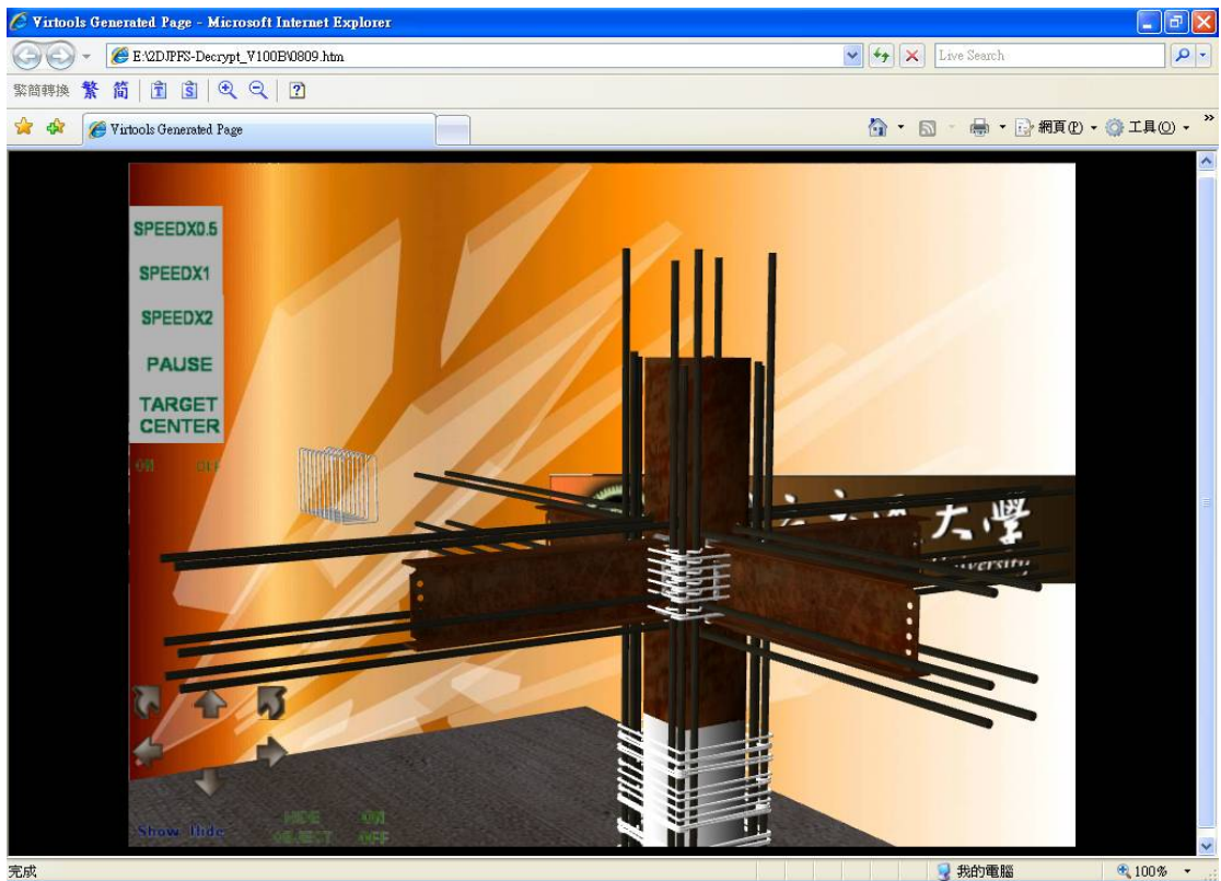
圖6-10 雙向梁主筋穿過鋼筋預留孔至指定位置
