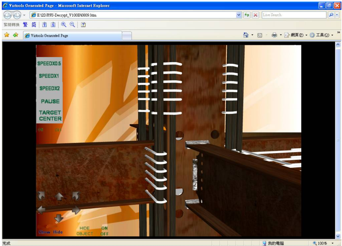
圖6-8 梁柱接頭箍筋組合正放置到定位
