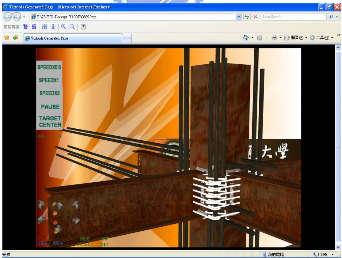
圖6-9 完成組裝後的梁柱接頭箍筋
