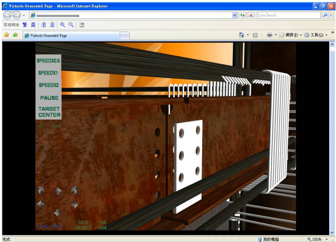
圖6-14 孔位對齊後加上接合板
