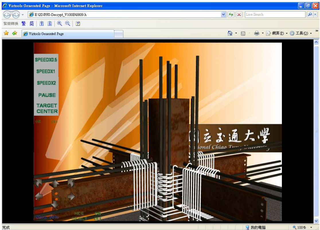
圖6-12 梁箍筋堆疊於靠近梁柱接頭側
