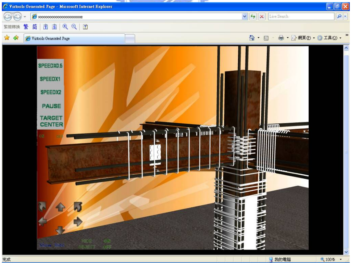
圖6-19 梁箍筋移動至指定位置
