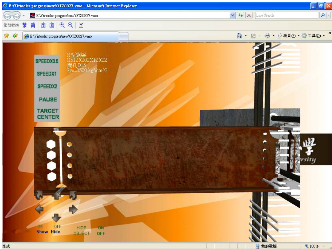
圖 6-30 隱藏H型鋼樑以外的物件
