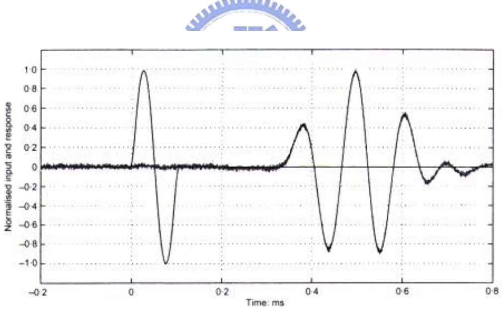
圖 2.6 剪力波傳送及接收訊號結果 (Ling and Greening, 2001)
