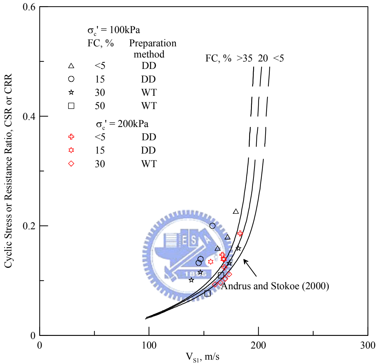
圖 4.23 Kawaguchi et al. (2001) A 點-CRR 與 V_{sl} 之關係
