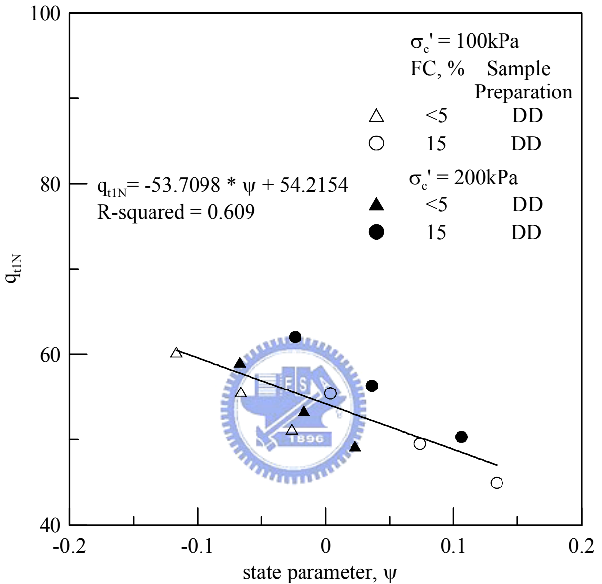
圖 4.10 排水行為下麥寮砂 q_{t1N} 與狀態參數之關係 ( K=0.5 )
