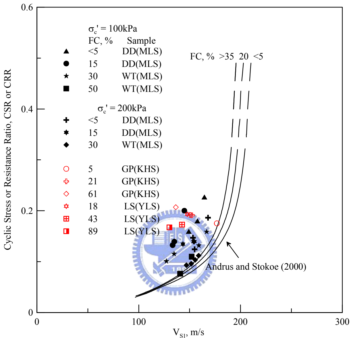
圖 5.27 麥寮砂、員林砂與高雄砂 CRR-V_{sl} 液化臨界曲線
