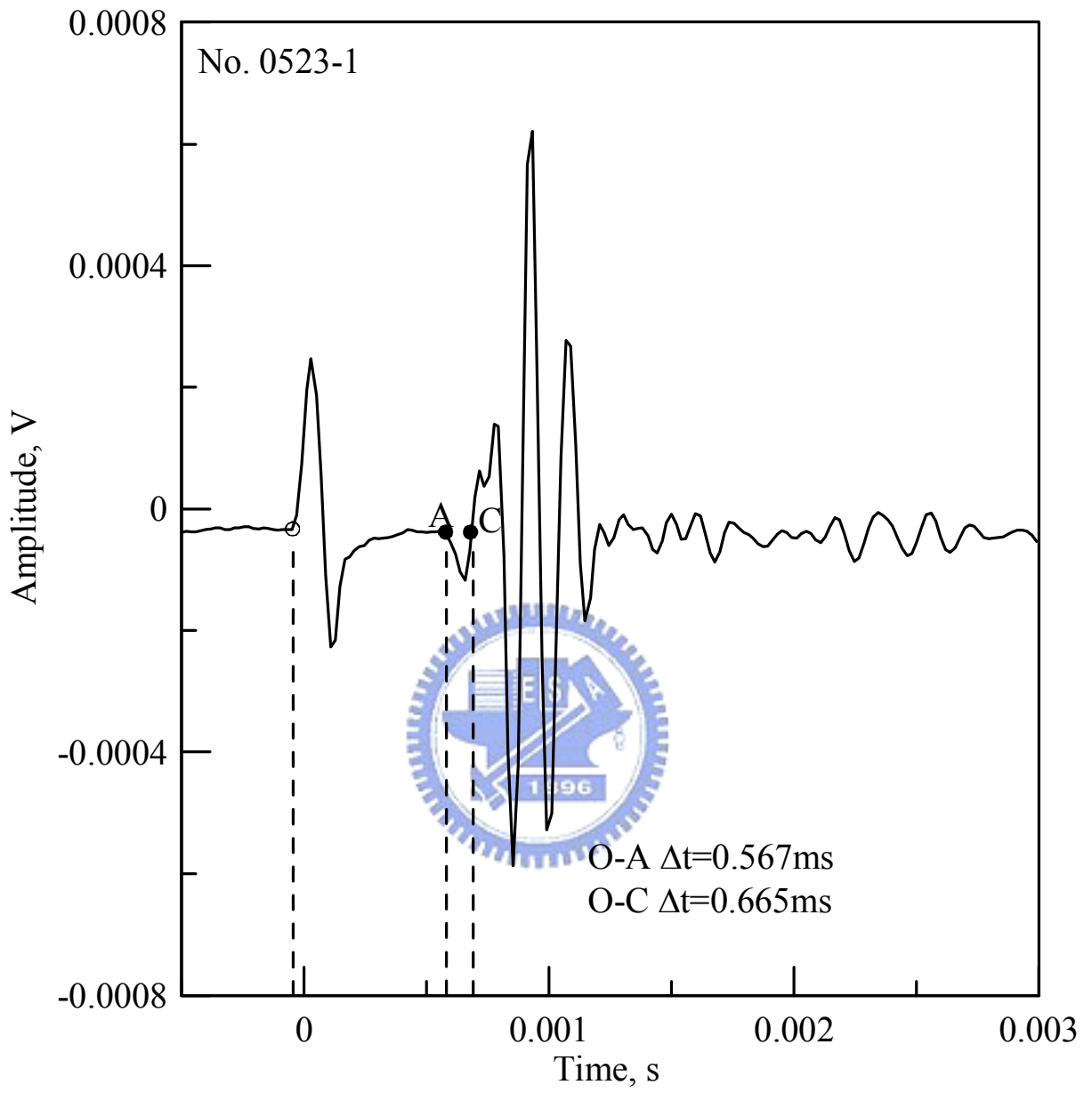
圖 4.17 剪力波到達時間判斷圖
