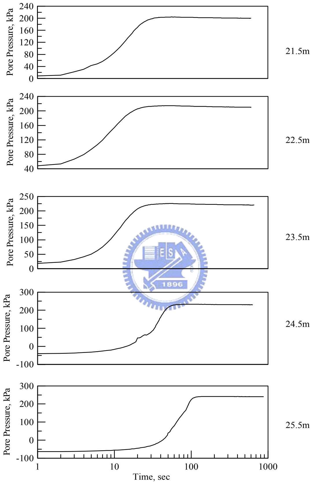
圖 5.20 高雄場址 CPT 孔隙水壓消散試驗結果 (21.5m~25.5m)
