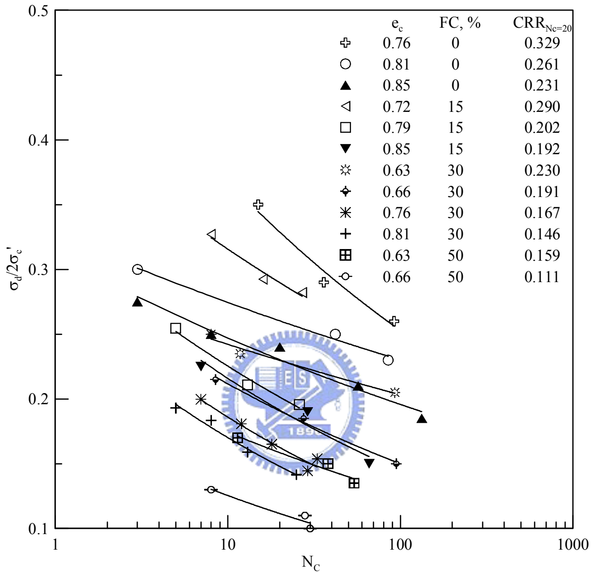
圖 4.4 動態三軸試驗結果 ( \sigma'_c=100\text{kPa} )
