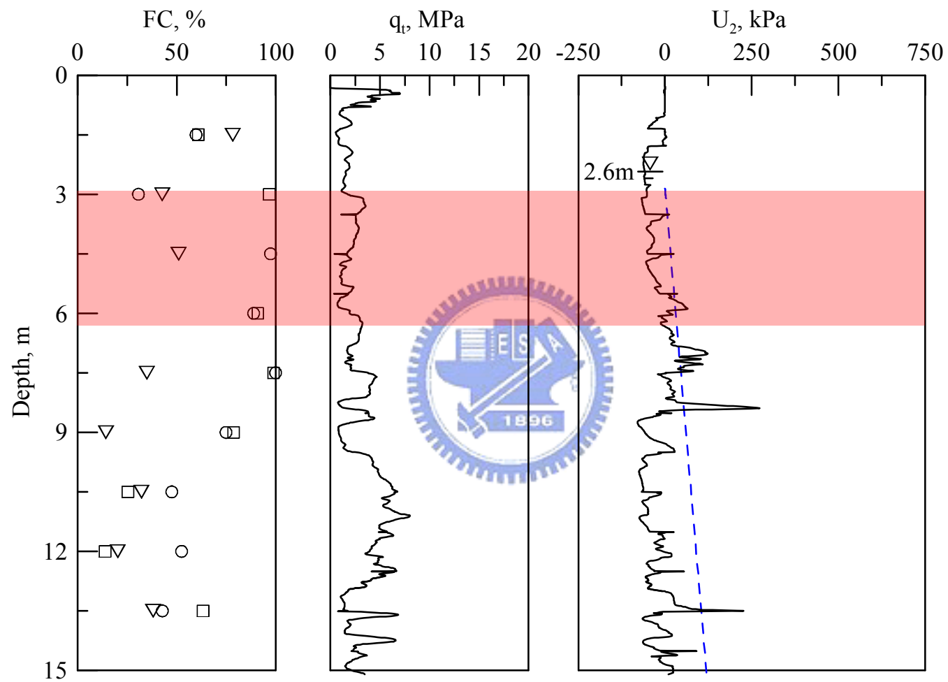
圖 5.13 員林場址 CPT 試驗結果
