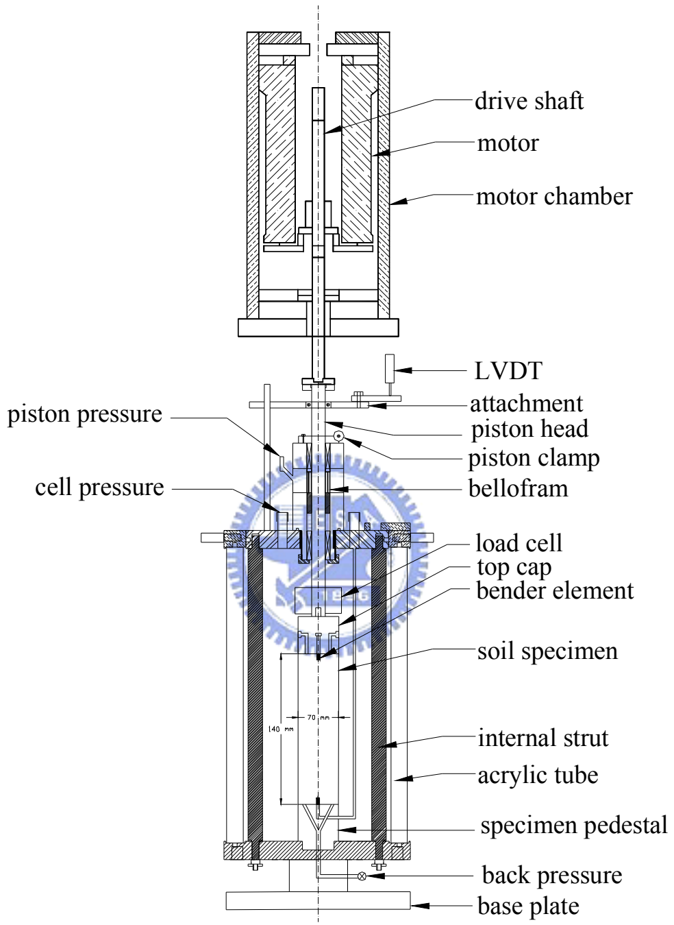
圖 3.4 三軸試驗設備設計示意圖
