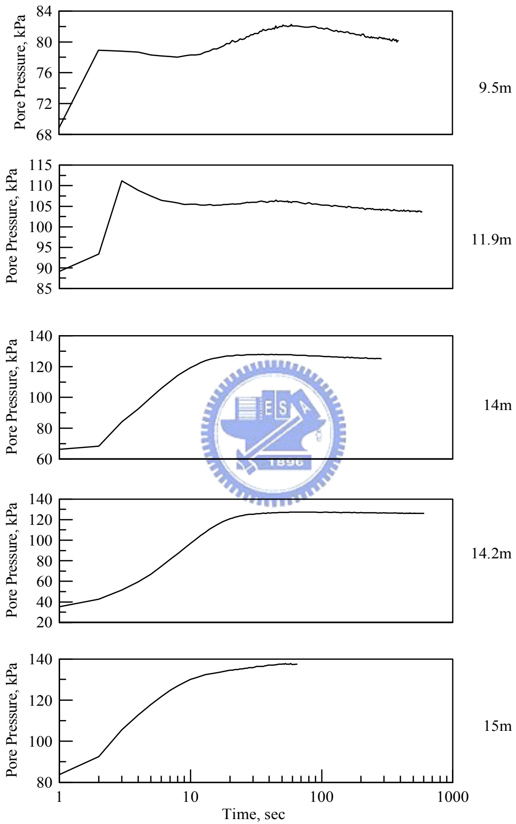
圖 5.18 高雄場址 CPT 孔隙水壓消散試驗結果 (9.5m~15m)
