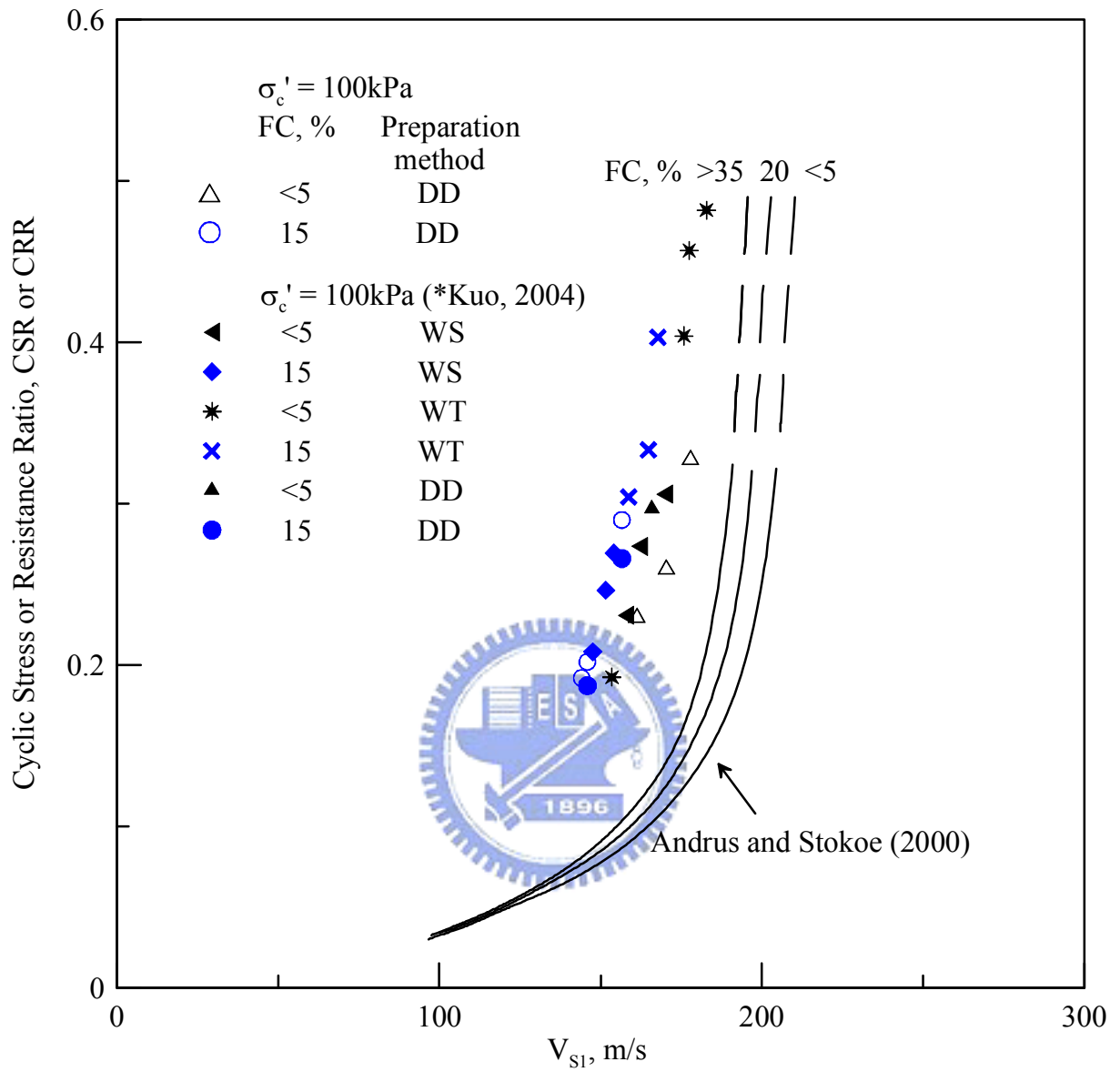
圖 4.20 麥寮砂 CRR 與 V_{S1} 關係圖 (FC<5%、FC=15%)
