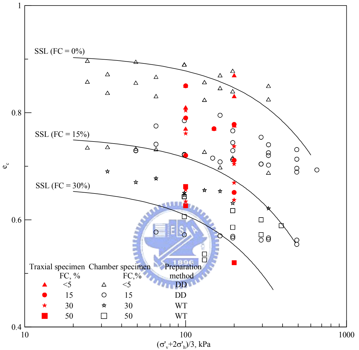
圖 4.6 動態三軸試驗與標定試驗條件關係圖
