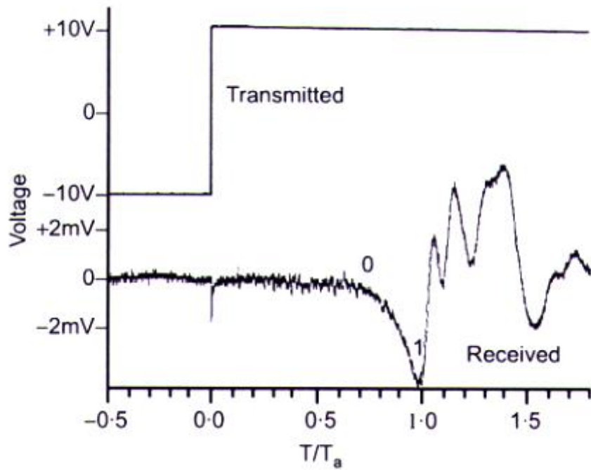
圖 2.8 高嶺土，以方波為激發源 (Jovicic et al., 1996)
