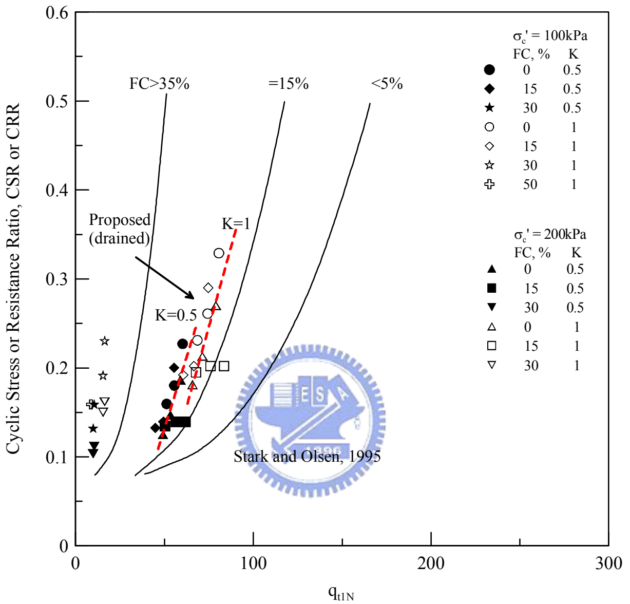
圖 4.13 麥寮砂排水行為下液化臨界線
