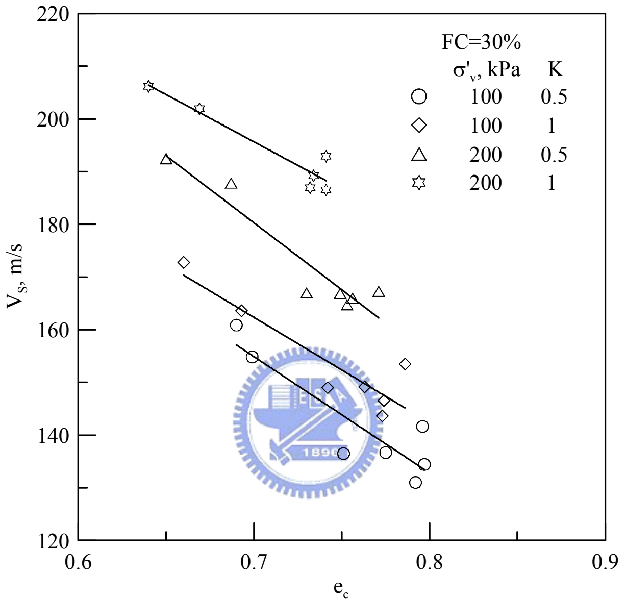
圖 4.16 FC=30%剪力波速與孔隙比在不同應力條件之關係
