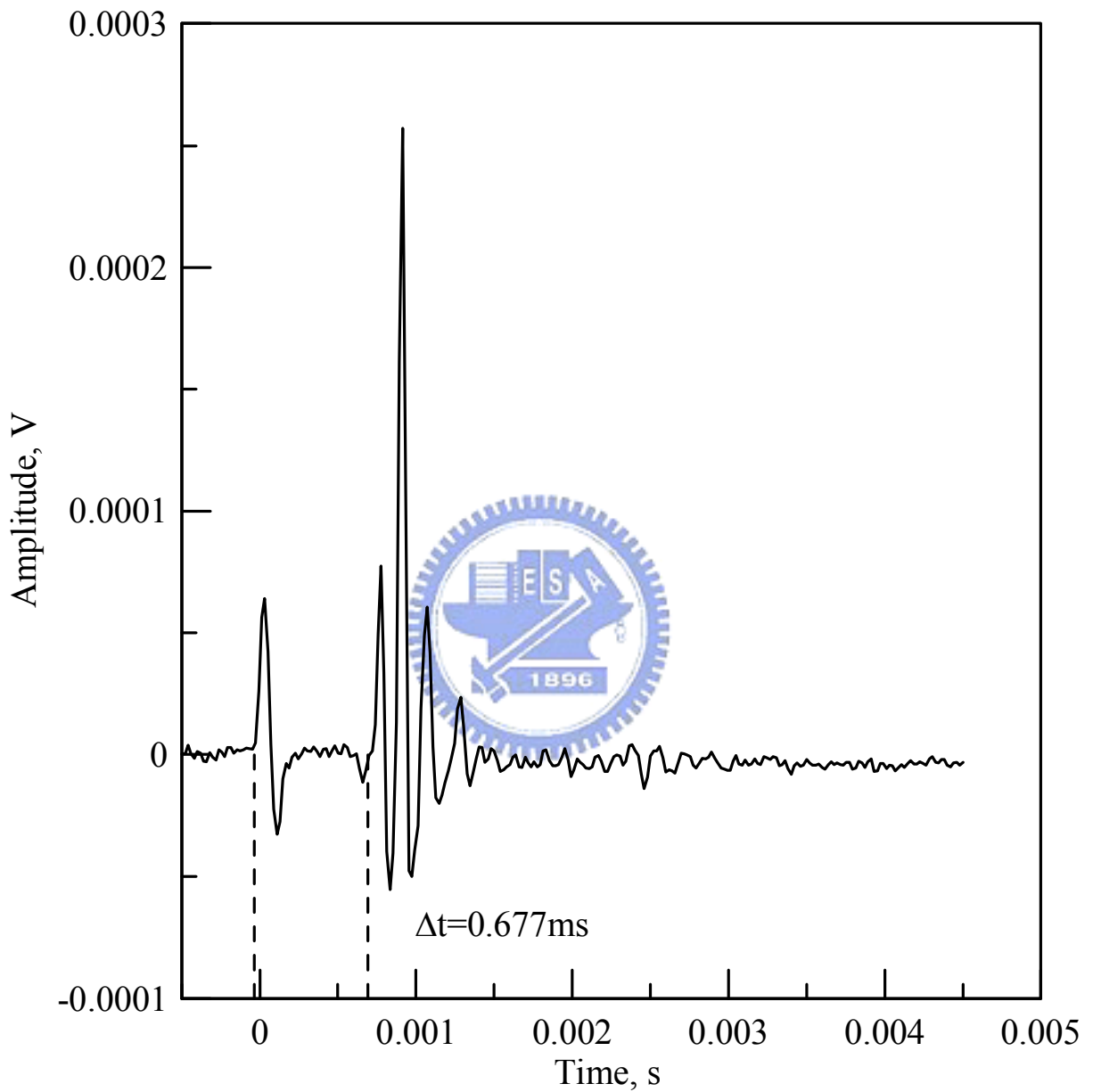
圖 4.3 剪力波傳遞時間圖
