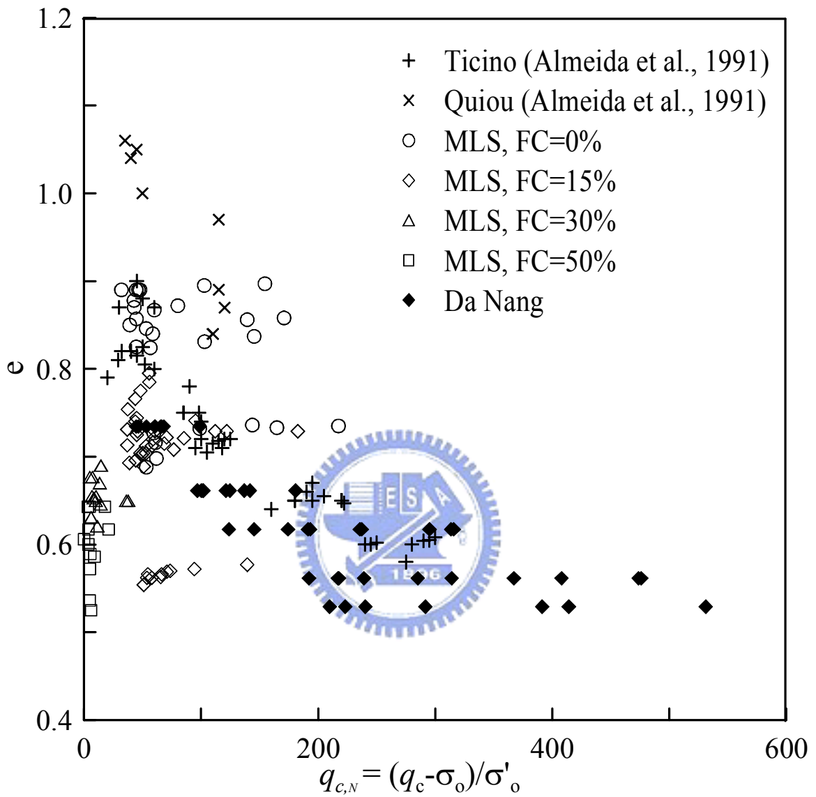
圖 2.22 麥寮砂、Ticino、Quiou 與 Da Nang 砂孔隙比與 q_{c,N} 的關係 (Huang and Hsu, 2004)
