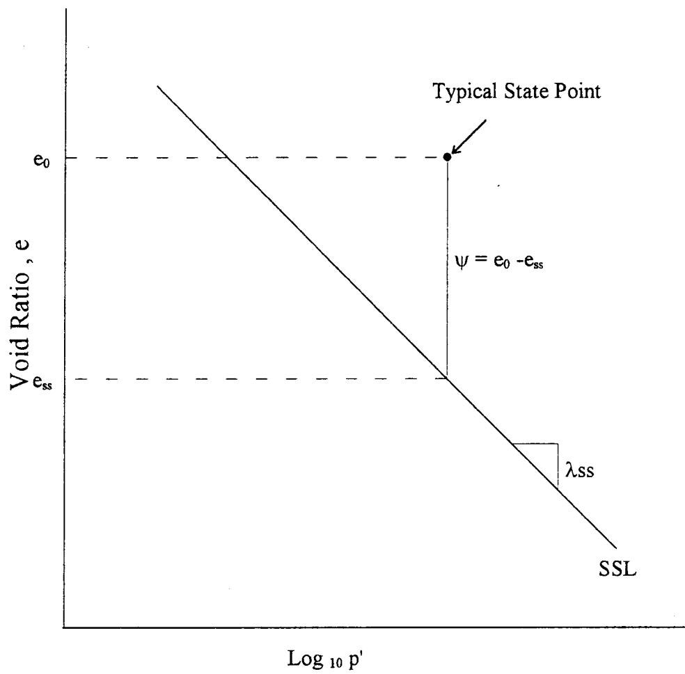
圖 3.3 狀態參數的定義 (Been and Jefferies, 1985)
