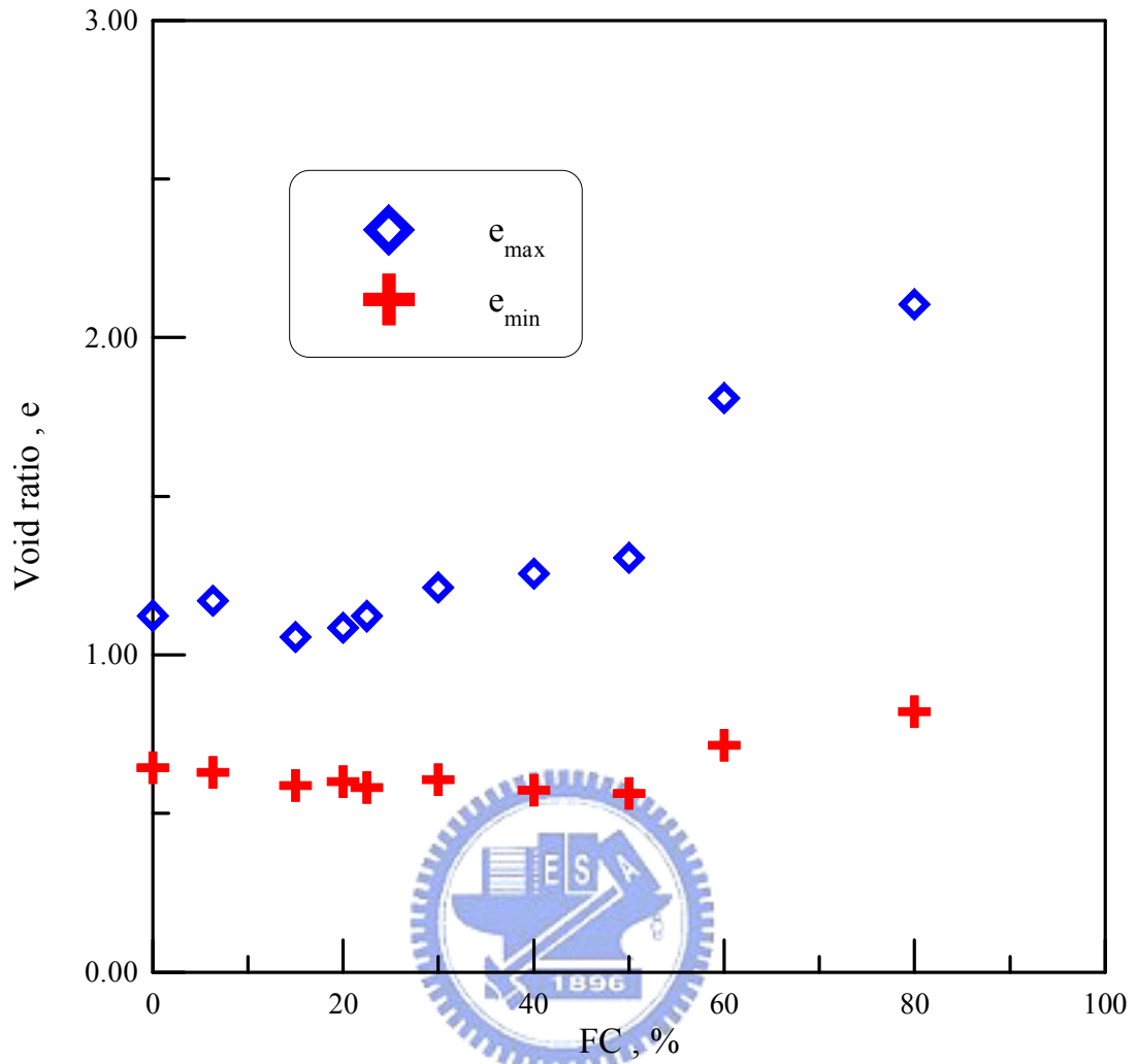
圖 2.12 麥寮砂細粒料含量與最大及最小孔隙比 ( e_{max} 和 e_{min} ) 之關係 (王統立, 2000)
