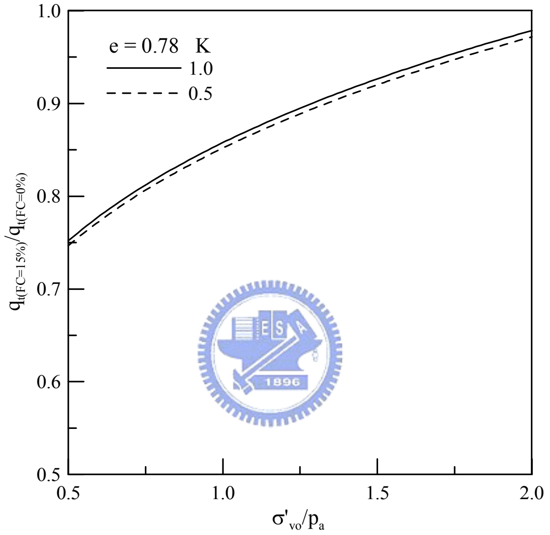
圖 2.24 q_t 與細料含量在不同垂直應力下之關係
