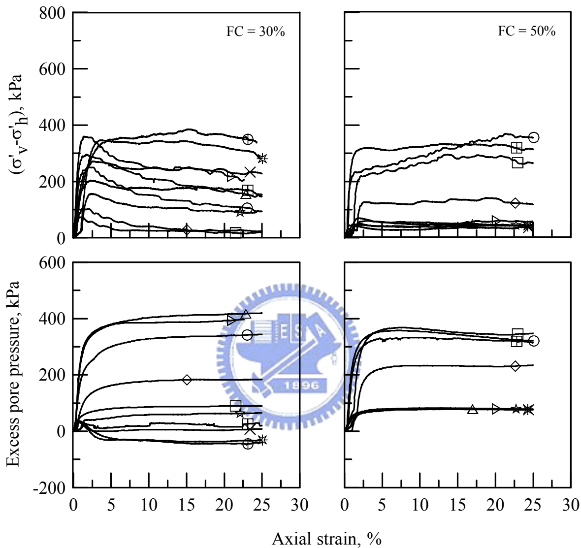
圖 2.16 麥寮砂 FC=30 與 50%三軸試驗應力、應變與超額孔隙水壓之相互關係 (蔡明道, 2002)
