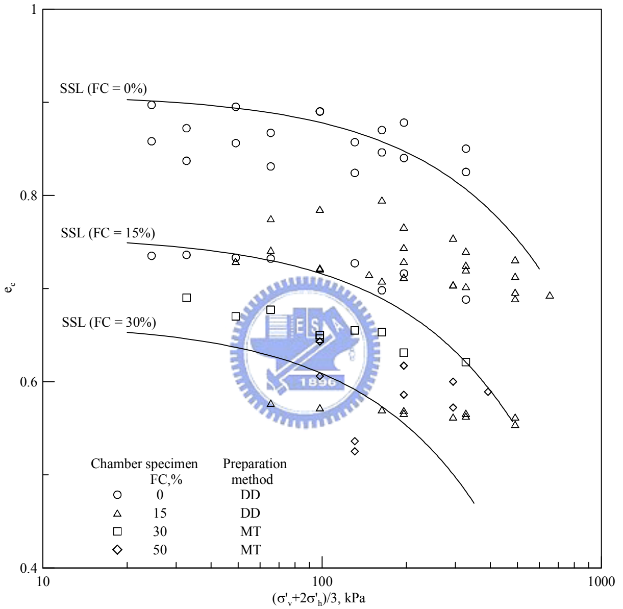
圖 3.2 CPT 試驗有效圍壓與壓密後孔隙比關係圖
