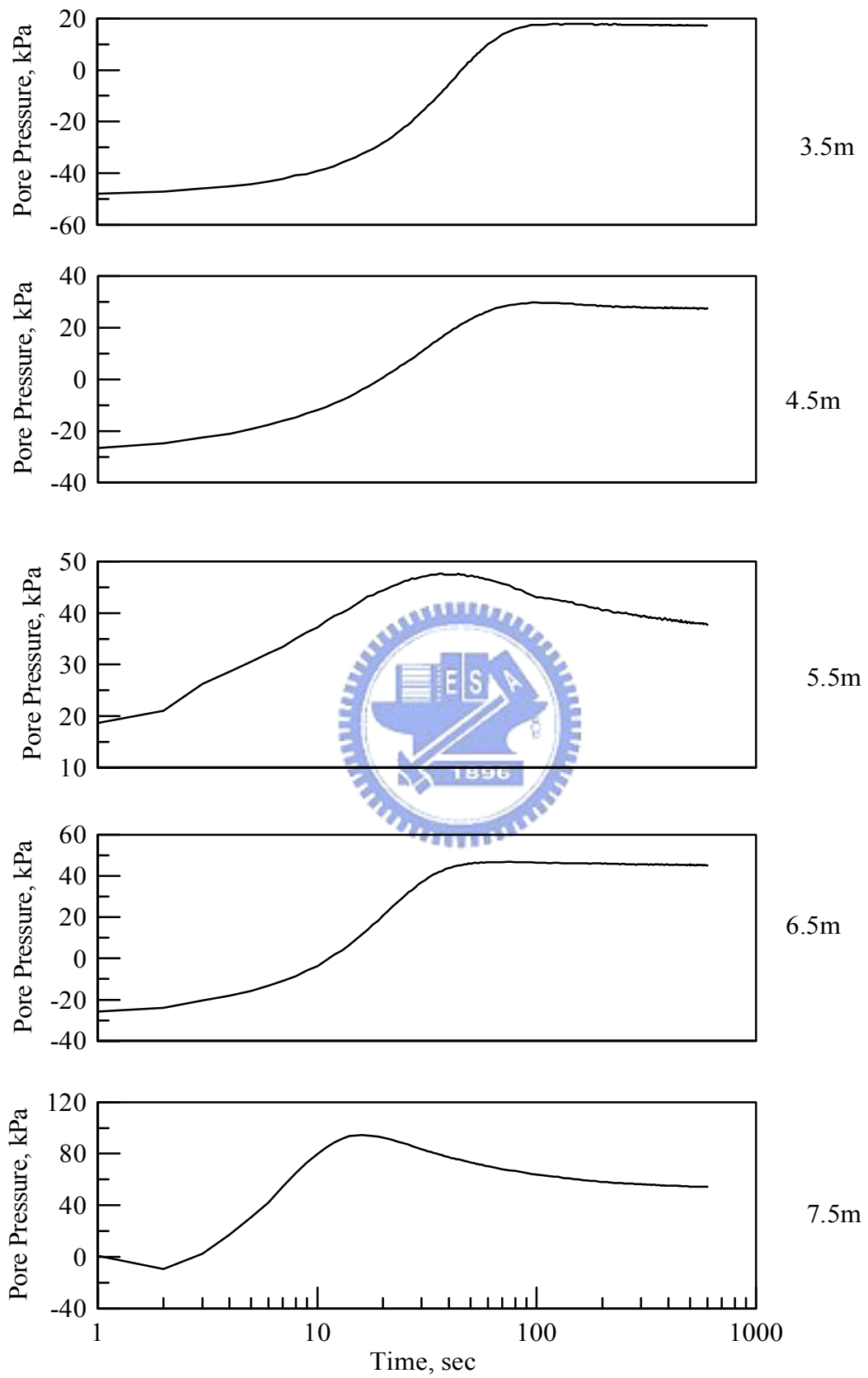
圖 5.16 員林場址 CPT 孔隙水壓消散試驗結果 (3.5m~7.5m)
