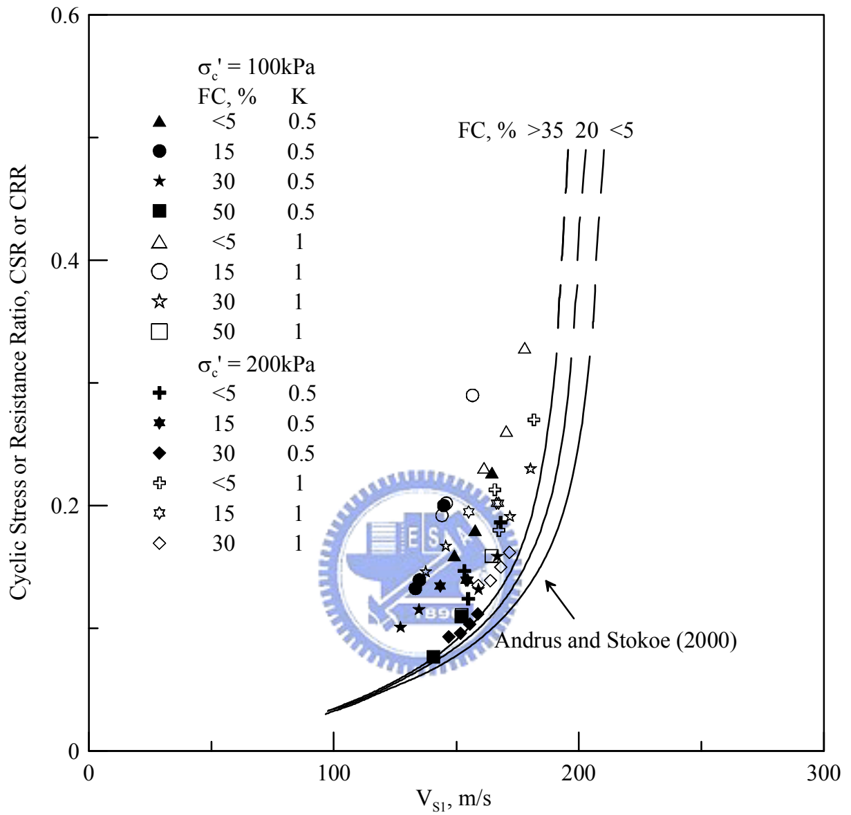
圖 4.21 麥寮砂之 CRR 與 V_{sl} 關係圖
