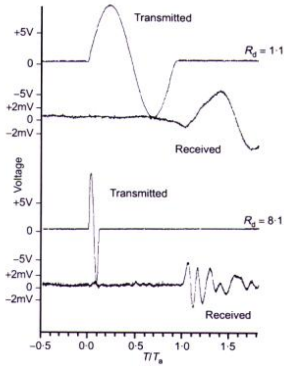
圖 2.7 不同 R_d 影響因子所致試驗結果 (Jovicic et al., 1996)
