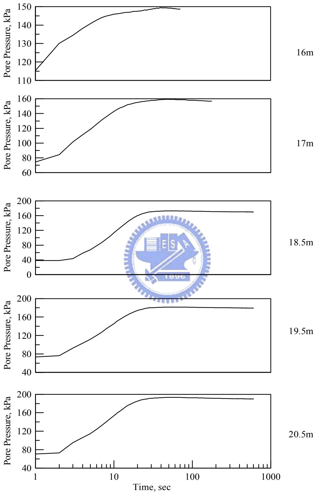
圖 5.19 高雄場址 CPT 孔隙水壓消散試驗結果 (16m~20.5m)
