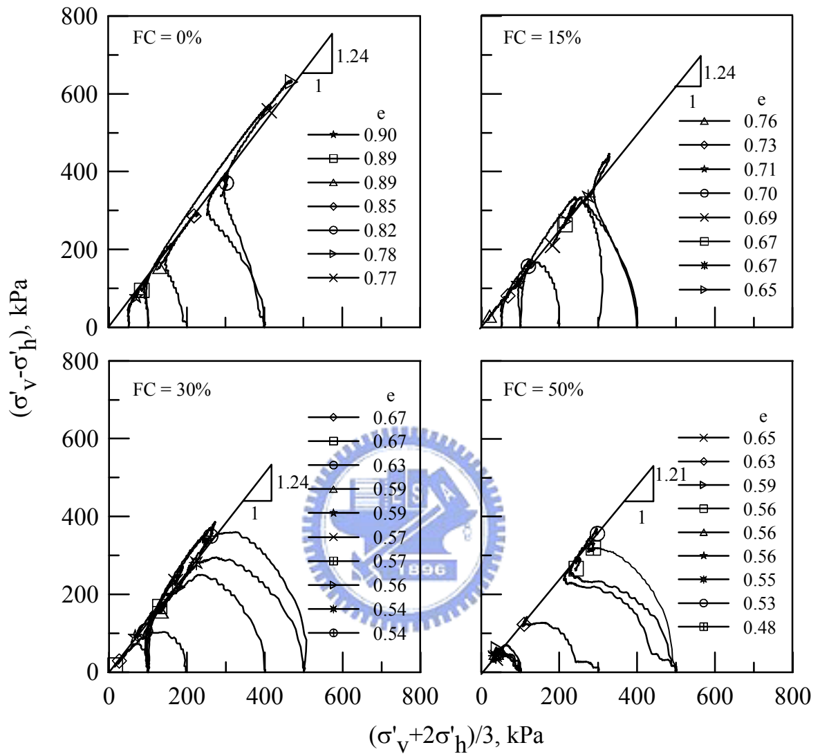
圖 2.17 麥寮砂三軸試驗有效應力路徑 (蔡明道, 2002)
