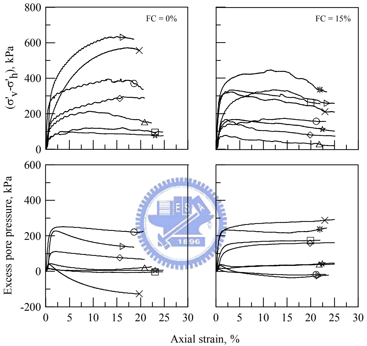
圖 2.15 麥寮砂 FC = 0 與 15% 三軸試驗應力、應變與超額孔隙水壓之相互關係 (蔡明道, 2002)
