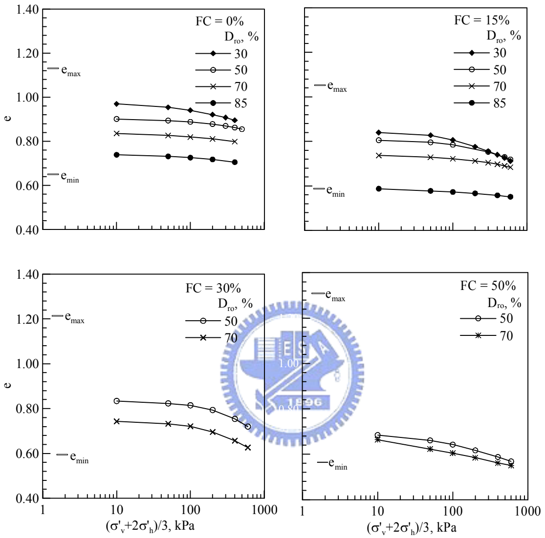
圖 2.14 麥寮砂之等向壓密曲線 (蔡明道, 2002)
