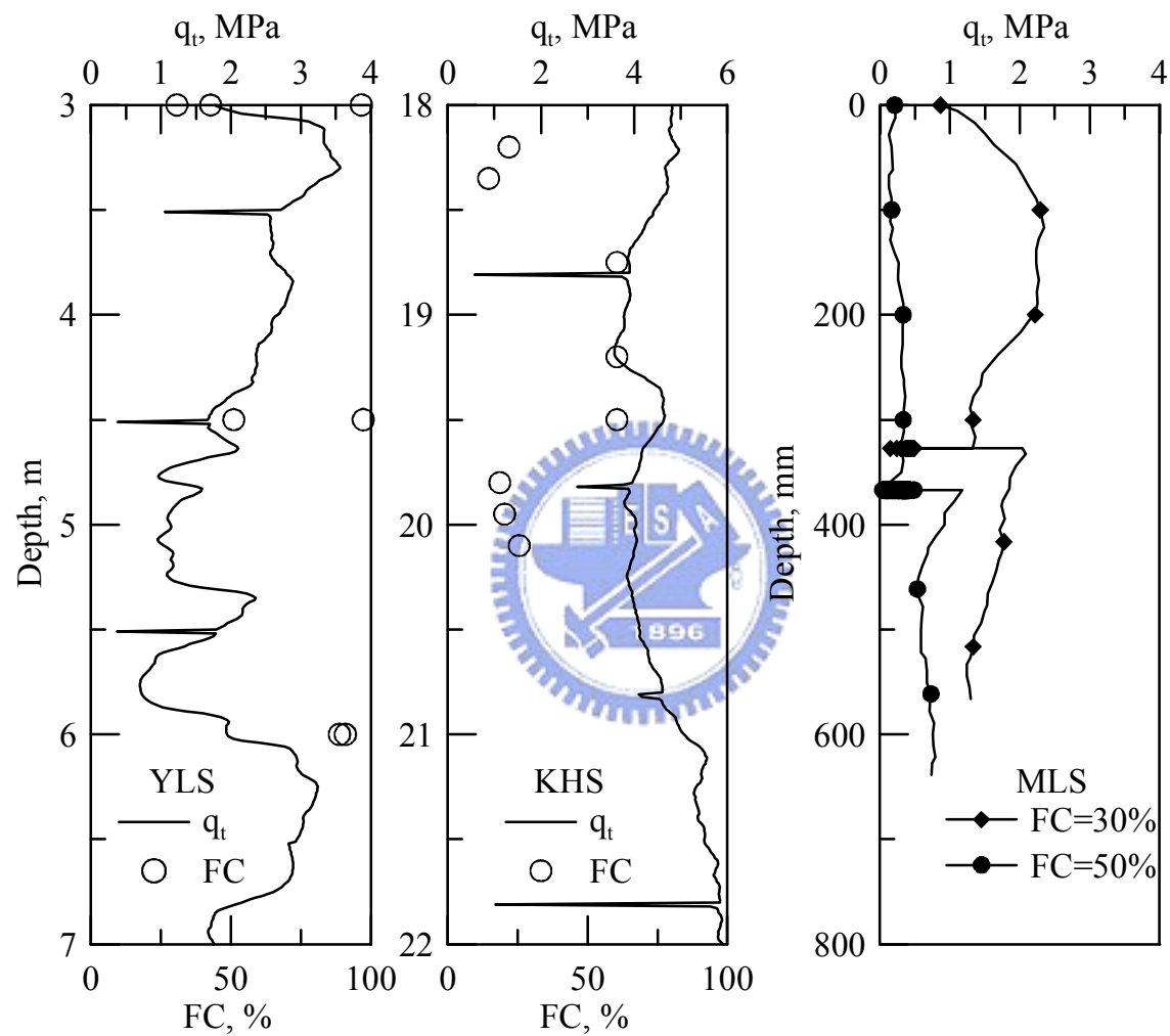
圖 5.15 現地試驗與室內標定試驗 q_t 比較
