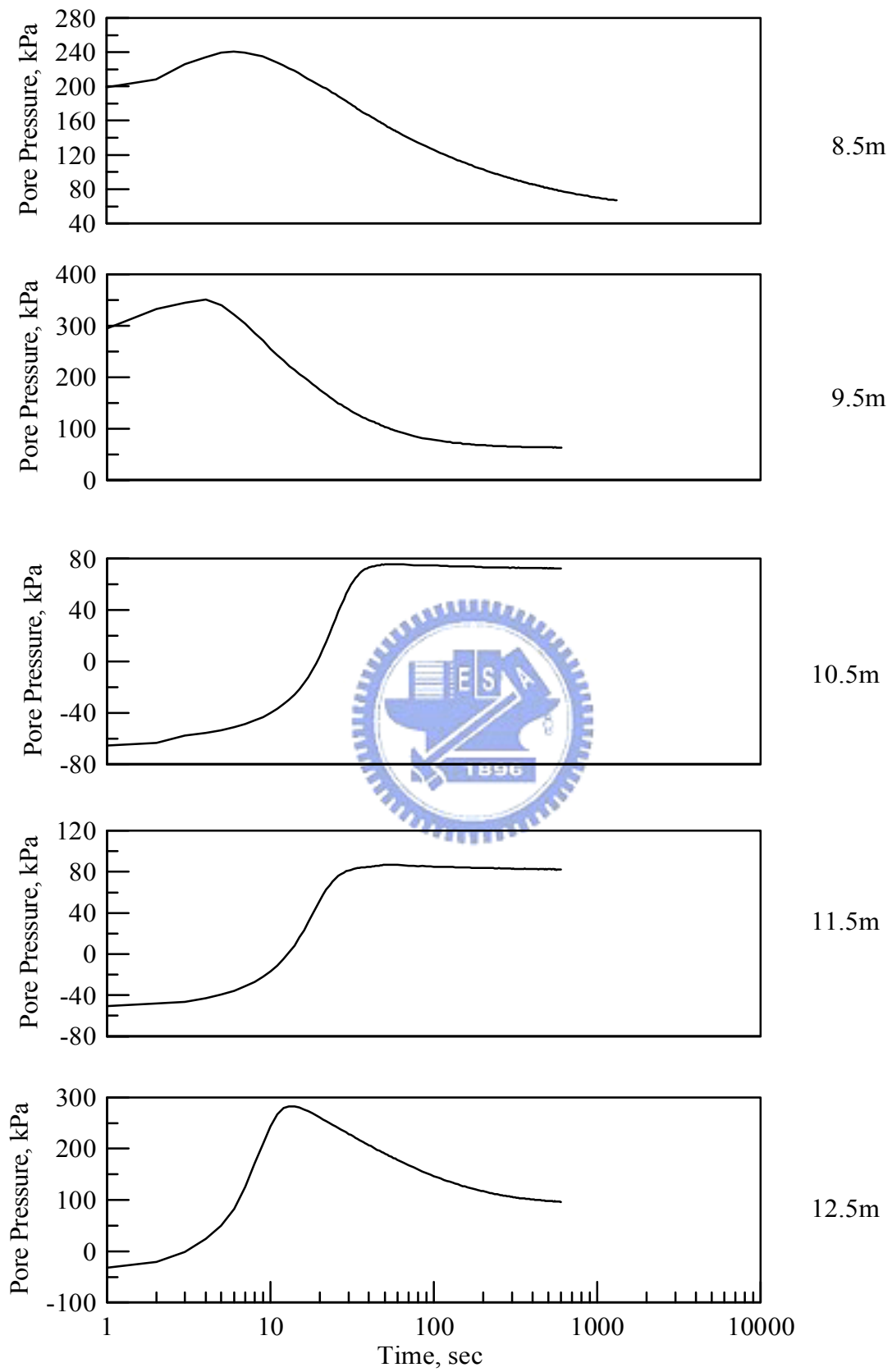
圖 5.17 員林場址 CPT 孔隙水壓消散試驗結果 (8.5m~12.5m)
