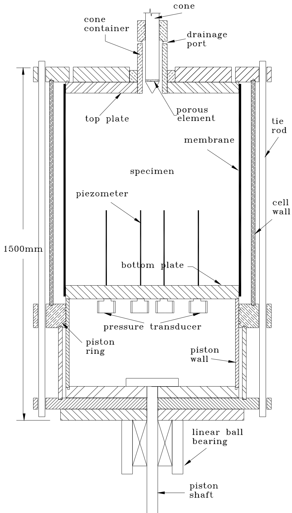
圖 2.19 可飽和試體之標定槽概念圖 (Huang et al., 1991)
