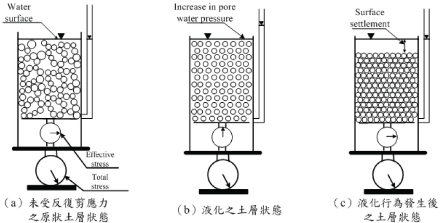
圖 2.1 液化示意圖 (Ishihara, 1985)
