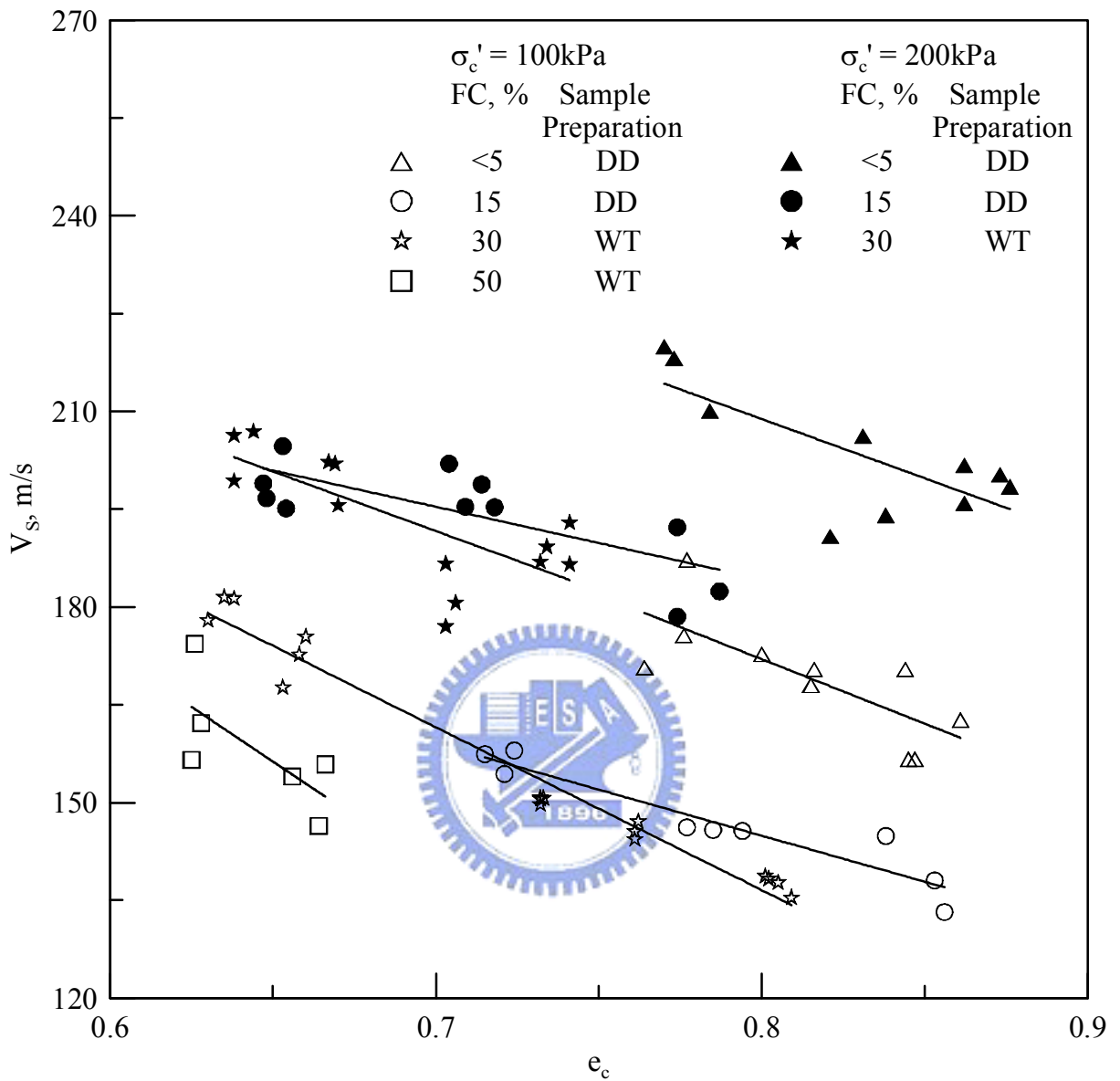
圖 4.14 麥寮砂剪力波速量測結果
