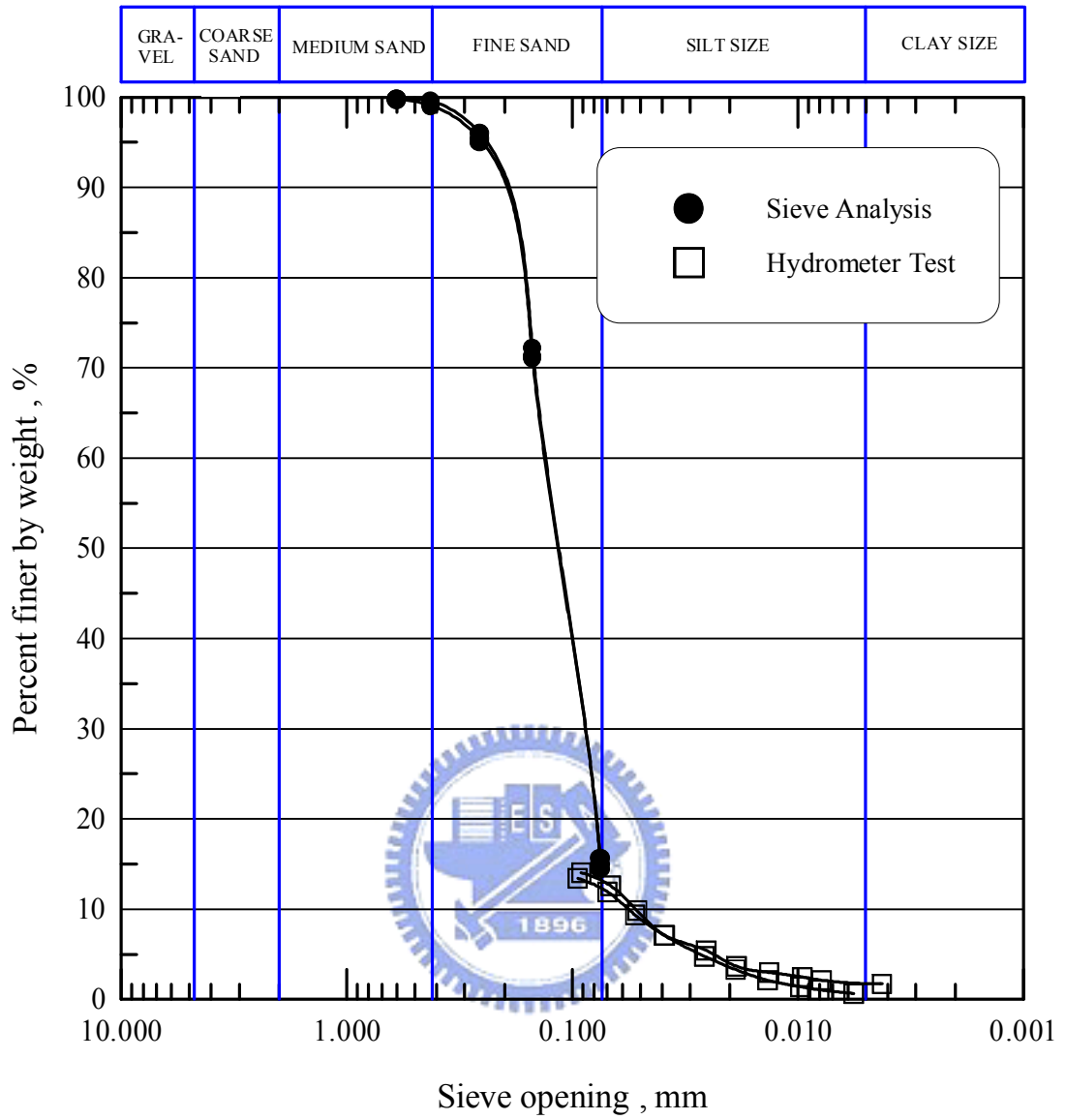
圖 2.10 麥寮砂之粒徑分布曲線 (張嘉偉, 1997)
