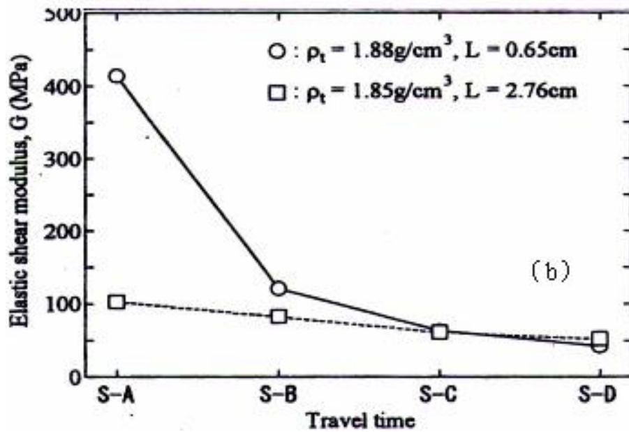
圖 2.9 不同時間到達點下試體長度對剪力模數 (G) 的影響 (Kawaguchi et al., 2001)
