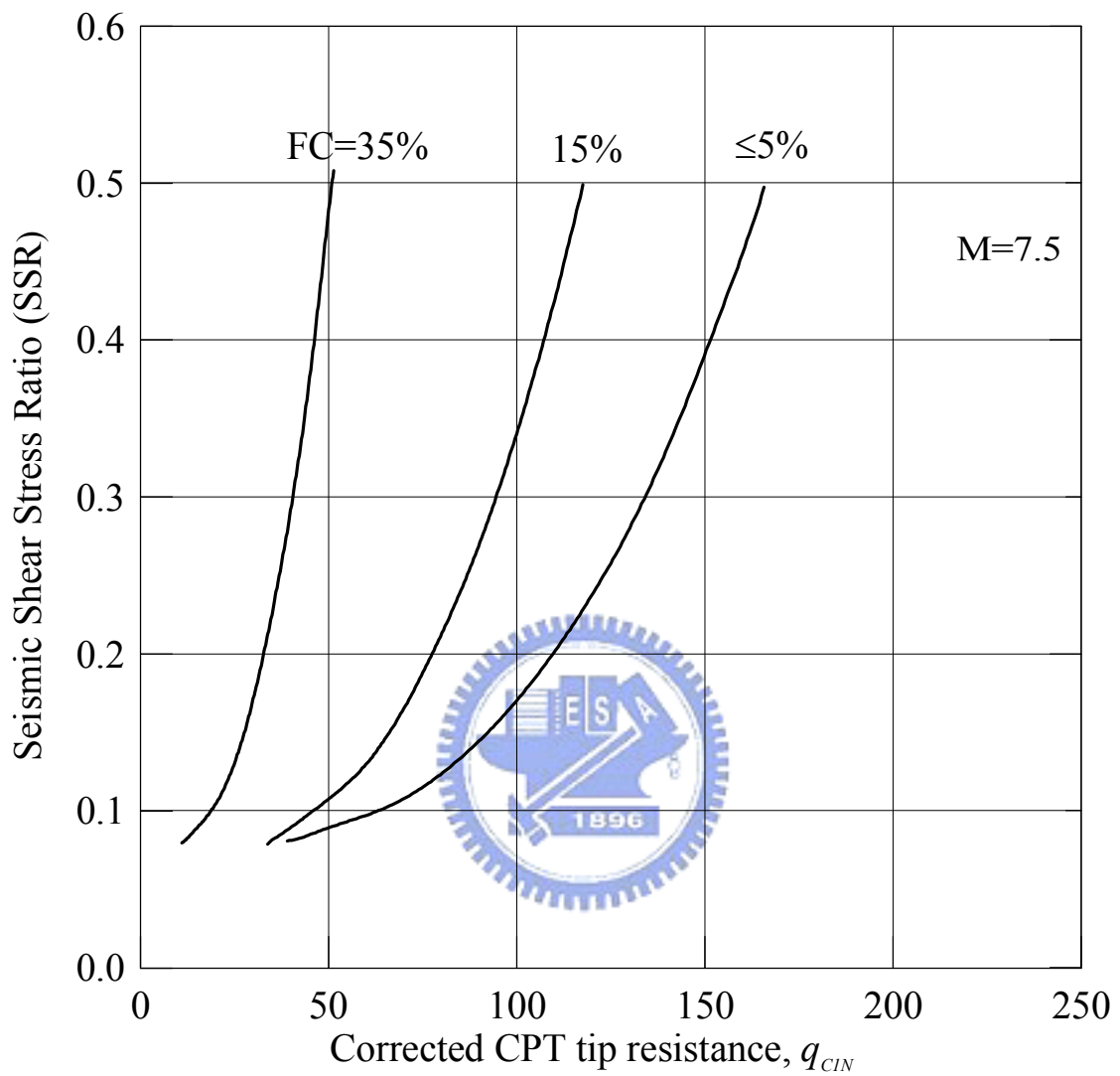
圖 2.2 不同細料含量之液化潛能臨界曲線圖 (Stark and Olson, 1995)
