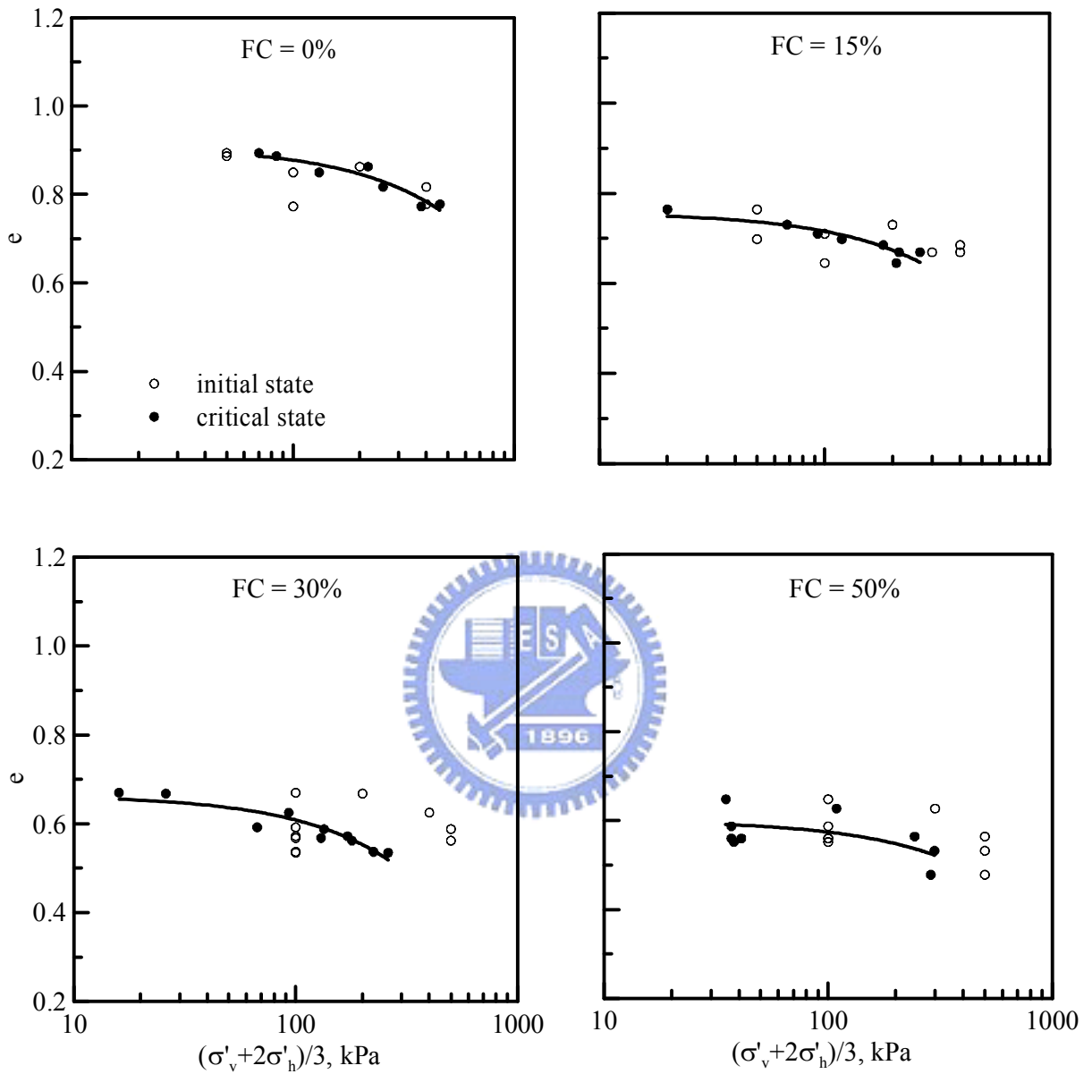
圖 2.18 麥寮砂三軸試驗之臨界狀態 (蔡明道, 2002)
