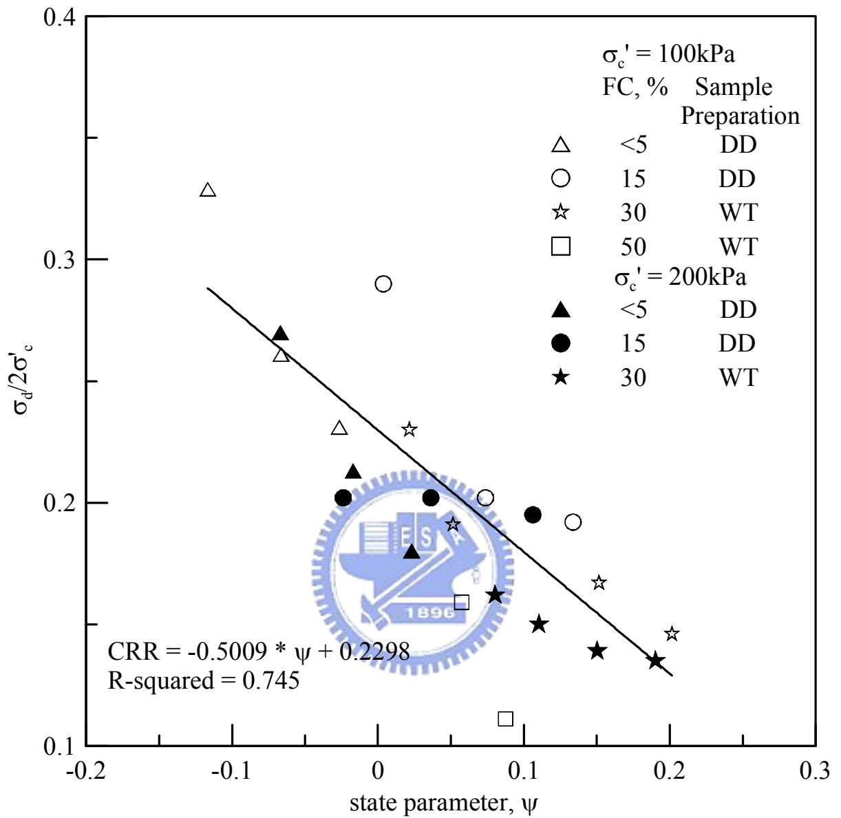
圖 4.7 麥寮砂 CRR 與狀態參數之關係 (K=1)
