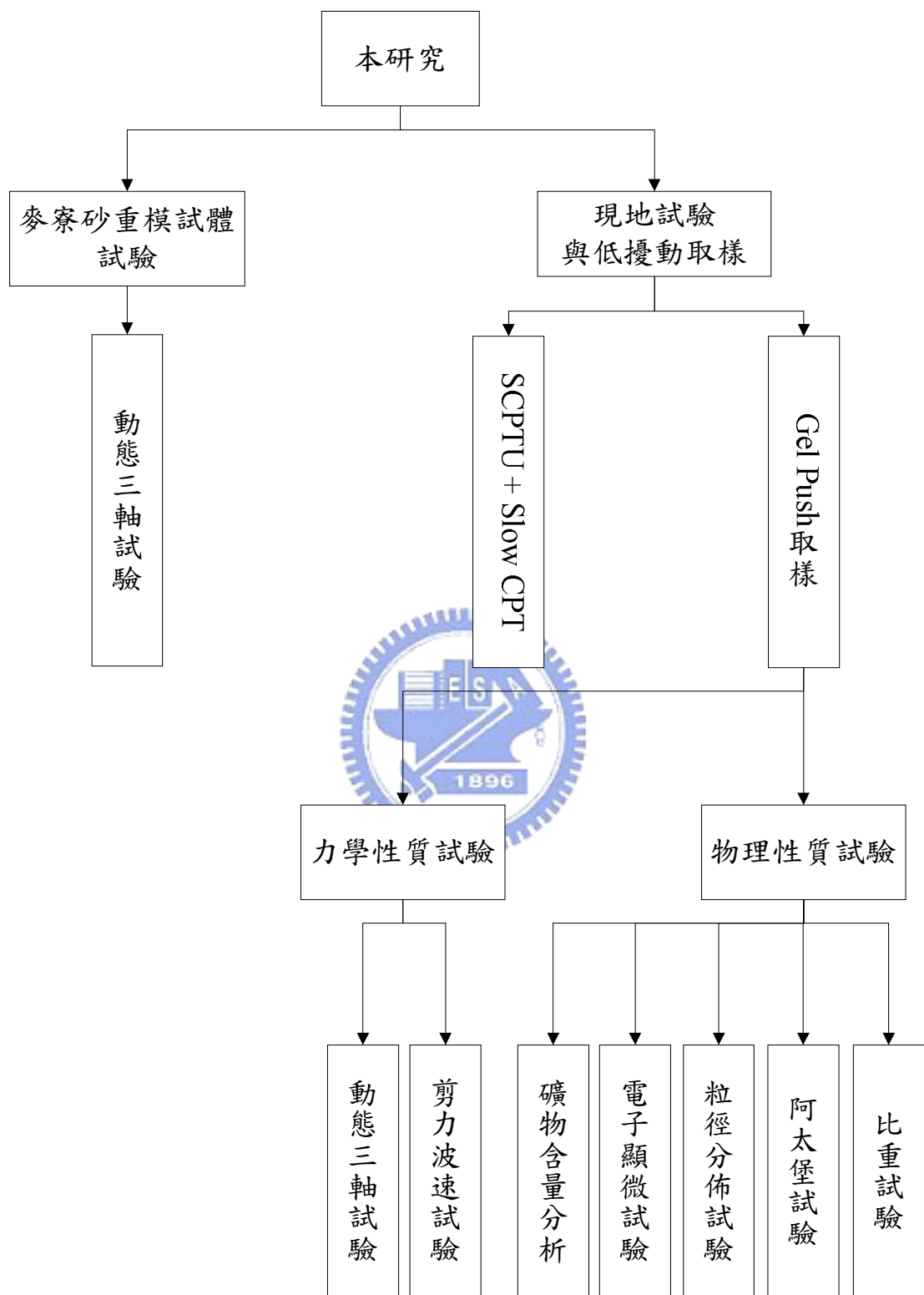
圖 3.1 試驗流程圖
