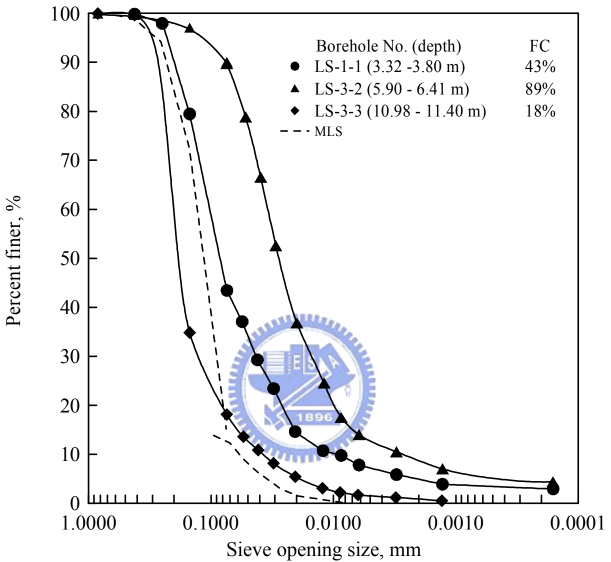
圖 5.1 員林砂 LS 試體之粒徑分布曲線 (黃耀道, 2007)
