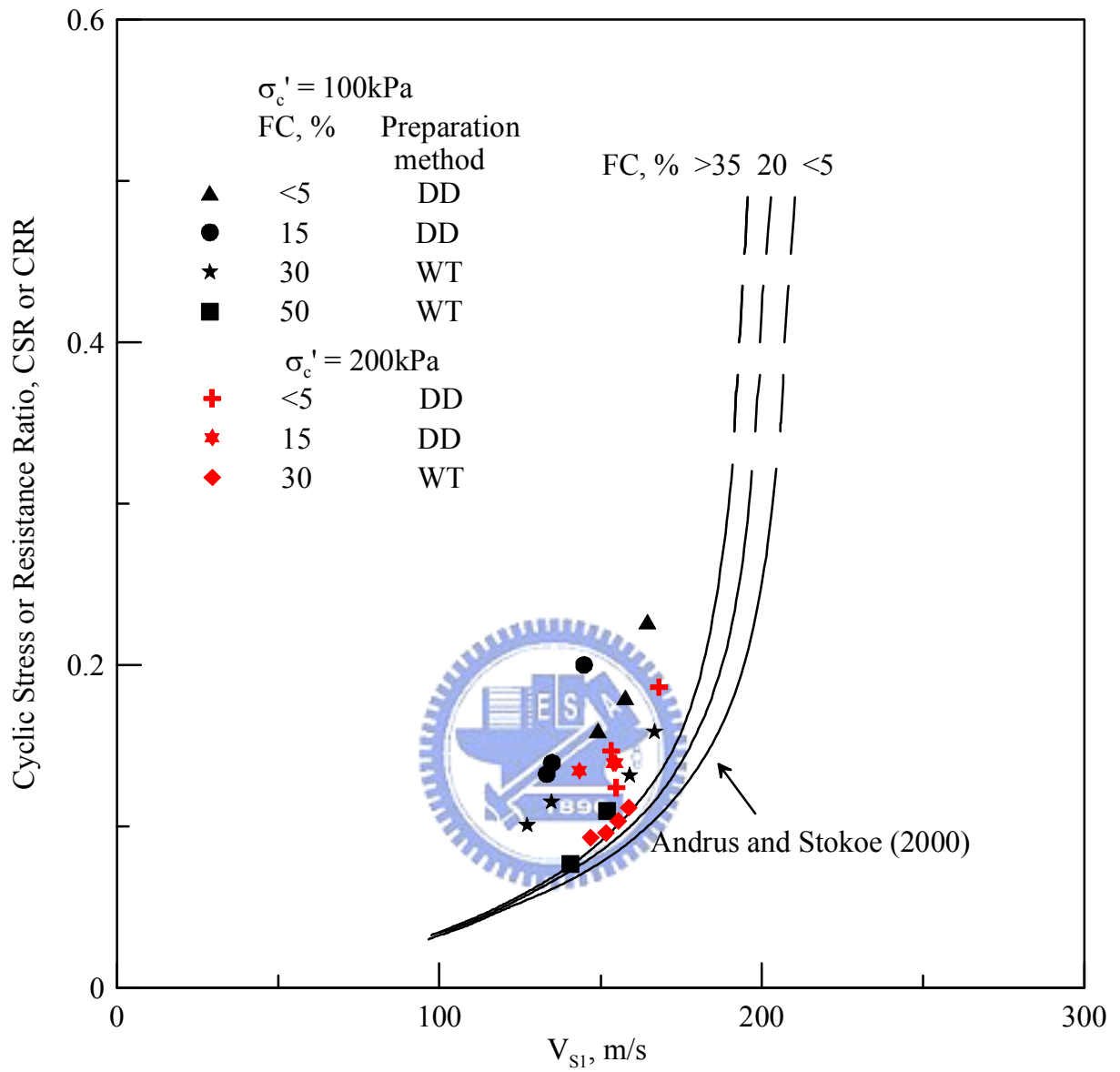
圖 4.22 Kawaguchi et al. (2001) C 點-CRR 與 V_{sl} 之關係
