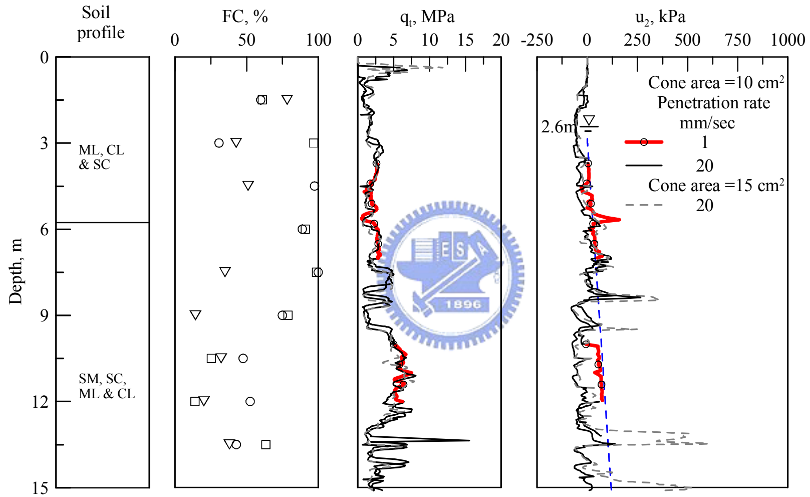
圖 5.22 員林場址慢速 CPT 試驗與標準 CPT 試驗結果
