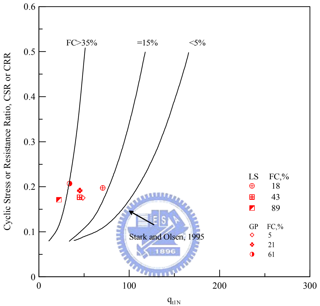
圖 5.25 低擾動試體與 Stark and Olsen 液化臨界線比較
