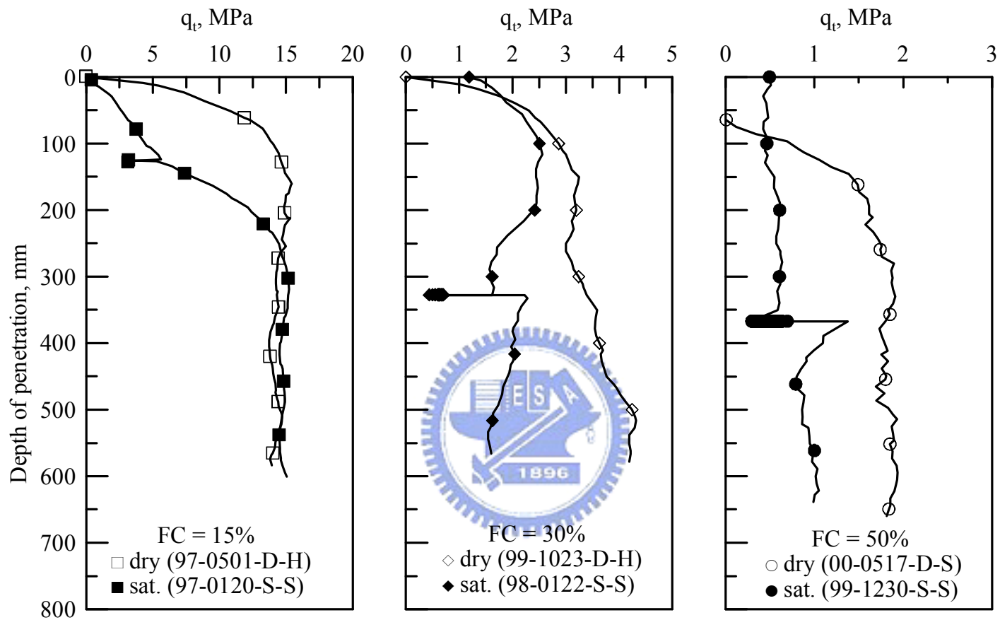
圖 2.21 乾燥與飽和試體 CPT 試驗結果之比較
