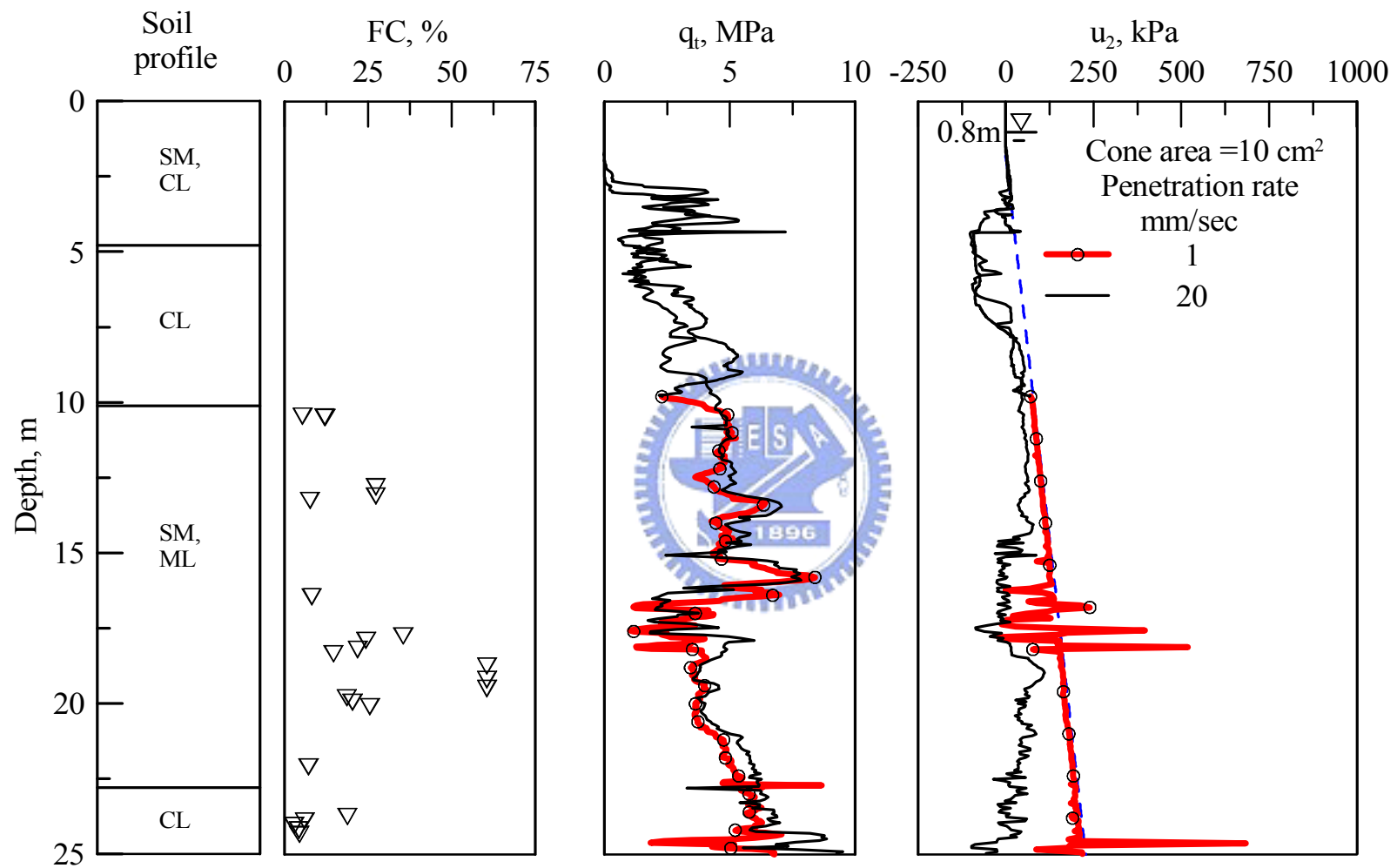
圖 5.23 高雄場址慢速 CPT 試驗與標準 CPT 試驗結果
