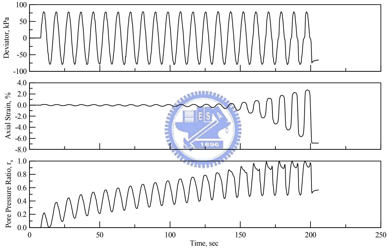
圖 4.1 時間對軸差應力、軸向應變、超額孔隙水壓比關係圖
