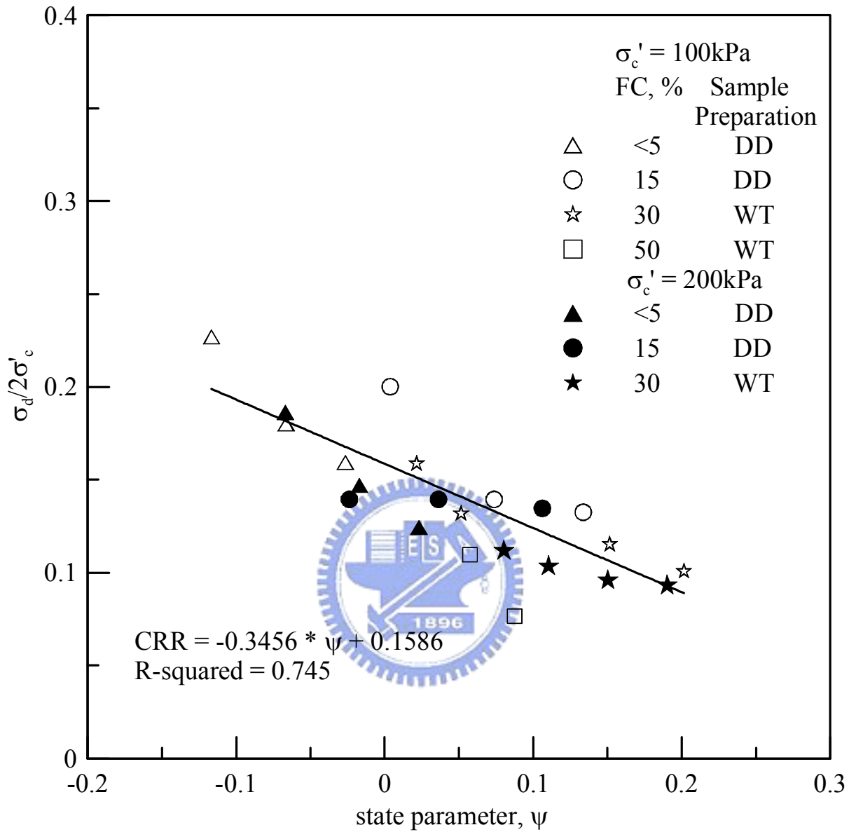
圖 4.8 麥寮砂 CRR 與狀態參數之關係 (K=0.5)
