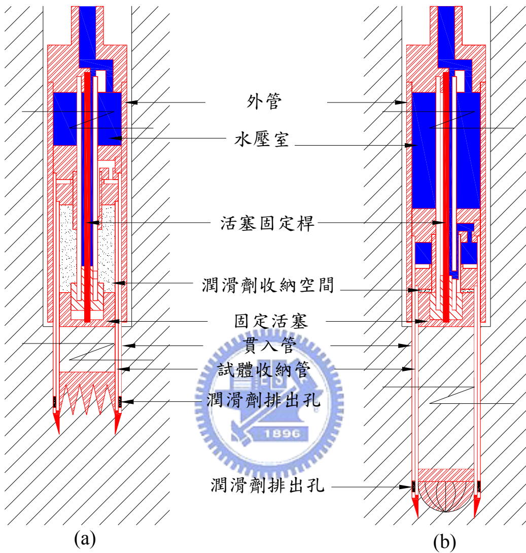
圖 3.11 Gel Push 活塞取樣器示意圖 (李維峰等人, 2006)
