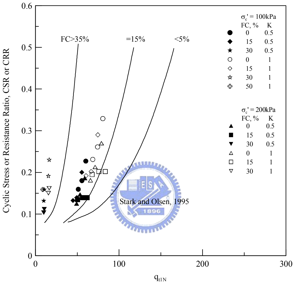
圖 4.11 麥寮砂 CRR- q_{t1N} 與 Stark and Olson 法之比較
