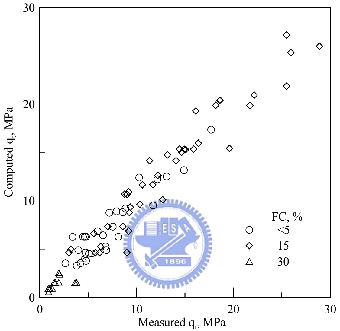
圖 2.23 試驗數據與經驗公式之對比
