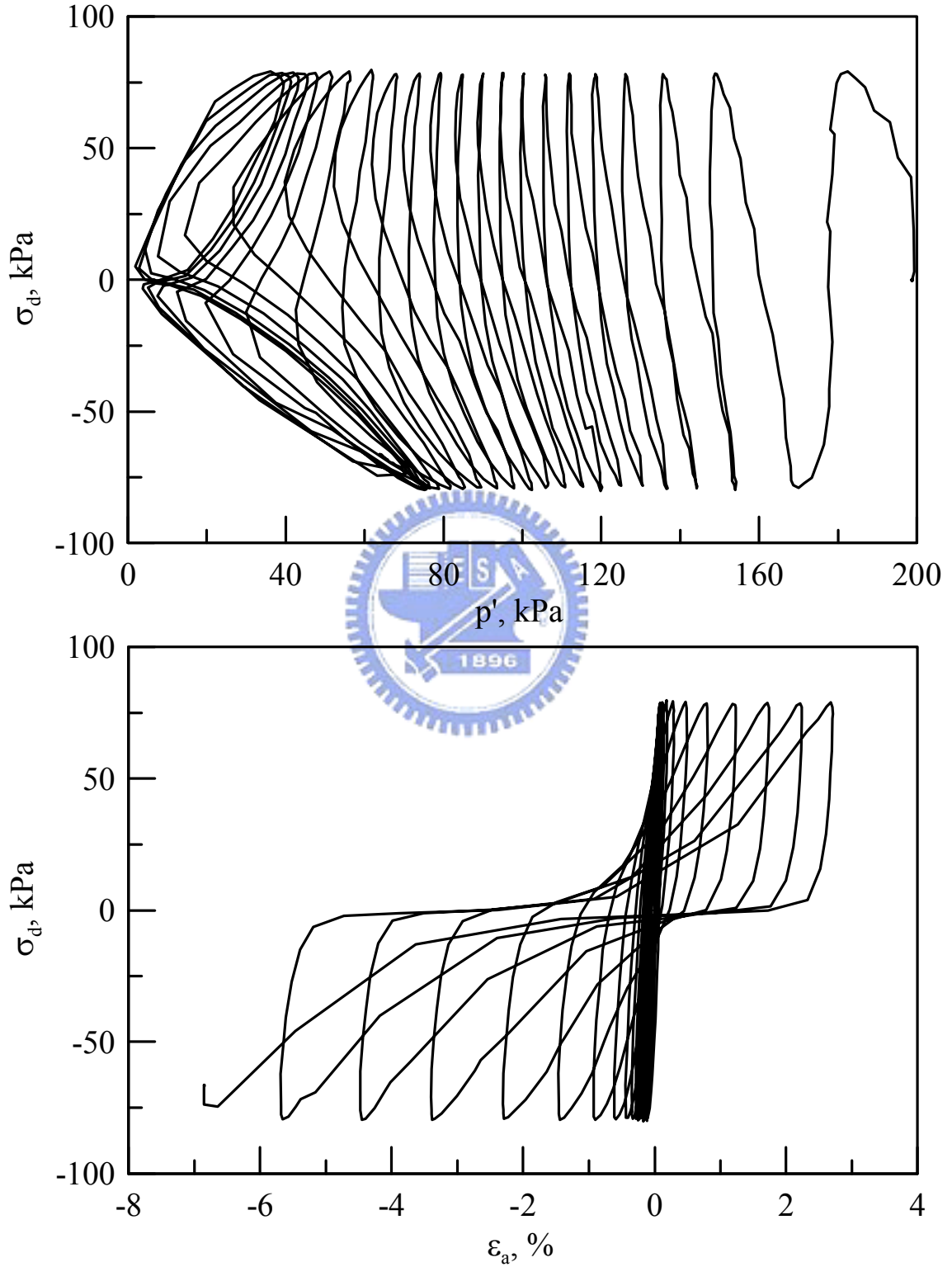
圖 4.2 p' 與軸差應力、軸向應變與軸差應力關係圖
