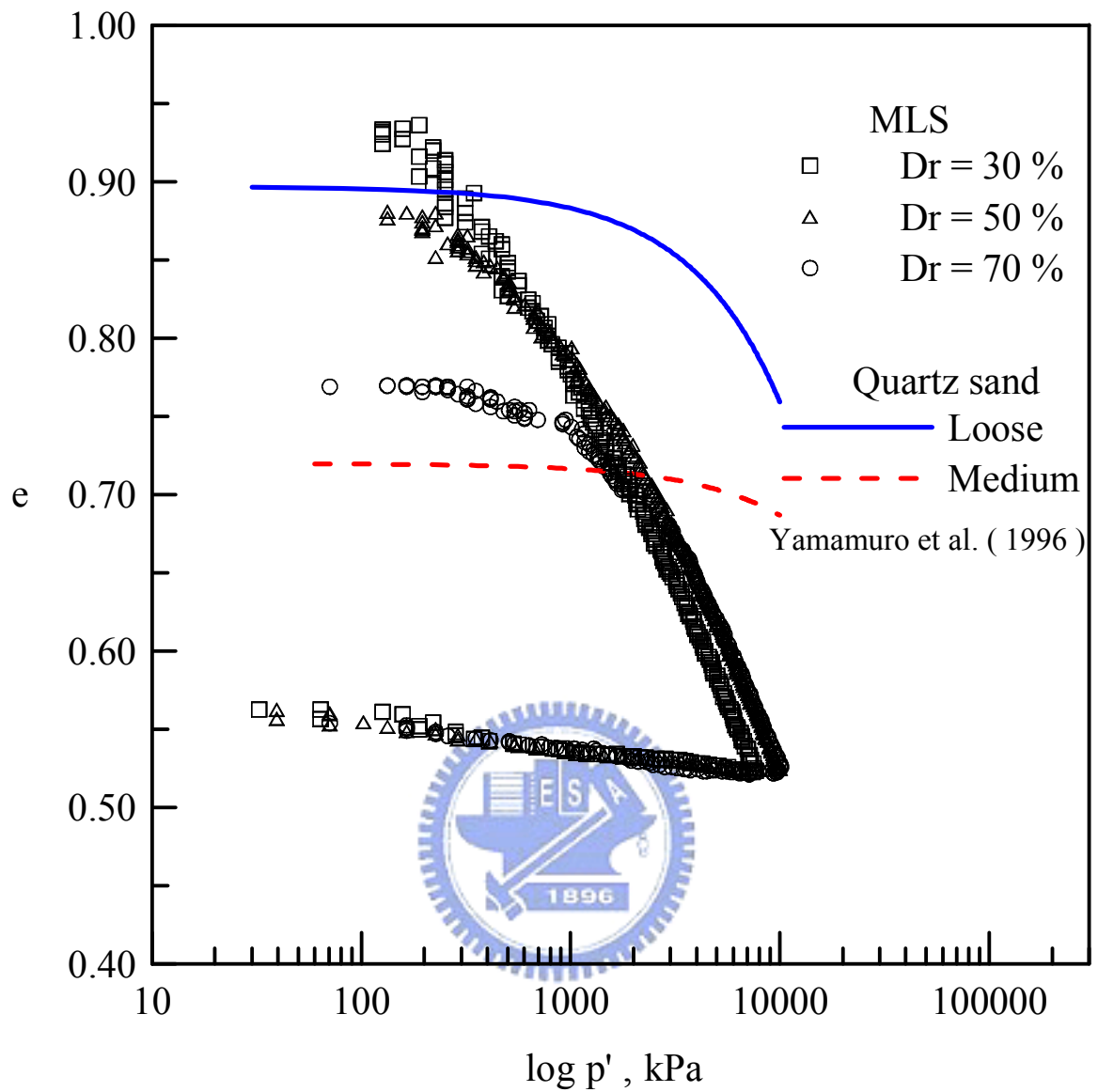
圖 2.13 單向度壓縮曲線 (張嘉偉, 1997)
