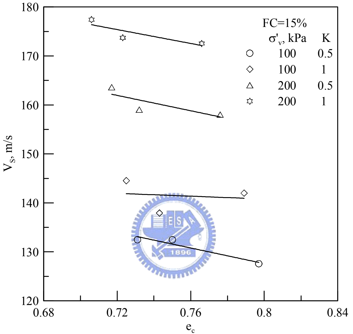
圖 4.15 FC=15%剪力波速與孔隙比在不同應力條件之關係
