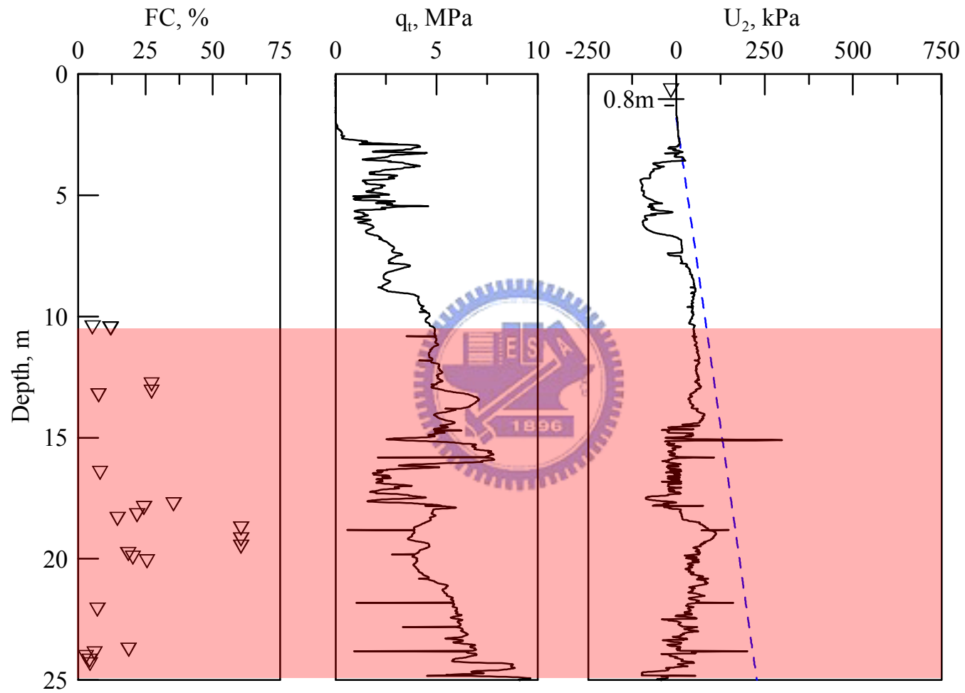
圖 5.14 高雄場址 CPT 試驗結果
