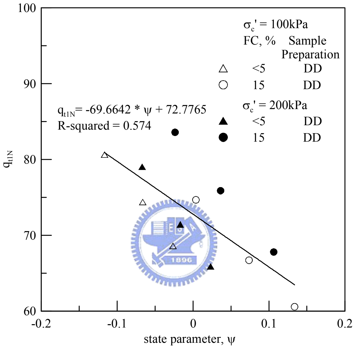
圖 4.9 排水行為下麥寮砂 q_{tIN} 與狀態參數之關係 (K=1)
