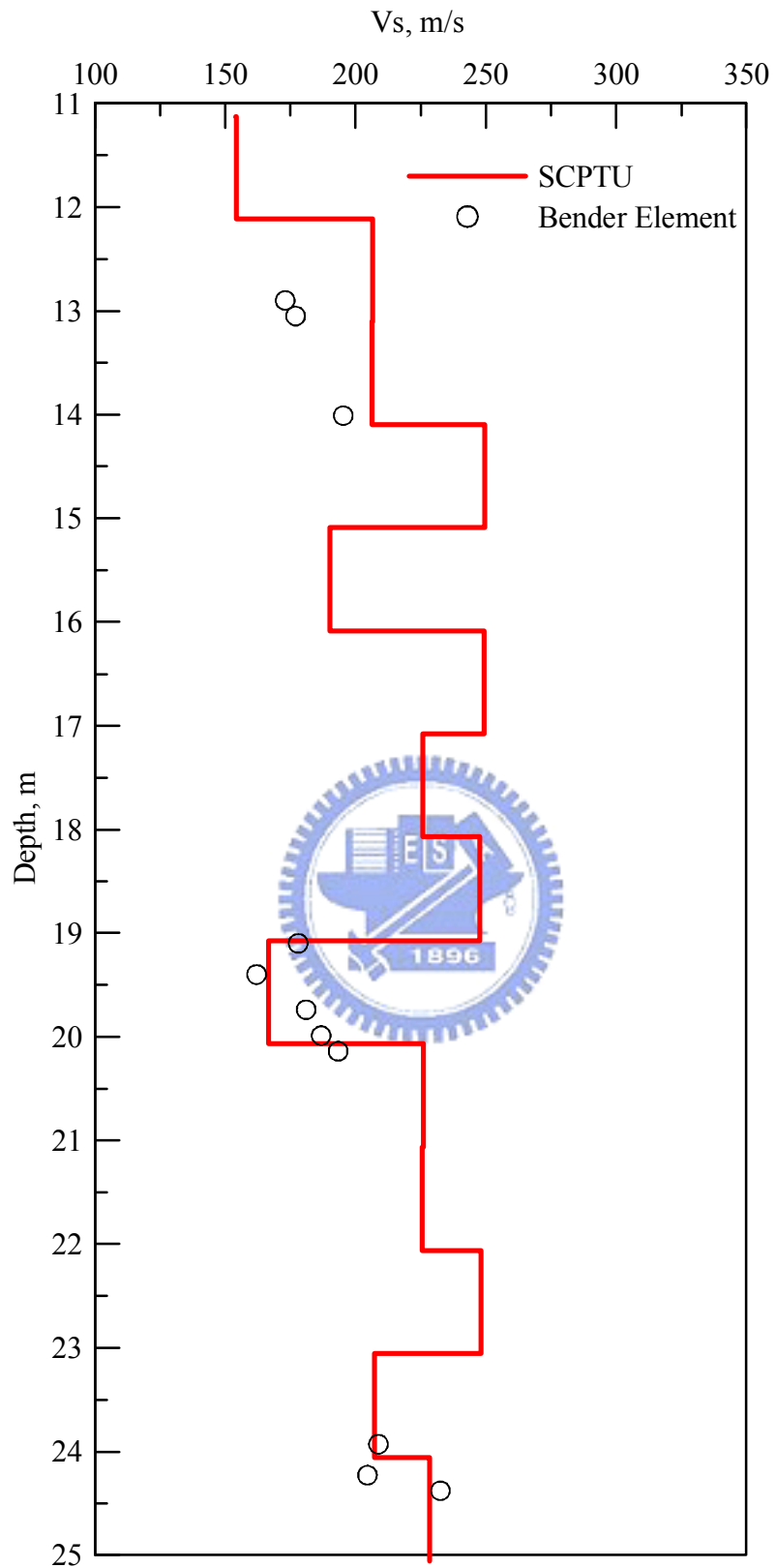
圖 5.12 現地 SCPTU 與動態三軸試體剪力波速比較
