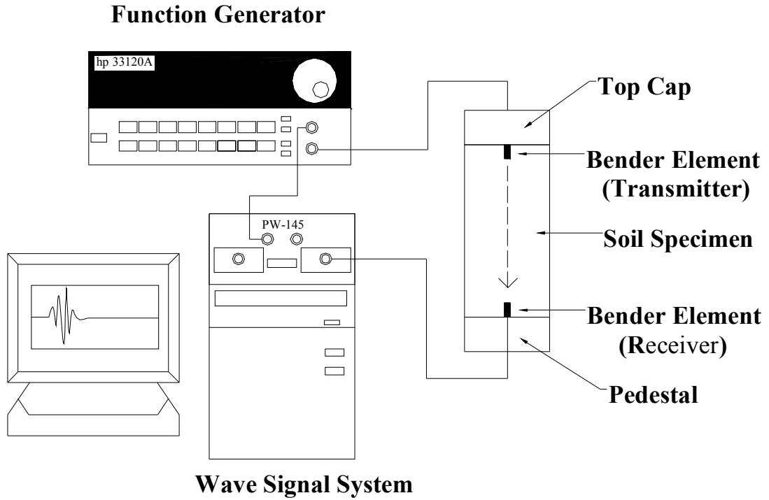
圖 2.5 剪力波量測試驗示意圖 (林靜怡, 2003)
