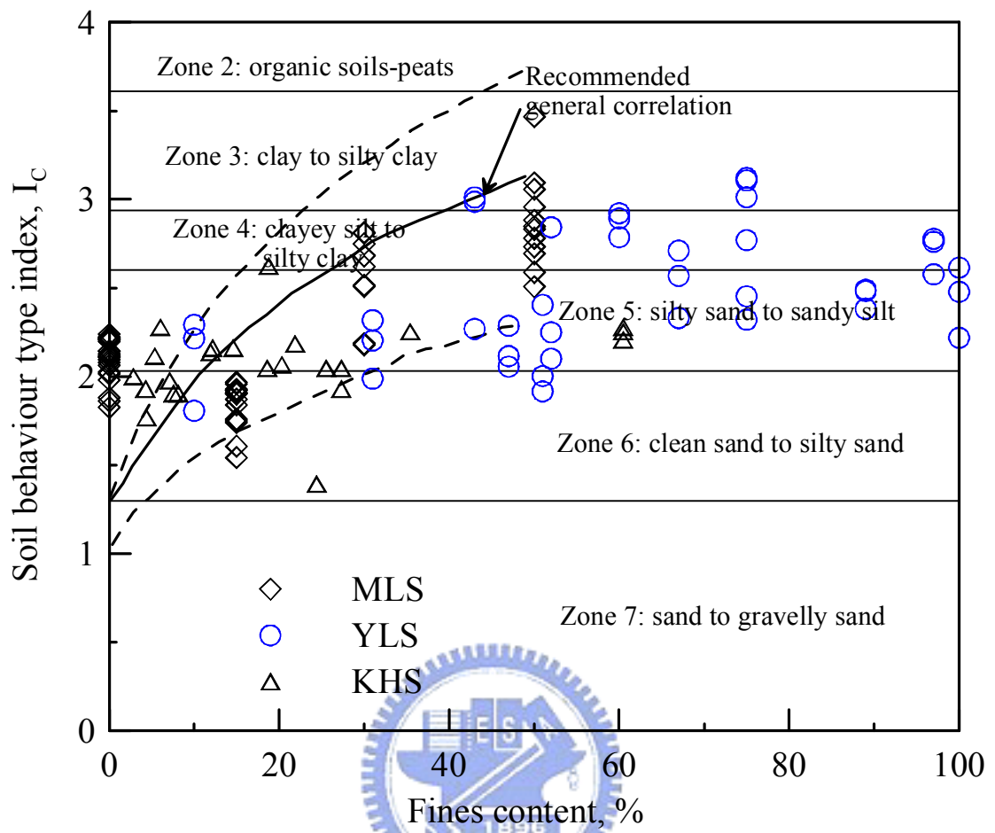
圖 5.24 麥寮砂、員林砂與高雄砂 I_c 與細料含量之關係
