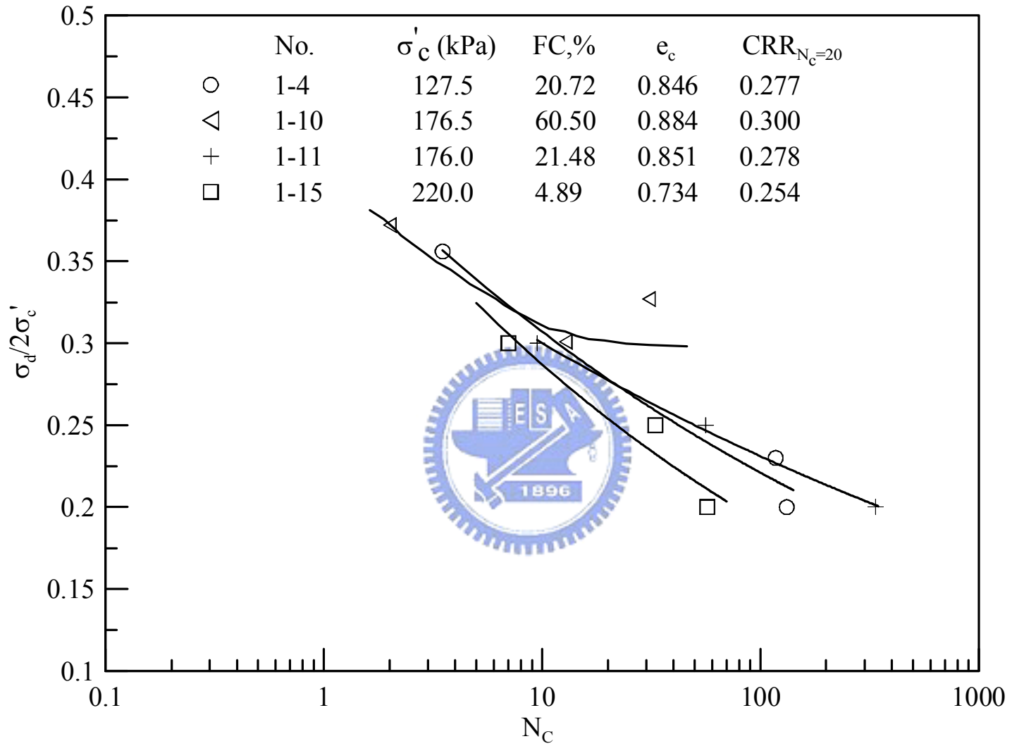
圖 5.11 動態三軸試驗結果
