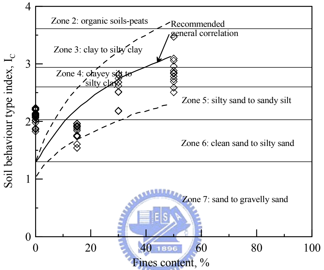
圖 2.25 麥寮砂之 I_c 與細料含量關係
