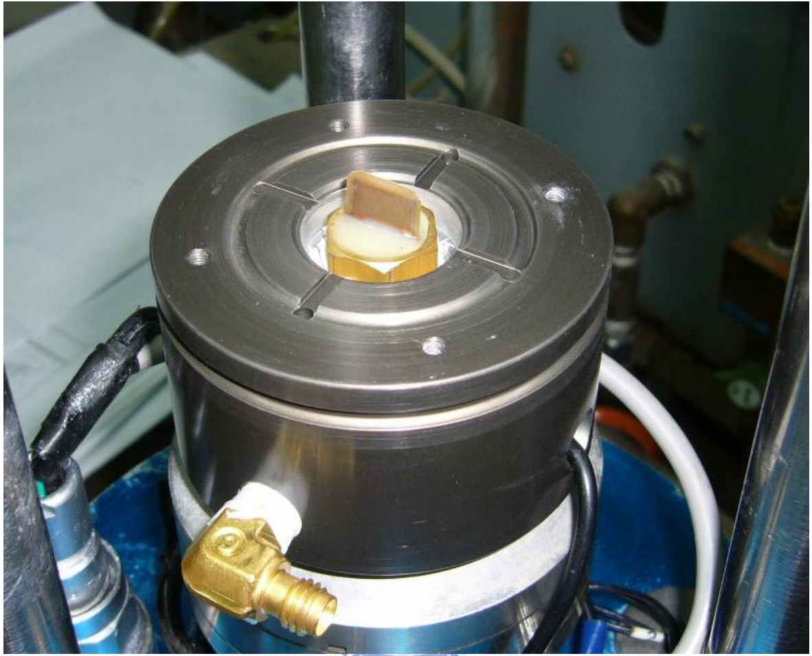
圖 3.8 激發端剪力波元件設備
