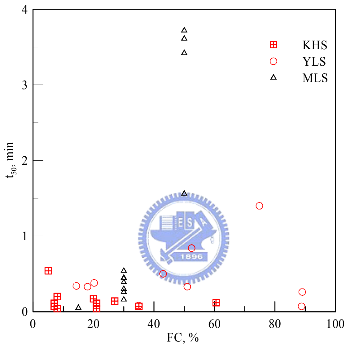
圖 5.21 細料含量與 t 50 之關係
