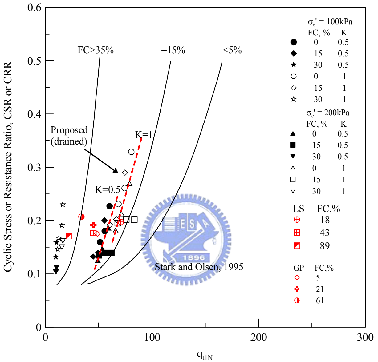
圖 5.26 台灣西南部粉土質細砂排水行為下液化臨界線
