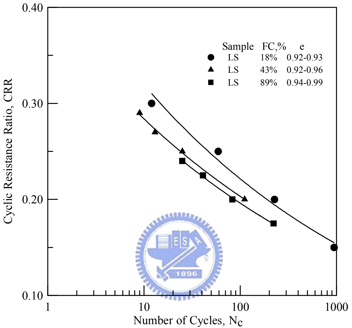
圖 5.3 員林砂非擾動試體動態三軸試驗結果 (修改自黃耀道, 2007)
