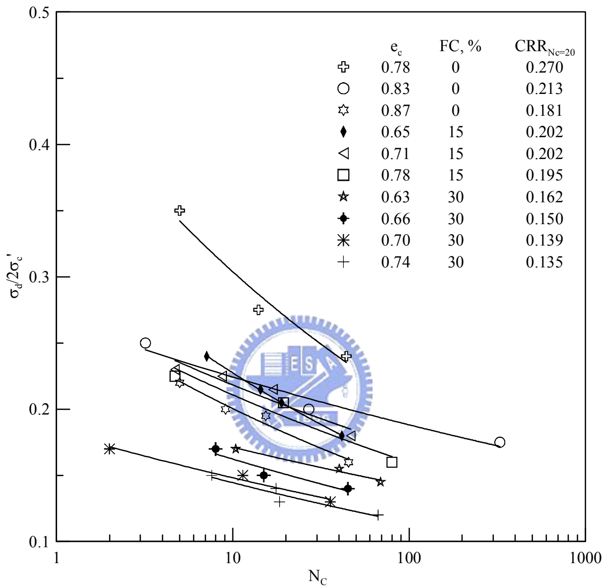
圖 4.5 動態三軸試驗結果 ( \sigma'_c=200\text{kPa} )
