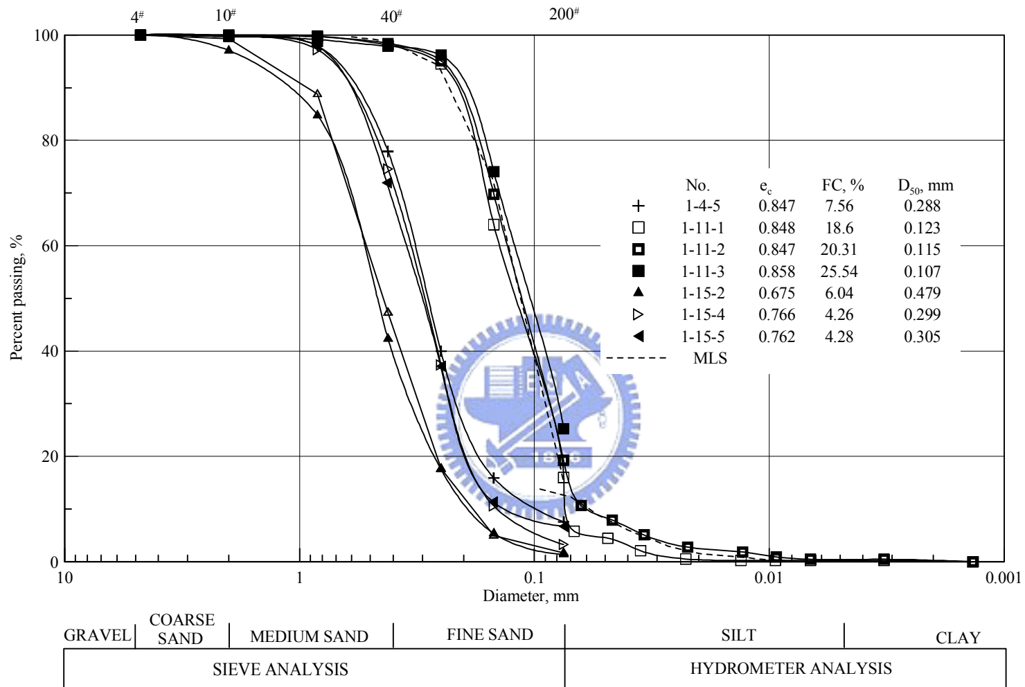
圖 5.9 高雄砂動態三軸試驗粒徑分佈曲線
