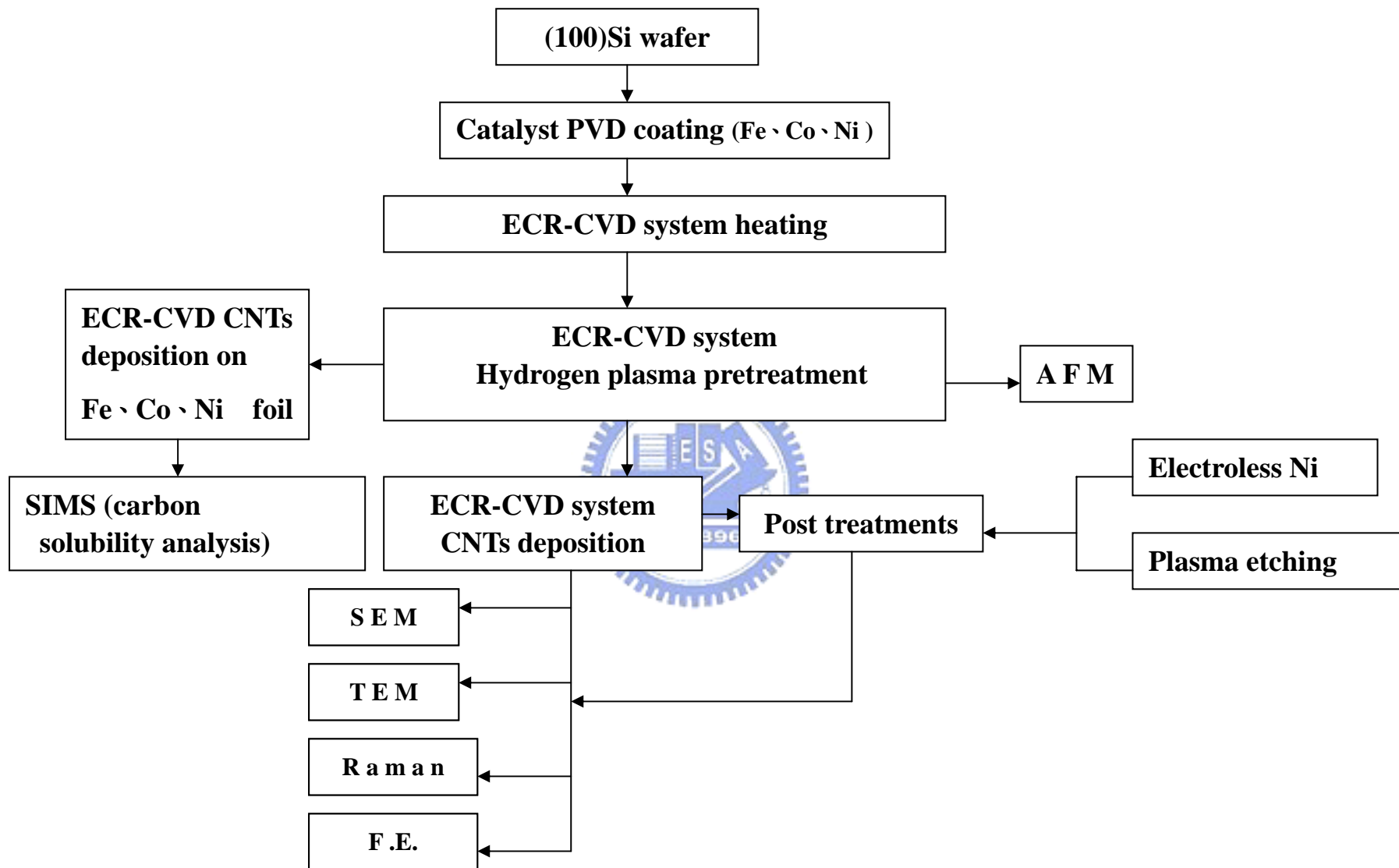
圖 3.3 實驗流程圖
