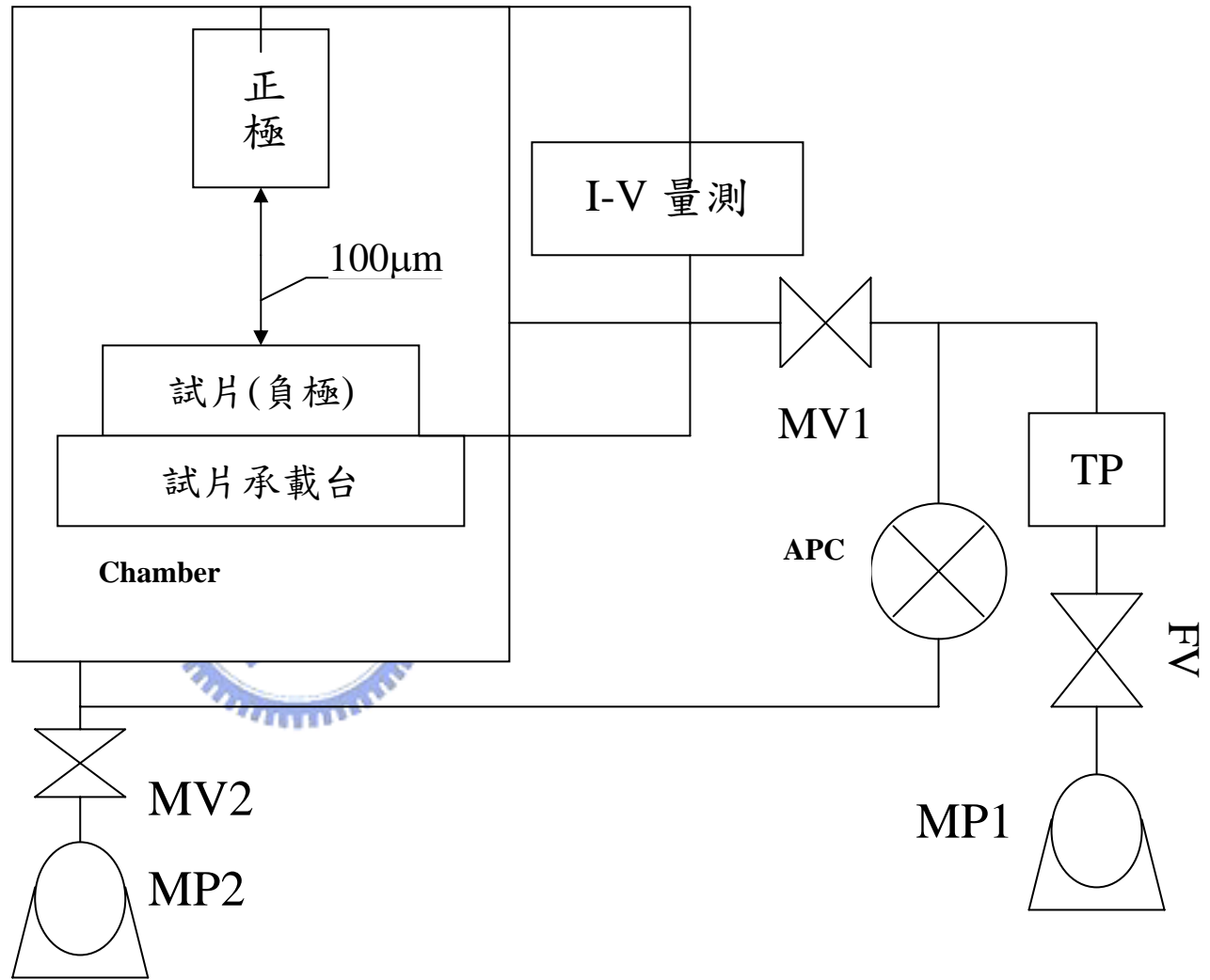
圖 3-4. 場發射量測系統[由張惠林提供]
