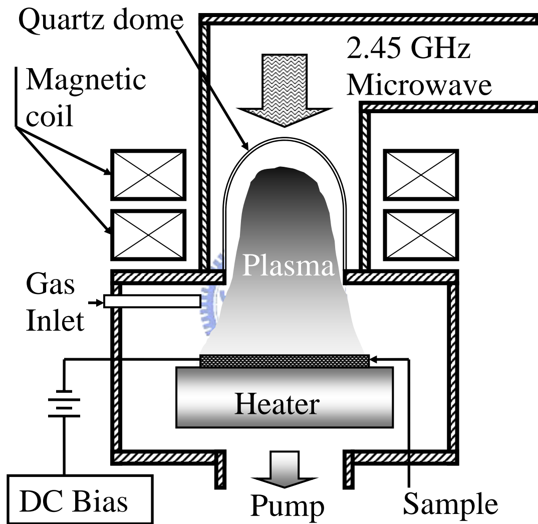
圖 3.1 ECR-CVD 系統[由林兆焄提供]
