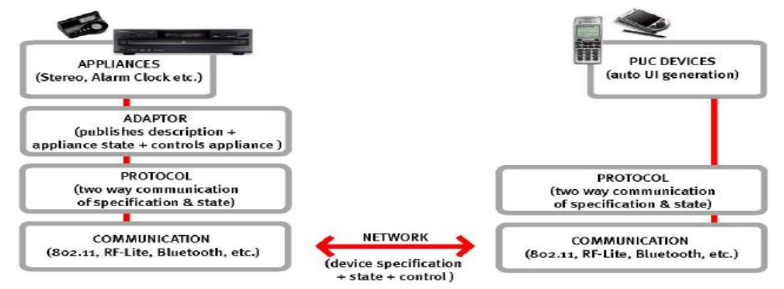
圖 11、PUC System Architectural Diagram
