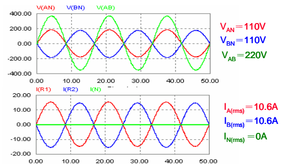
圖 7 平衡負載輸出電壓模擬圖
