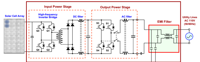
圖 5 高頻隔離式雙級全橋式併網型變頻器
