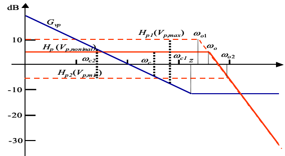
圖 15 輸出級變流器的迴路增益設計
