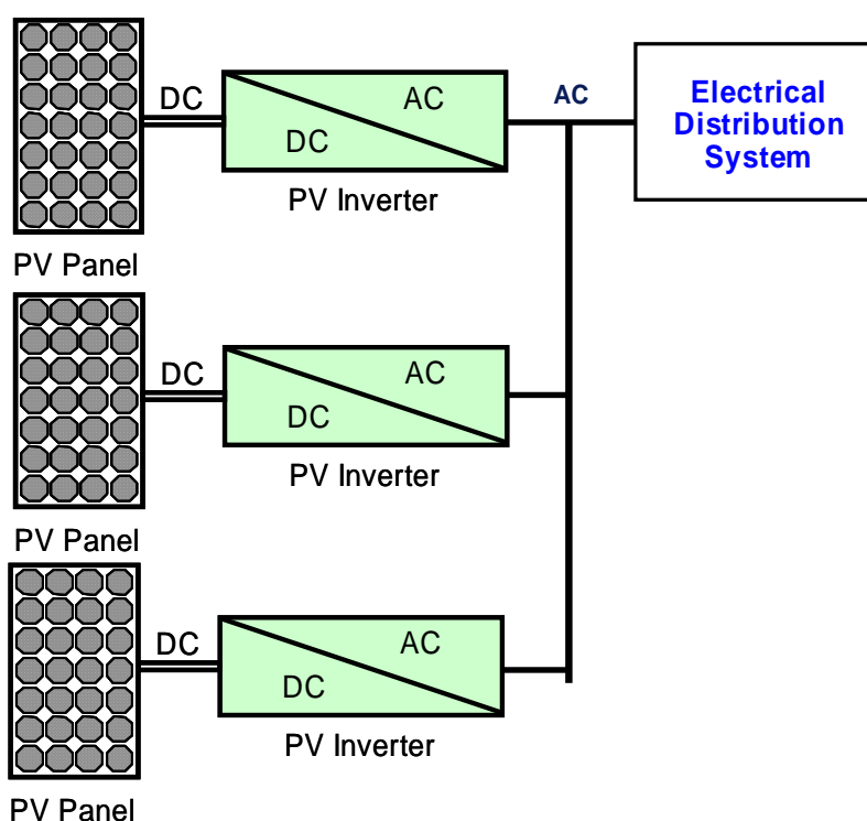
圖 1.1 太陽能發電系統的系統架構圖
