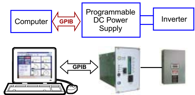
圖 8 太陽光模組模擬器的系統方塊圖
