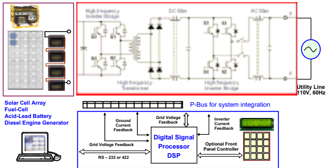
圖 17 雙級式併網型太陽光發電系統之系統架構圖
