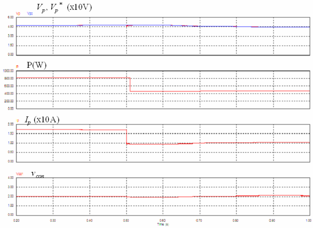
圖 4.10 日照量由 1KW/m^2 變化為 0.6KW/m^2 下 MPPT 控制之模擬結果
