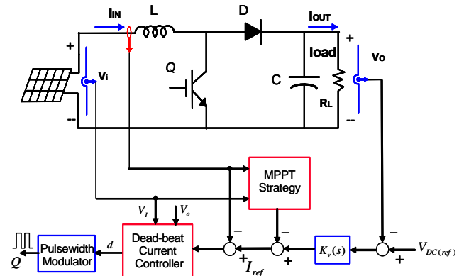
圖 2 升壓式直流轉換器電路暨控制方塊圖
