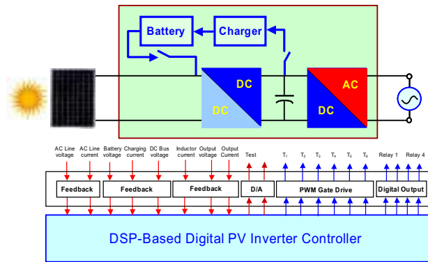
圖 23 太陽光變頻器 DSP 數位控制器的介面圖
