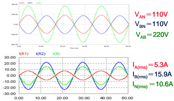
圖 8 不平衡負載輸出電壓模擬圖
