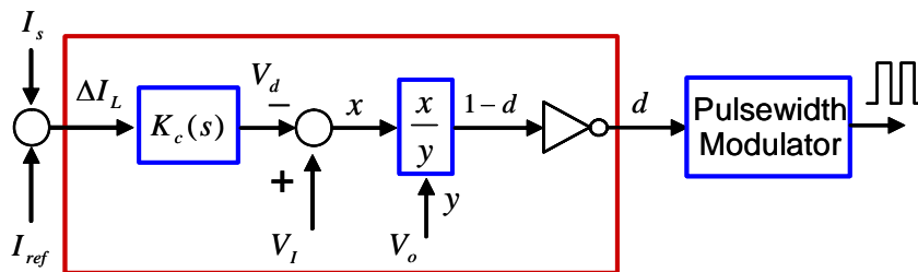
圖 7.2 前級之 Dead-beat 電流控制器
