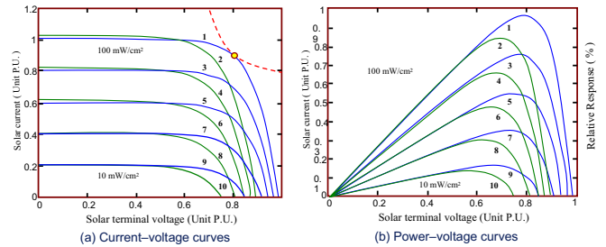
圖 6 典型的太陽光模組(I, V) 與(P, V)特性曲線
