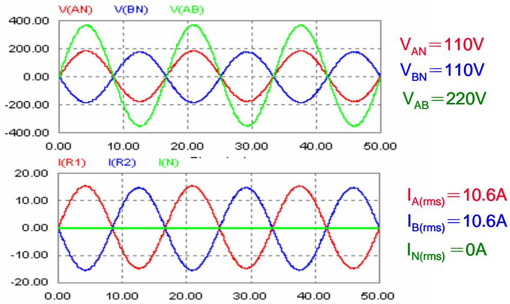
圖 7.6 平衡負載輸出電壓模擬圖
