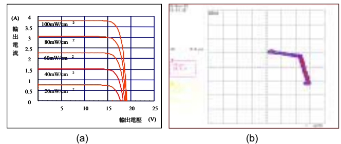
圖 9 太陽光模組模擬器 (a)特性曲線(b)實驗結果
