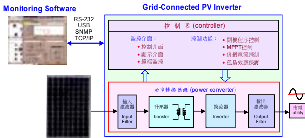
圖 22 併網型太陽光發電系統的系統架構圖
