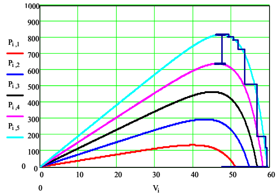
圖 19 併網型太陽光發電系統的 MPPT 控制模擬結果
