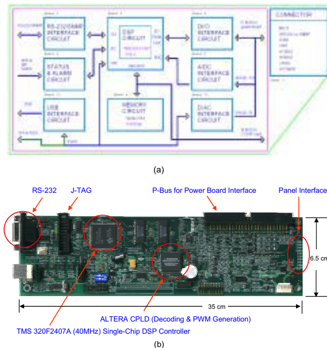
圖 24 PV inverter DSP 數位控制器 (a) 功能方塊圖 (b) 電路板
