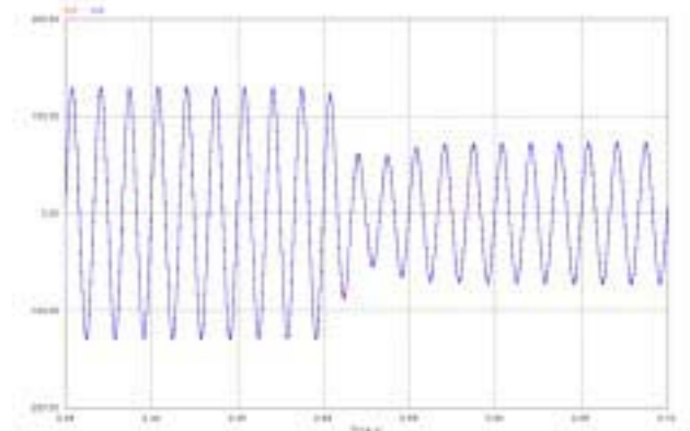
圖 20 併網模式瞬間輸出功率變化下的模擬結果
