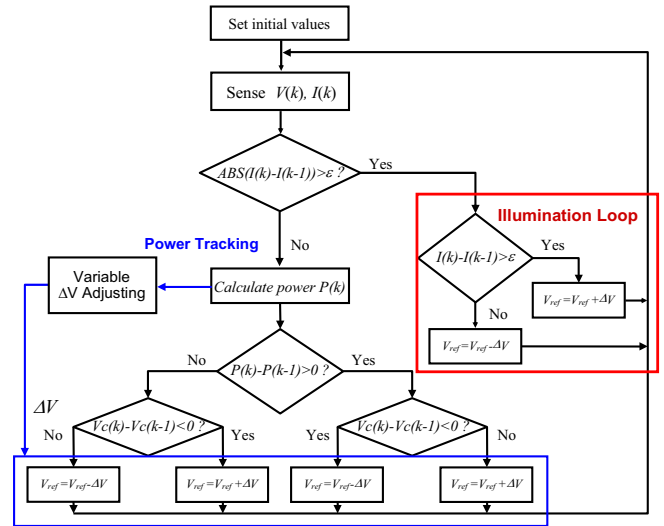
圖 12 最大功率操作點追蹤控制法則的程式流程圖
