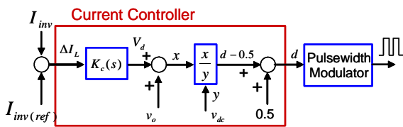
圖 5 變流器之 Dead-Beat 電流控制器
