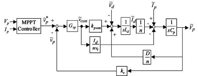
圖 14 輸出級變流器控制架構圖
