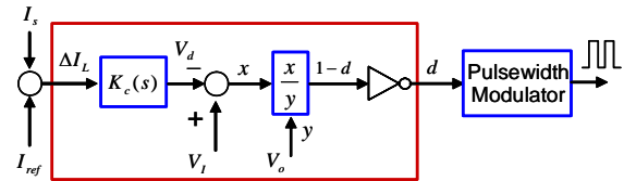
圖 3 前級之 Dead-beat 電流控制器
