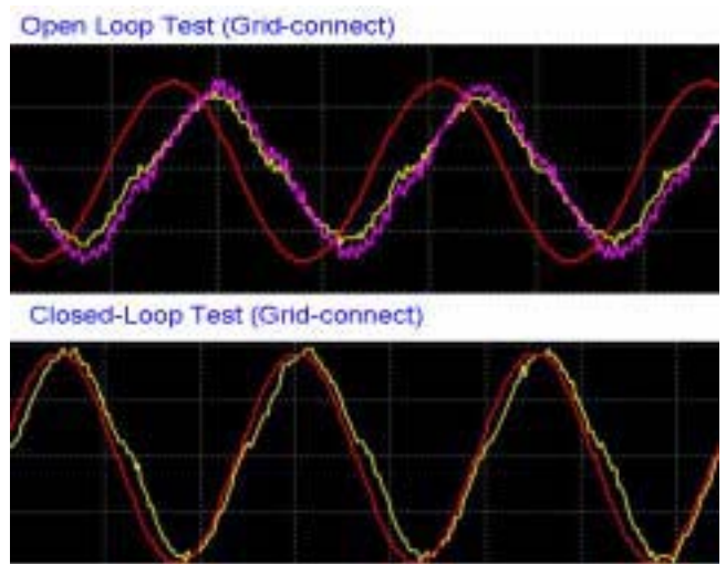
圖 26 併網模式輸出功率 2kW 的實驗結果
