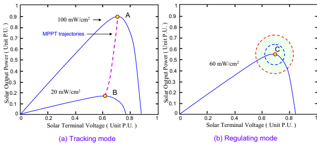
圖 10 MPPT 追蹤控制(a)追蹤模式(b)調節模式
