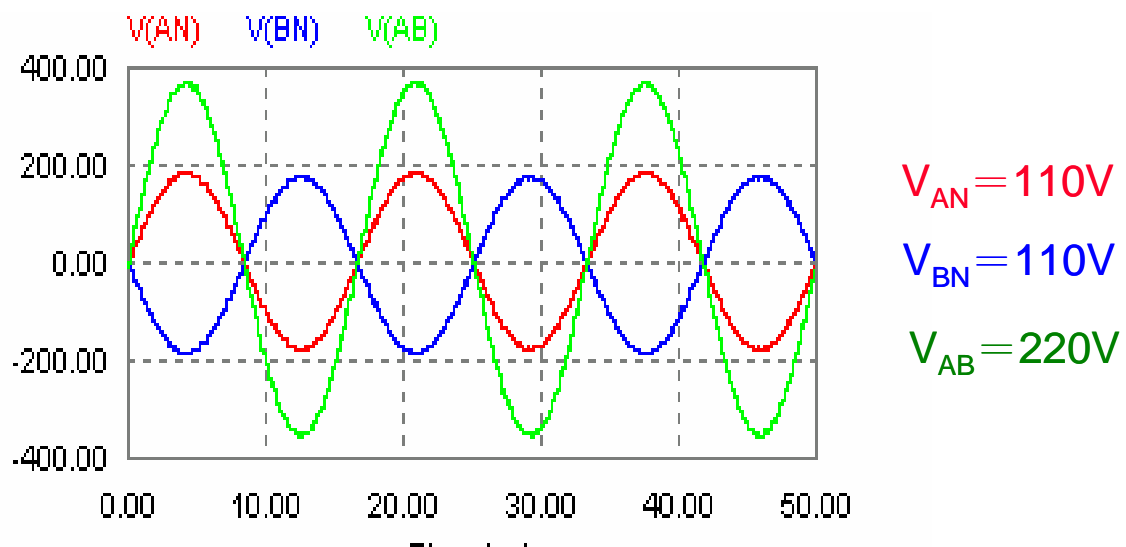
圖 7.5 單相三線制輸出電壓模擬圖
