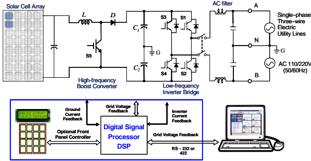
圖 1 功率級系統架構示意圖
