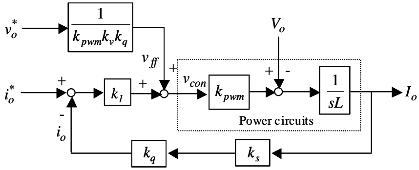
圖 6.3 電流迴路控制方塊圖
