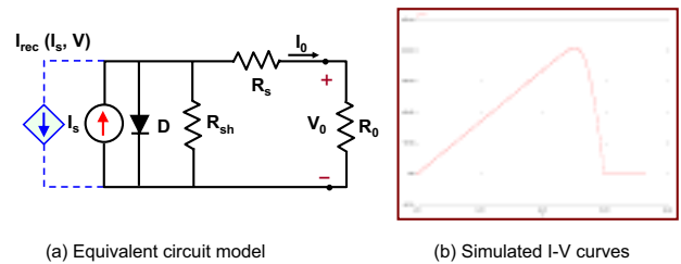
圖 7 太陽光模組的(a)等效電路圖與(b)模擬 IV 特性曲線
