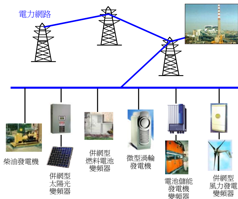
圖 2.10 併網型分散式電力供應系統
