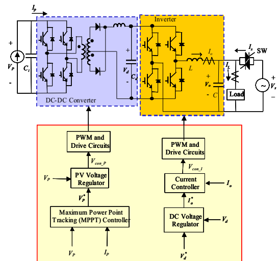
圖 16 數位式併網電流饋入控制的軟體架構圖
