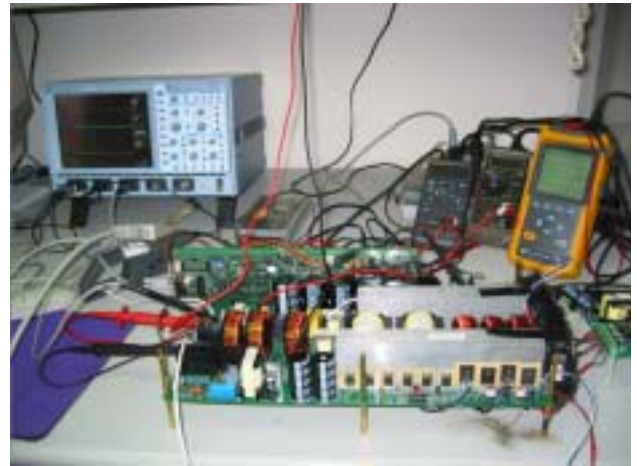
圖 25 研製完成的 DSP 控制併網型太陽光變頻器
