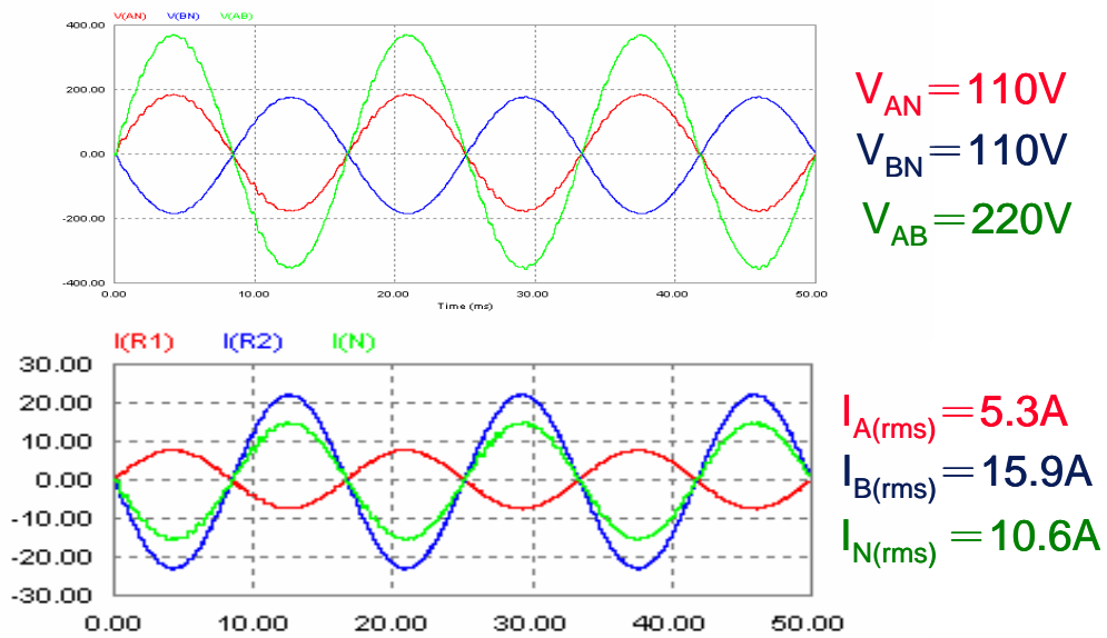
圖 7.7 不平衡負載輸出電壓模擬圖
