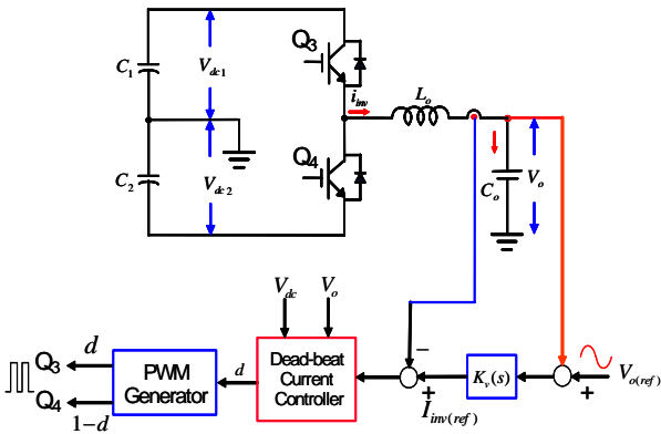
圖 4 變流器之控制方塊圖
