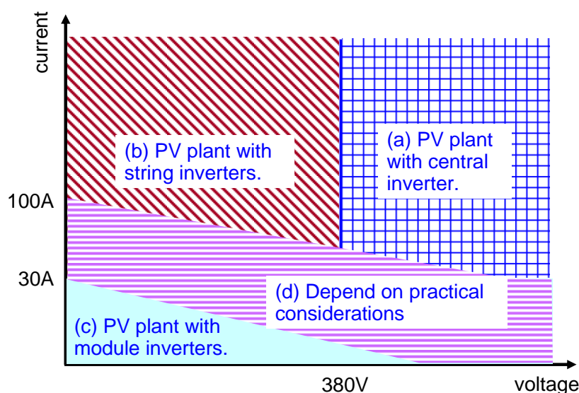
圖 2.4 併網型太陽光發電系統的系统架構選擇的考量
