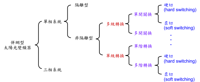
圖 1 併網型變頻器電路架構的分類
