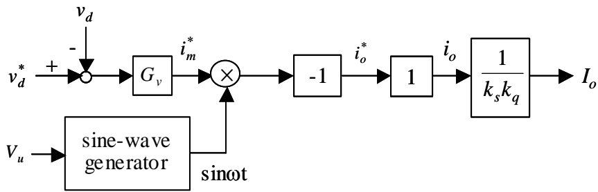
圖 6.4 直流電壓之控制方塊圖
