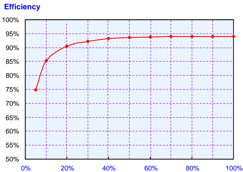
圖 8.9 併網太陽光變頻器的效率測試結果
