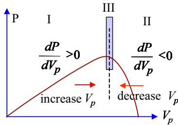
圖 11 最大功率操作點追蹤控制法則
