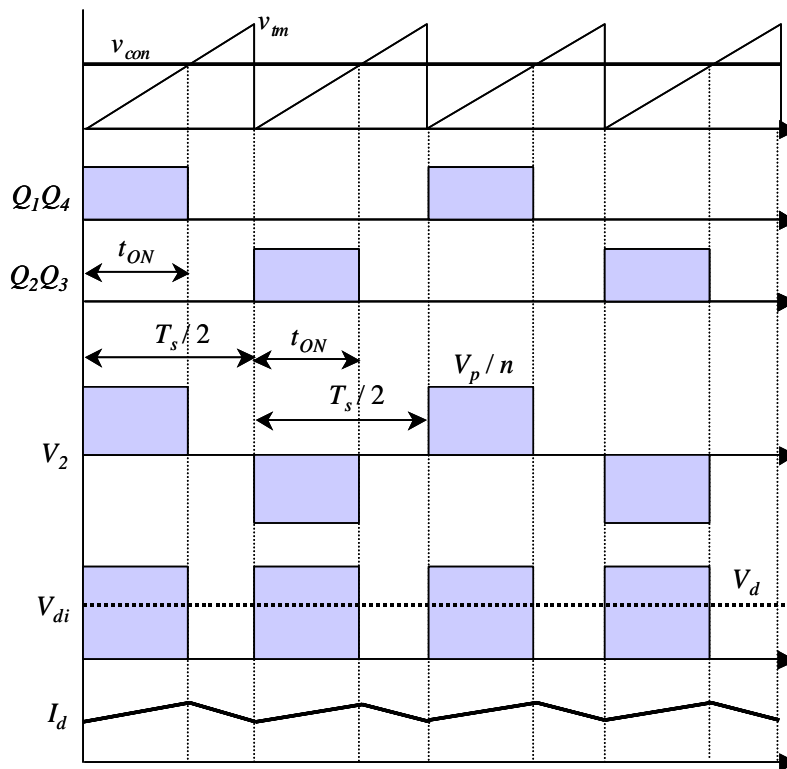
圖 4.2 採用 PWM 切換控制之全橋式 DC-DC 轉換器之工作波形
