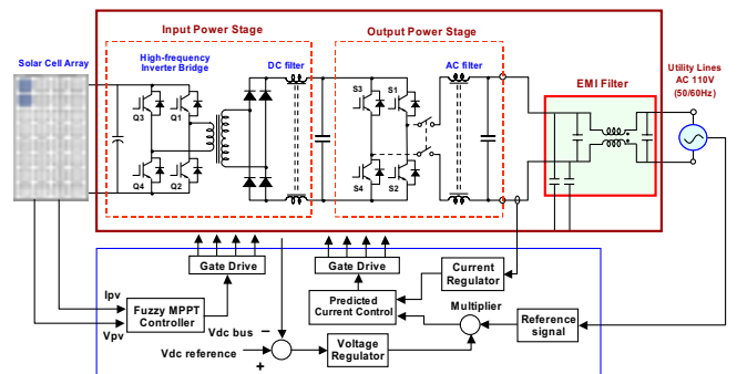
圖 13 雙級式併網型太陽光發電系統的控制方塊圖
