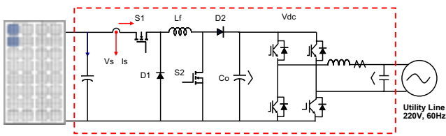
圖 4 非隔離式雙級併網型變頻器
