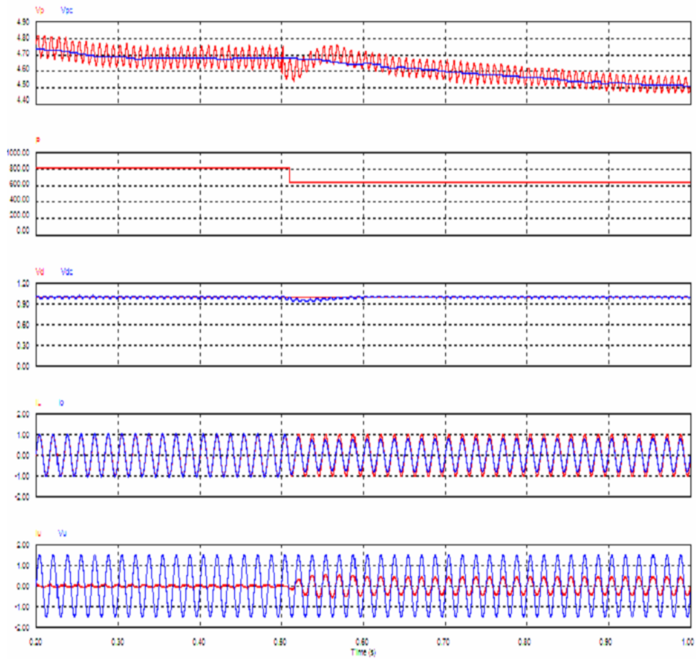
圖 6.14 一完整系統之模擬結果
