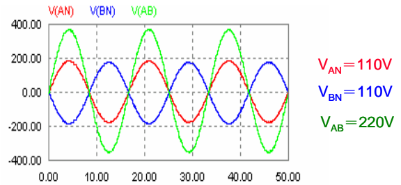
圖 6 單相三線制輸出電壓模擬圖
