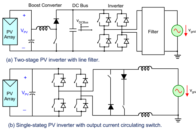
圖 3 非隔離式併網型變頻器的基本電路架構
