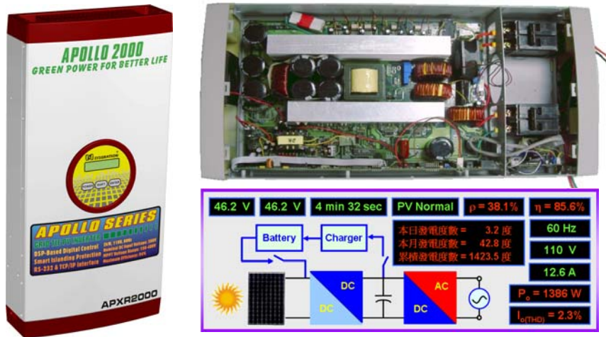
圖 8.8 研製完成的併網型太陽光變頻器原型
