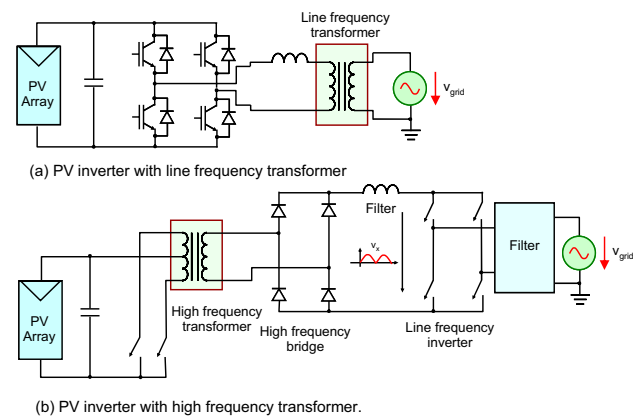
圖 2 隔離式併網型變頻器的基本電路架構
