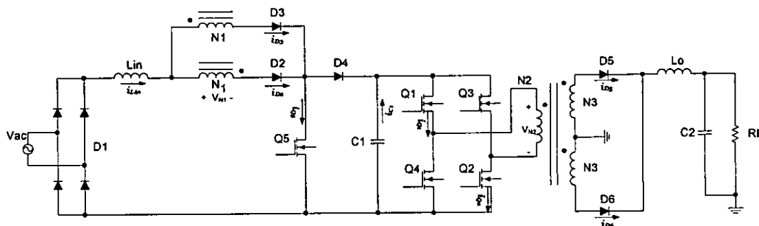
圖 2-4 單級全橋式交/直流轉換器
