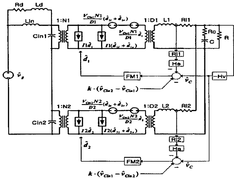
圖 3-5 ISOP 的小訊號模型
