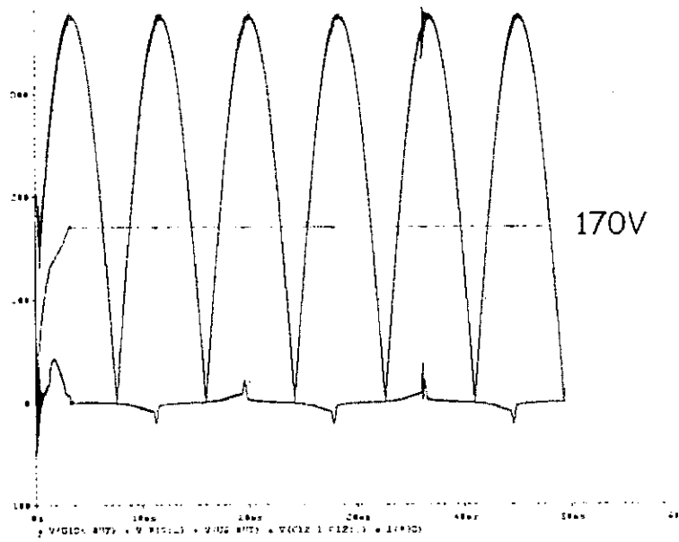
圖 3-20 輸出電壓 170V，負載 30.05 歐姆，輸出功率 961W
