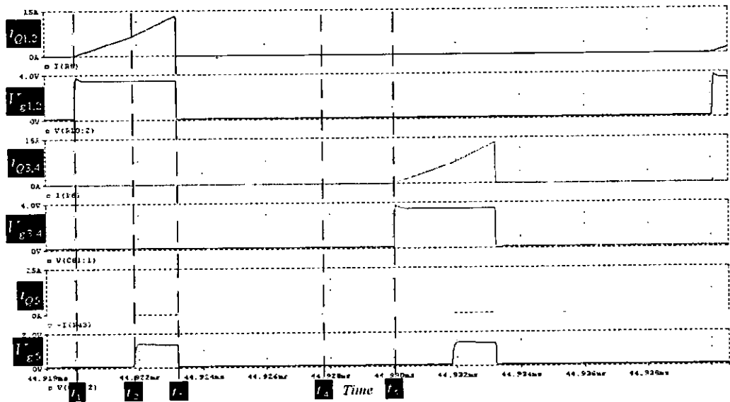
圖 2-12 5 個模式時間內開關電流 i_{Q1} 、 i_{Q2} 和 i_{Q5} 並配合 Q_1 \sim Q_5 開極控制信號
