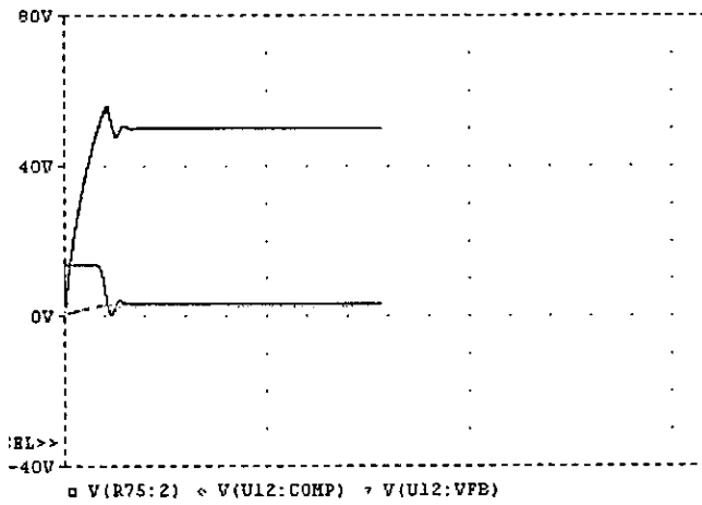
圖 3-13 沒有加上光耦合器的單級全橋輸出電壓波形
