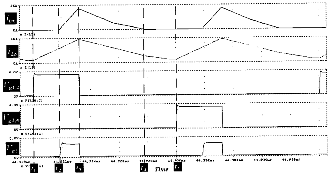
圖 2-13 5 個模式時間內的輸入電感電流和輸出電感電流並配合 Q_1 \sim Q_5 開極控制信號
