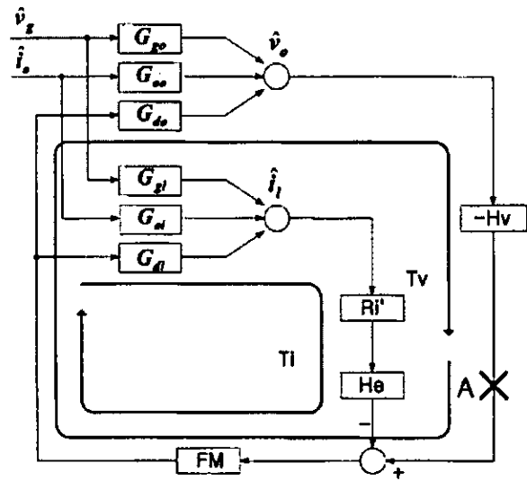
圖 3-4 圖 3-3 的簡化方塊圖
