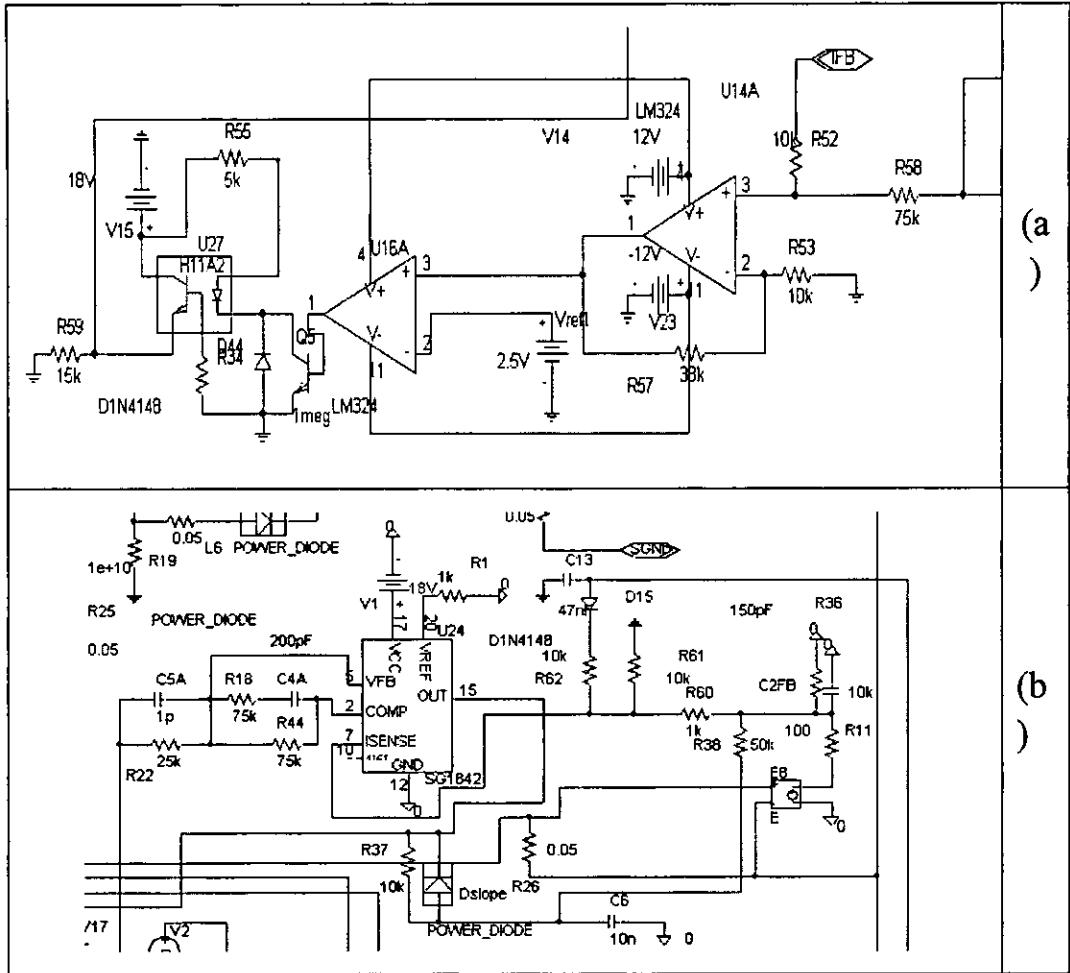
圖 3-24 (a)UC3842 周邊電路
