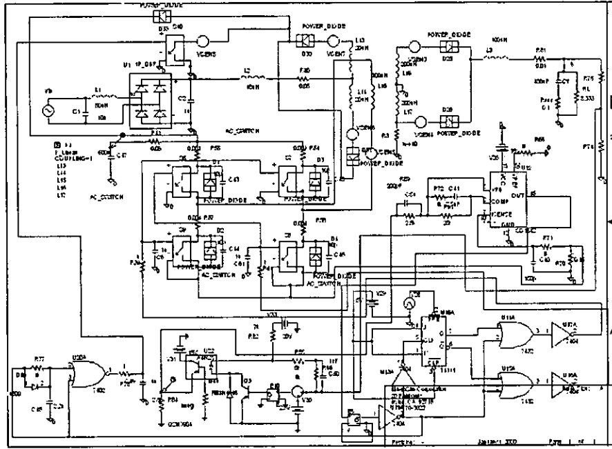
圖 3-12 單級全橋加上光耦合器的電路
