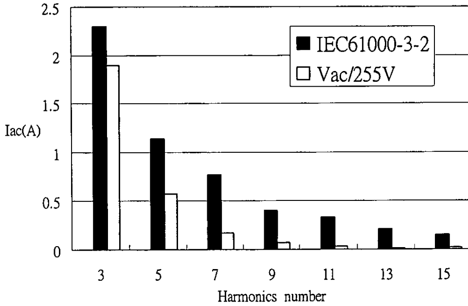
圖 2-20 工作於 1000W 且 255Vac 輸入時的輸入諧波電流與 IEC61000-3-2 A 類標準的比較圖
