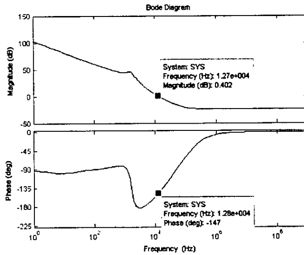
圖 3-7 單模組 BIFRED 的 T_v(s) 之波德圖
