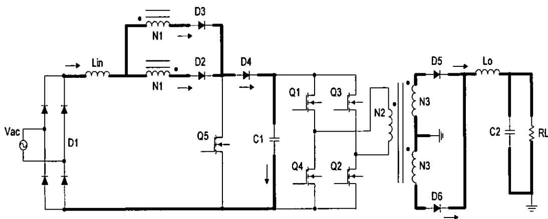
圖 2-8 t_3 \leq t < t_4 的電流迴路
