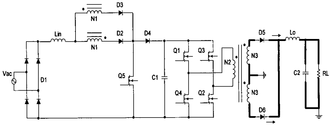
圖 2-9 t_4 \leq t < t_5 的電流迴路
