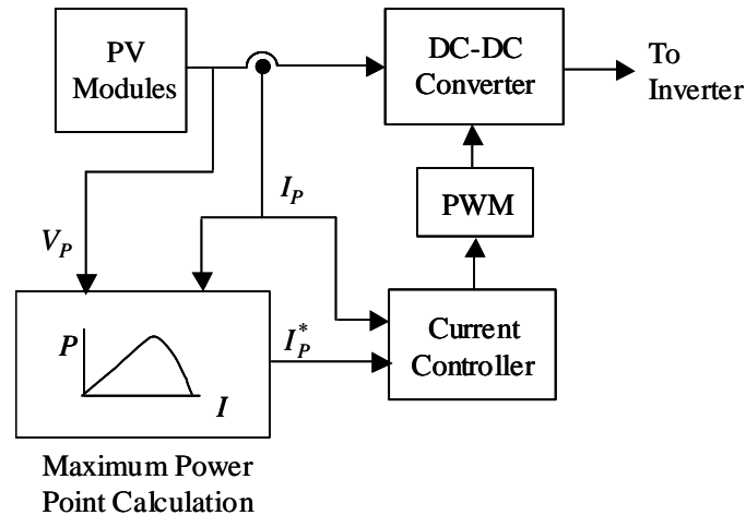
圖 4.9 利用電流模式控制 DC-DC 轉換器來實現 MPPT 之方法
