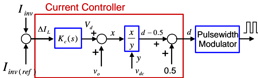
圖 6.4 變流器之預測型電流控制器
