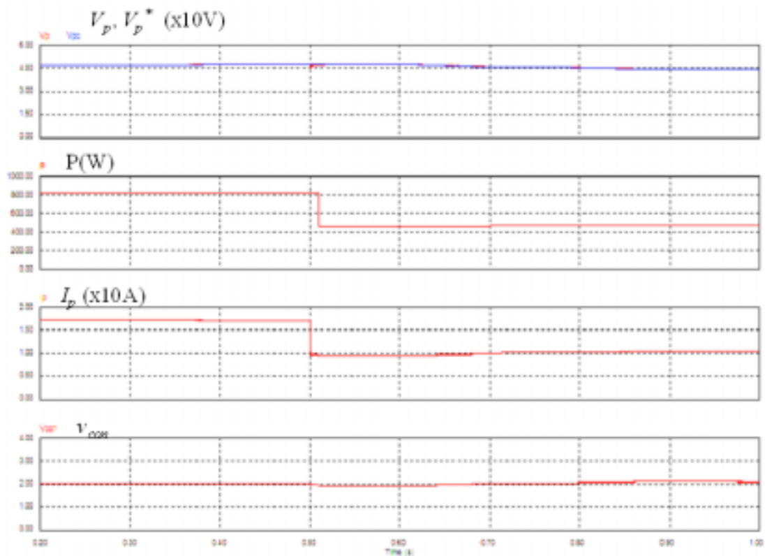
圖 4.14 日照量由 1\text{KW}/\text{m}^2 變化為 0.6\text{KW}/\text{m}^2 下 MPPT 控制之模擬結果
