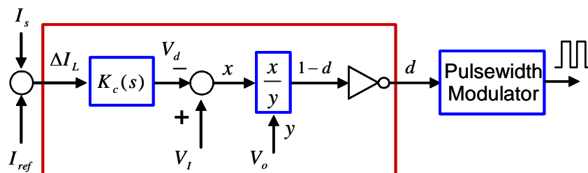
圖 6.2 前級之 Dead-beat 電流控制器
