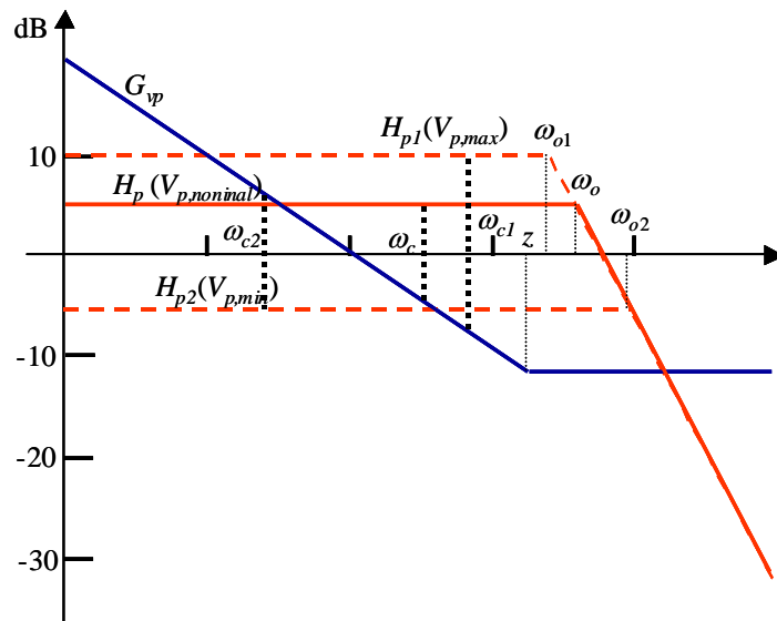
圖 4.4 H_p(s) 之波德圖以及 PI 控制器之設計
