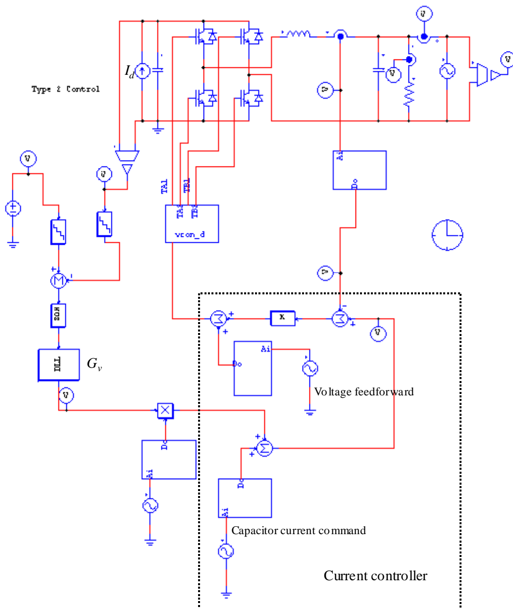
圖 5.7 PSIM 之變流器模擬電路
