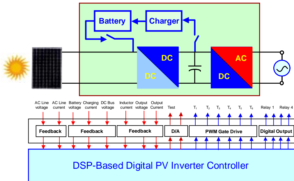
圖 7.2 太陽光變頻器 DSP 數位控制器的系統架構
