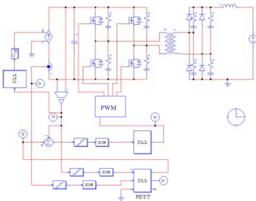
圖 4.13 包含 MPPT 及 DC-DC 轉換器之 PSIM 模擬程式
