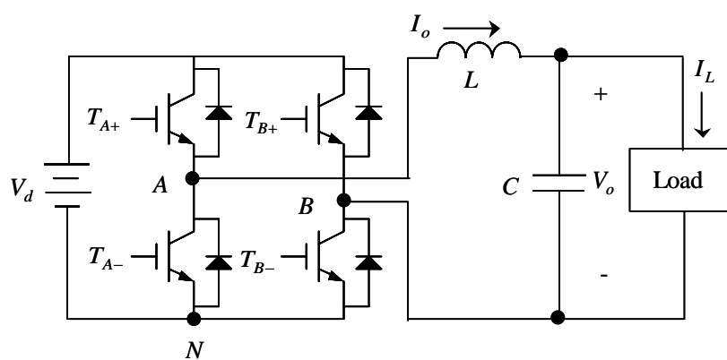
圖 5.1 全橋式電壓源變流器
