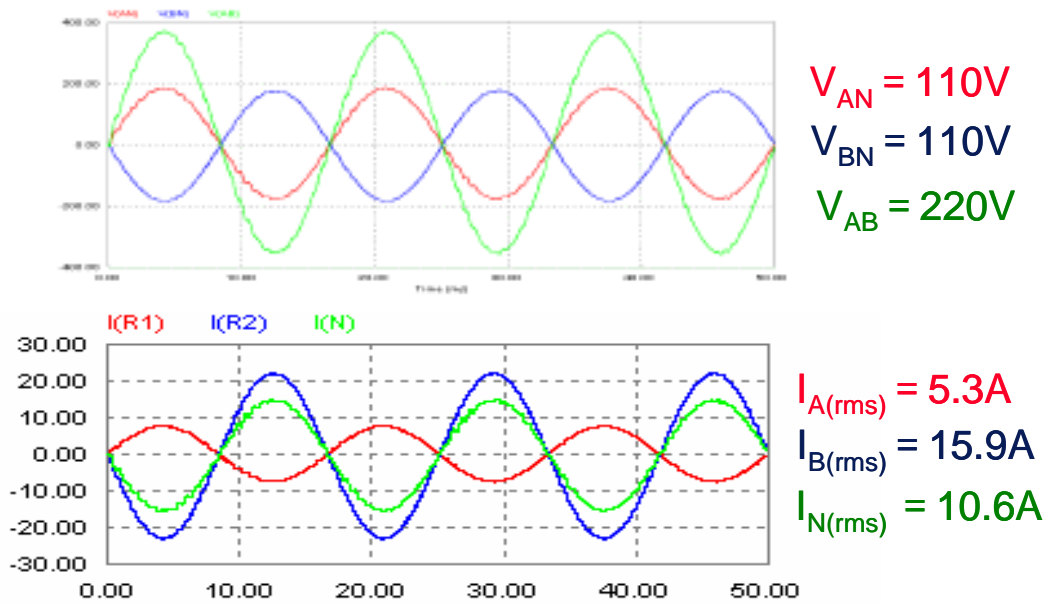
圖 6.7 不平衡負載輸出電壓模擬圖
