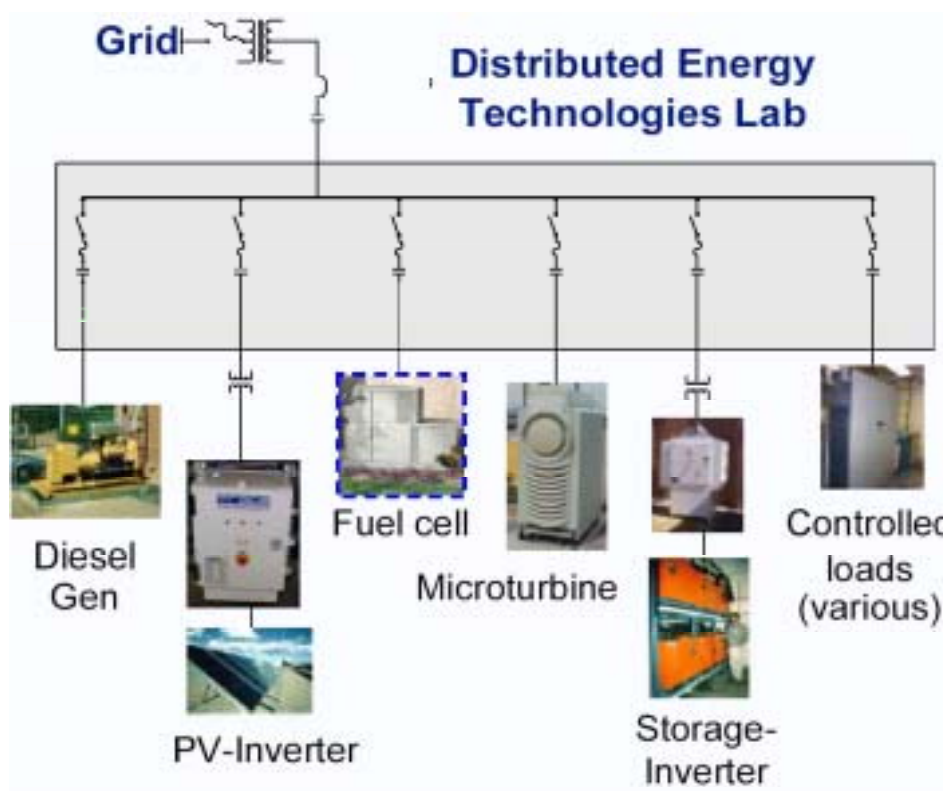
圖 2.6 併網型分散式電力供應系統
