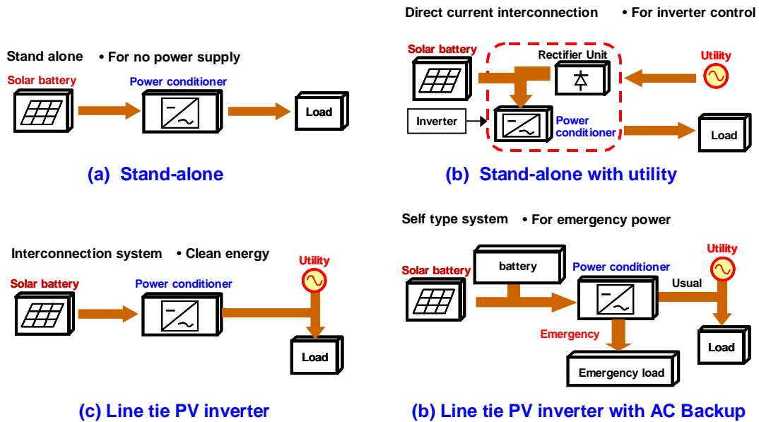
圖 2.1 不同型式太陽光變頻器的系統架構圖
