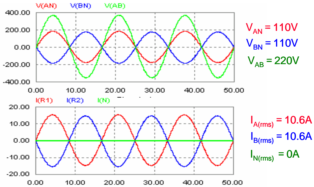
圖 6.6 平衡負載輸出電壓模擬圖
