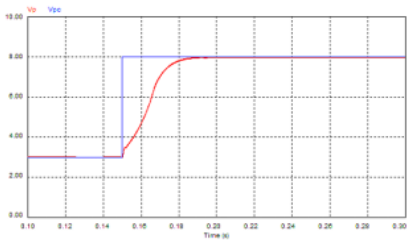
圖 4.12 模擬之輸入電壓波形及其命令
