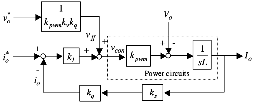
圖 5.3 電流迴路控制方塊圖
