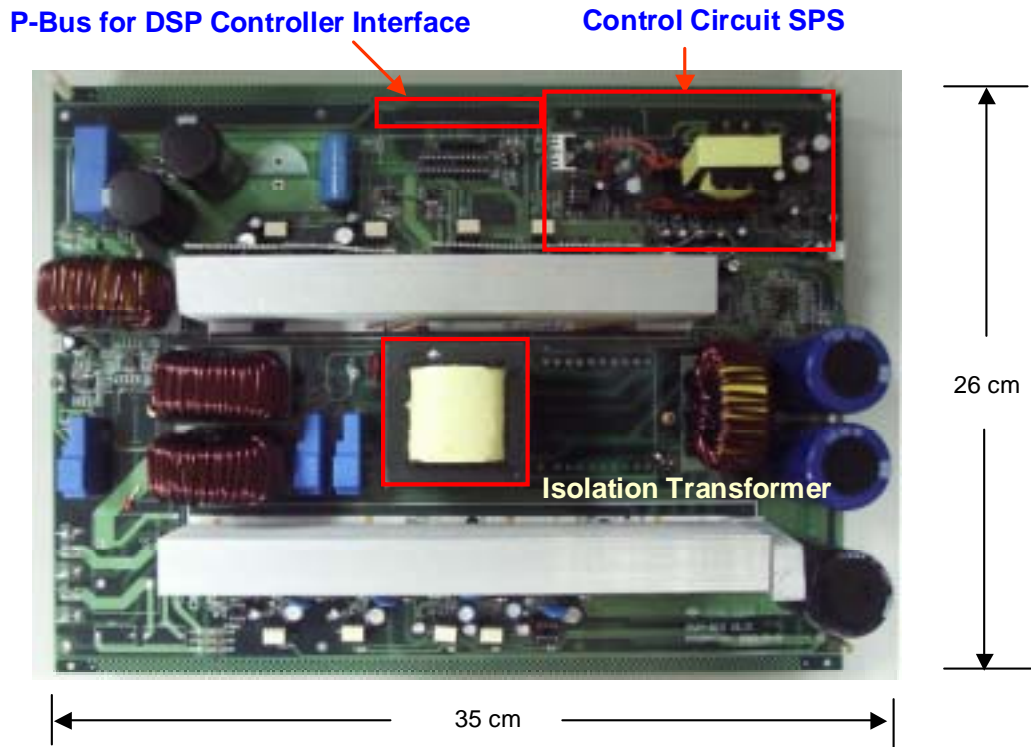
圖 7.5 研製完成的 2kVA PV-Inverter 功率電路板
