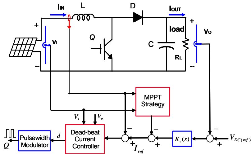
圖 6.1 升壓式直流轉換器電路暨控制方塊圖
