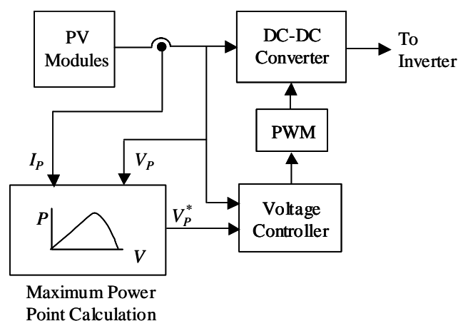
圖 4.8 利用電壓模式控制 DC-DC 轉換器來實現 MPPT 之方法
