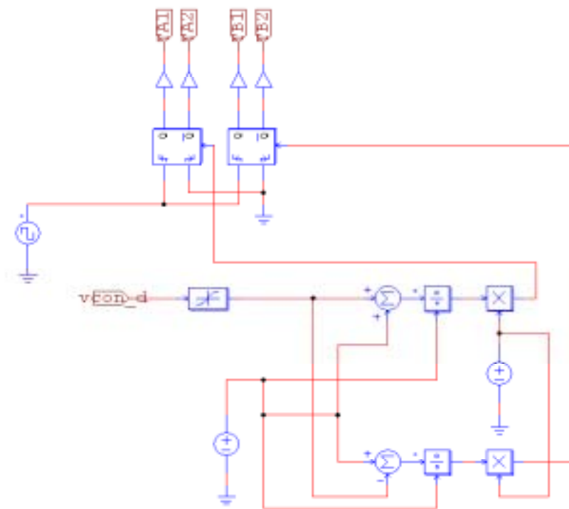
圖 5.9 單電壓極性切換 PWM 電路之建立
