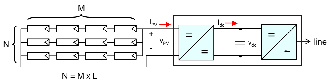
圖 2.5 太陽光模組的排列組合圖
