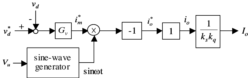
圖 5.4 直流電壓之控制方塊圖
