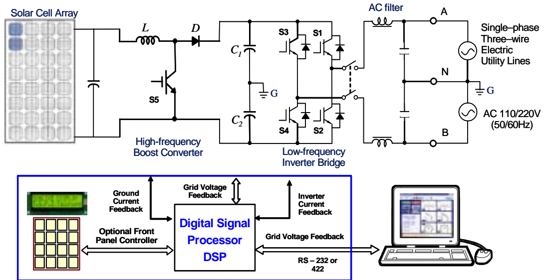
圖 2.4 三線單相式併網型太陽光變頻器的電路架構圖
