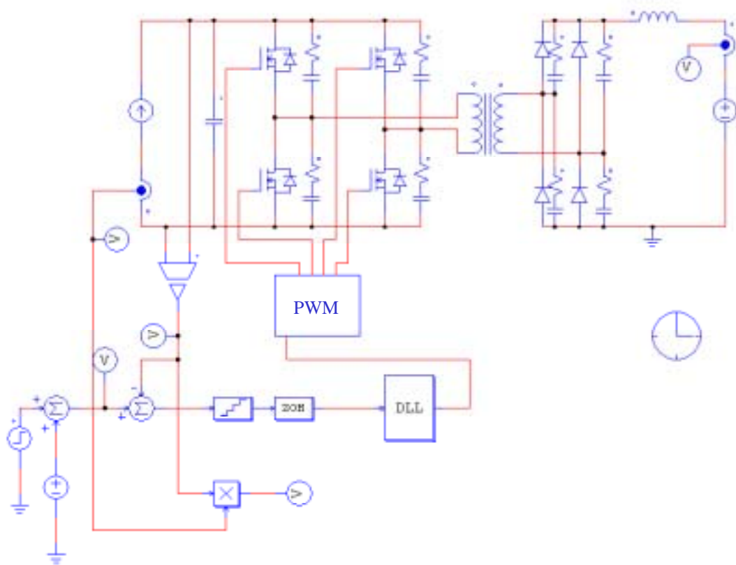
圖 4.11 驗證 DC-DC 轉換器之 PSIM 模擬電路
