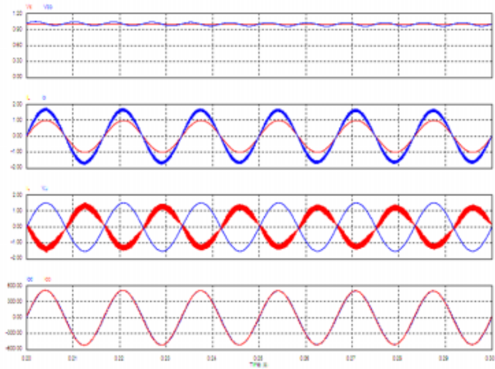
圖 5.12 負載電力小於太陽能所發電力之模擬結果
