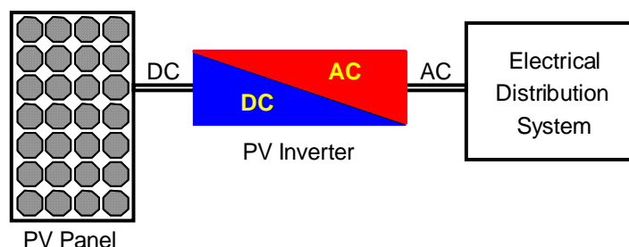
圖 2.2 併網型太陽光變頻器的系統方塊圖
