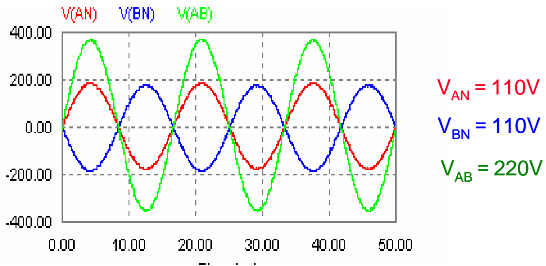
圖 6.5 單相三線制輸出電壓模擬圖
