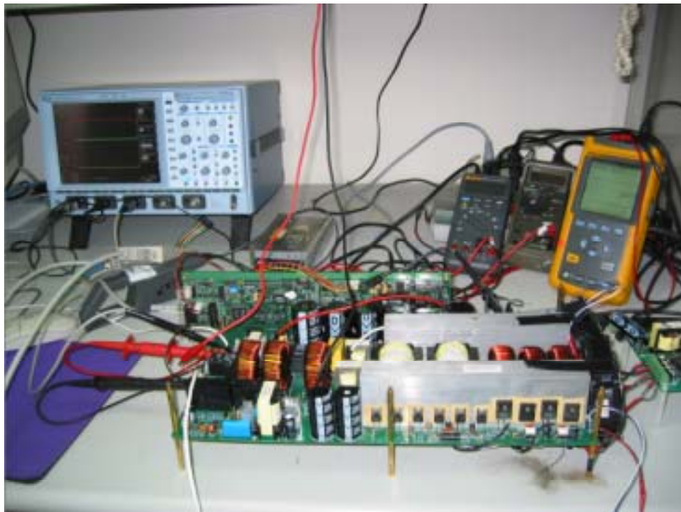
圖 7.6 整合測試中的 DSP 控制併網型太陽光變頻器
