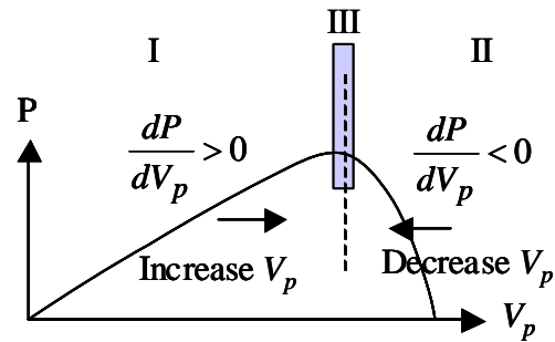
圖 4.10 所提之最大功率點追蹤控制方法
