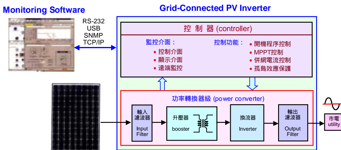
圖 3.1 併網型太陽光發電系統的系統架構圖
