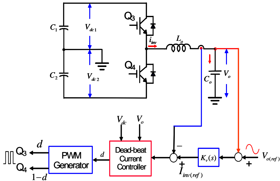
圖 6.3 變流器之控制方塊圖
