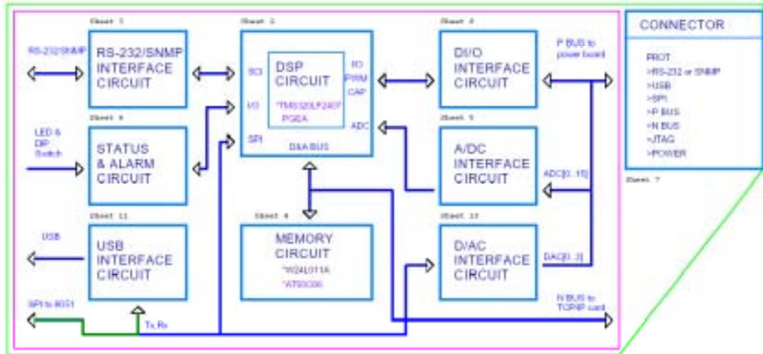
圖 7.3 DSP 數位控制器的功能方塊圖
