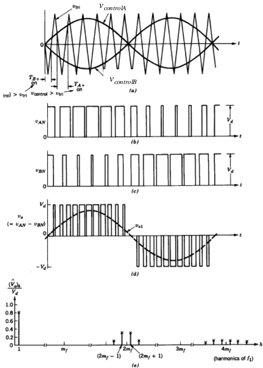
圖 5.2 Uni-polar 正弦式 PWM
