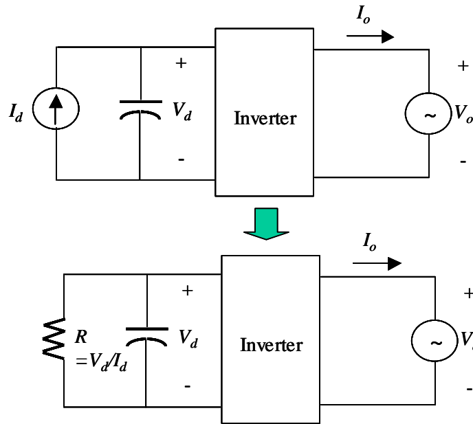
圖 5.5 變流器直流側可視為一等效電阻為 R(=V_d/I_d) 之直流負載
