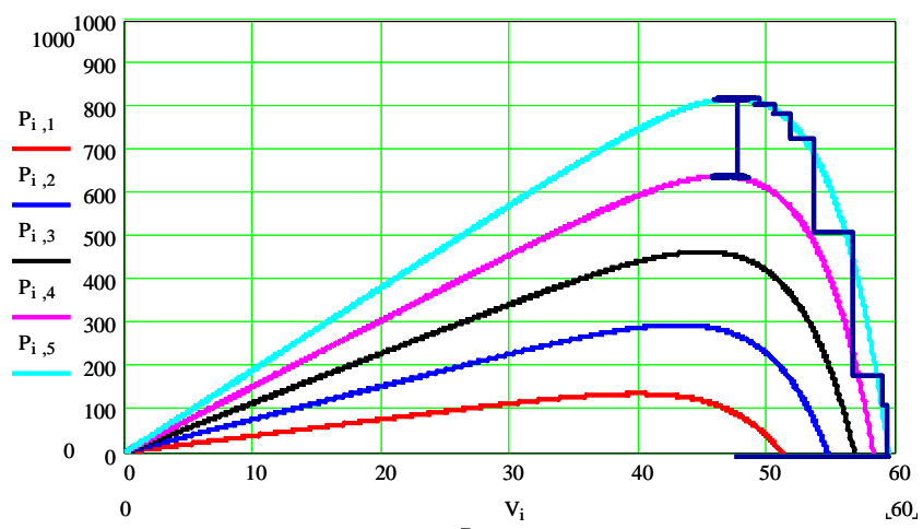
圖 5.15 最大功率點追蹤之模擬結果
