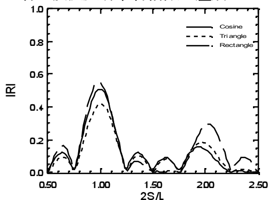
圖 2 不同人工沙洲形狀上之波浪反射率 ( d=15\text{cm} , D=5\text{cm} , B=50\text{cm} , S=80\text{cm} , N=4 )
