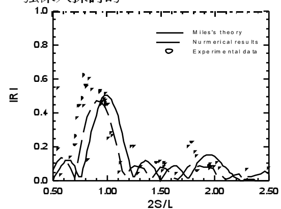
圖 1 正弦型人工沙洲上波浪反射率之理論解、數值解及實驗值之比較 ( d=15\text{cm} , D=5\text{cm} , B=50\text{cm} , S=80\text{cm} , N=4 )
